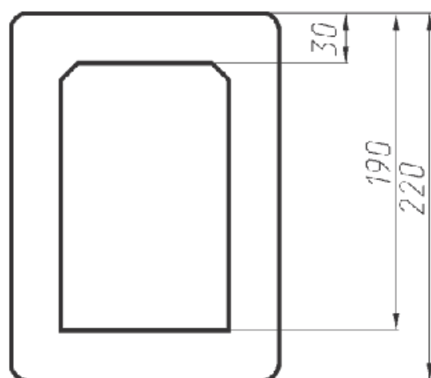
Базовые размеры
