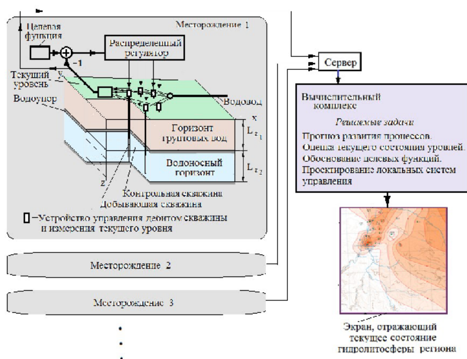
Рис.1.1. Сеть мониторинга и управления гидrolитосферными процессами региона .
