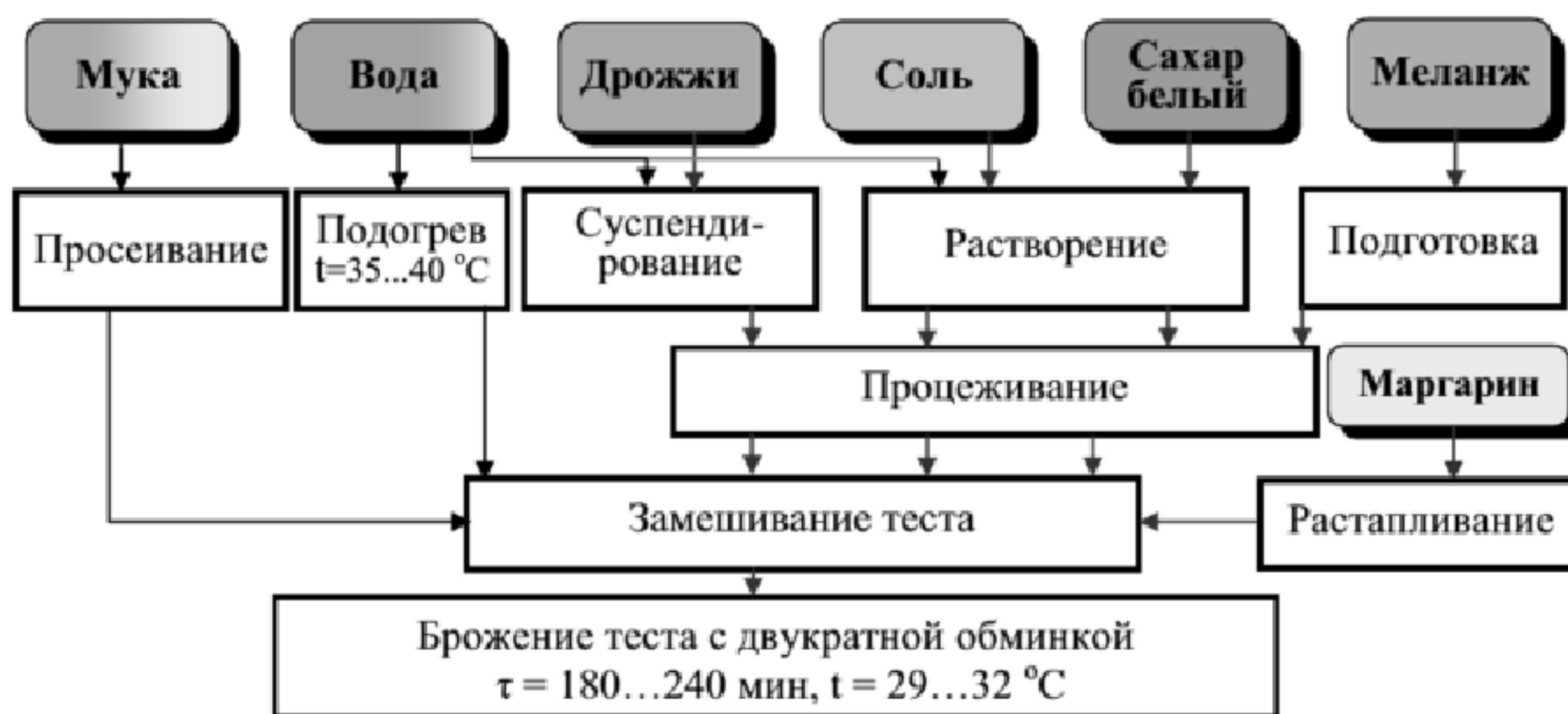
Технологическая схема дрожжевого теста безопарного
