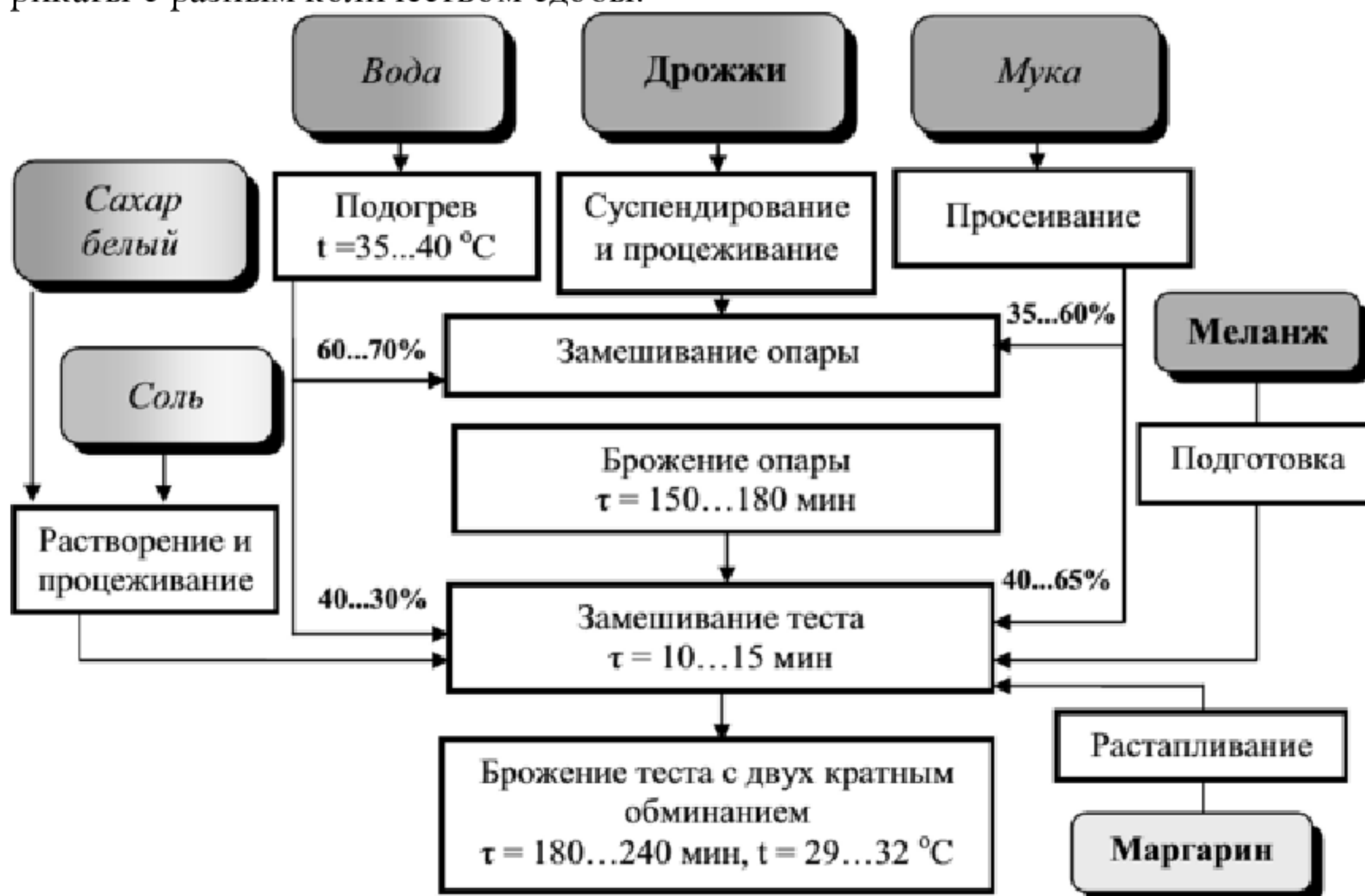
Технологическая схема опарного дрожжевого теста
