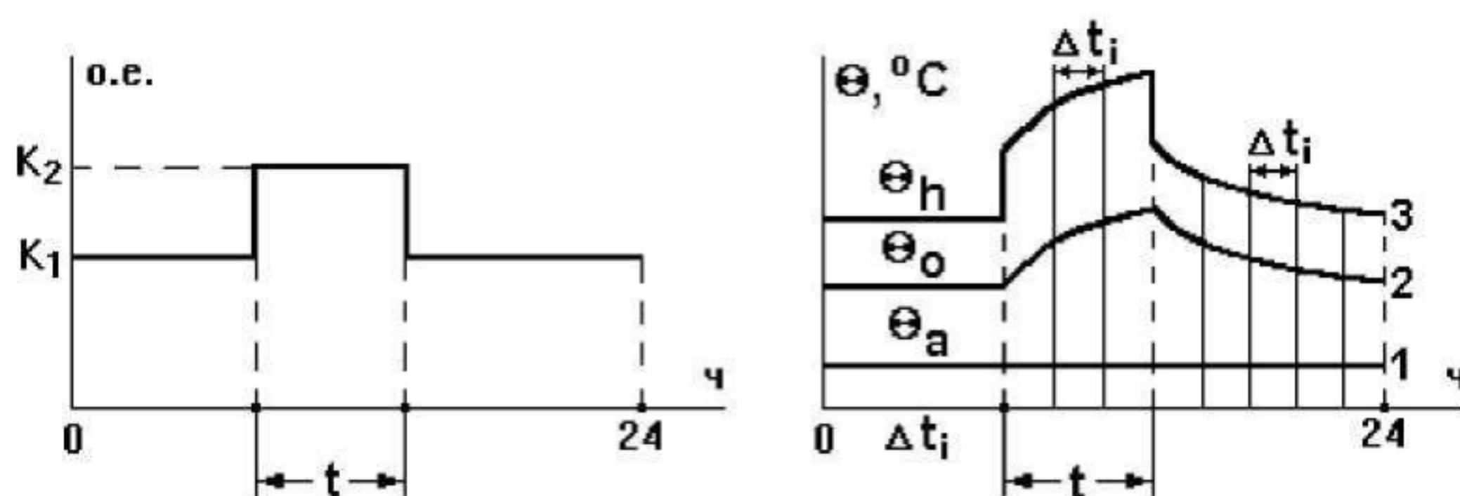
Рисунок 3.1 - Двухступенчатый суточный график нагрузки (а) и переходный тепловой режим в трансформаторе (б)
