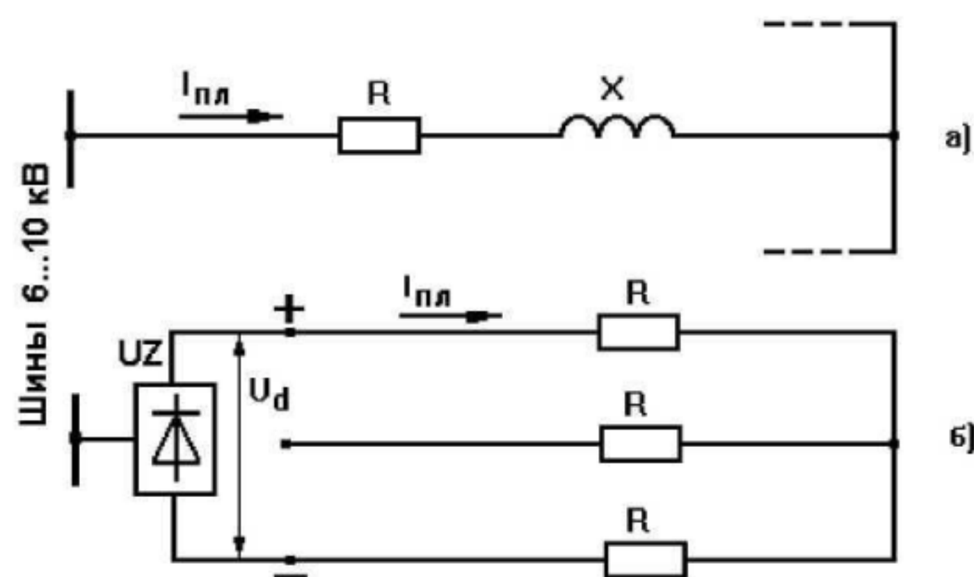
Рисунок 1.1 - Принципиальные схемы плавки гололеда переменным (а) и постоянным (б) током
