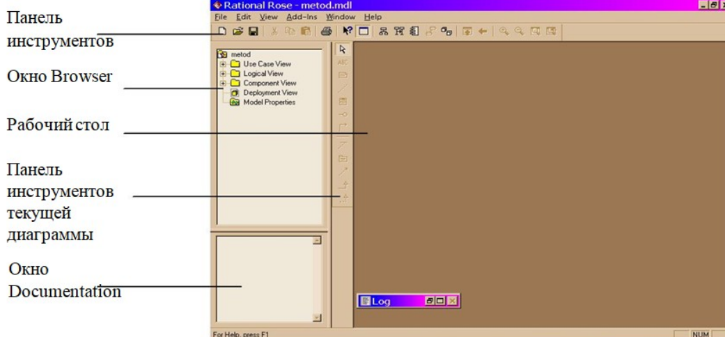
Рис.5 - Главное окно Rational Rose2000
