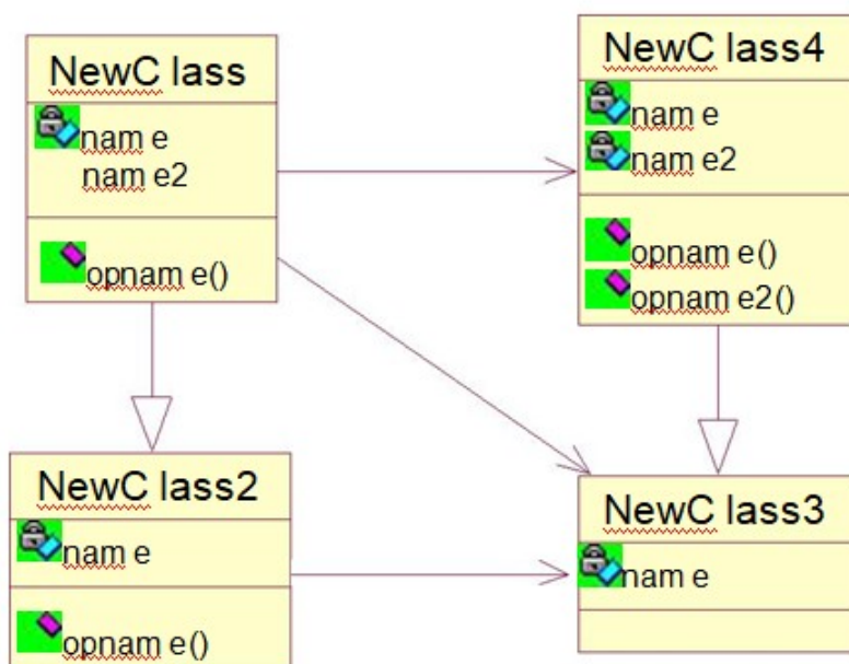
Рис.1 Диаграмма классов
