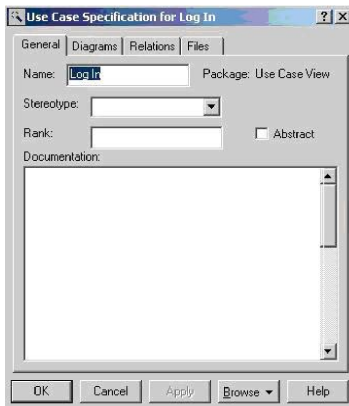
Рис. 2. Окно спецификаций
