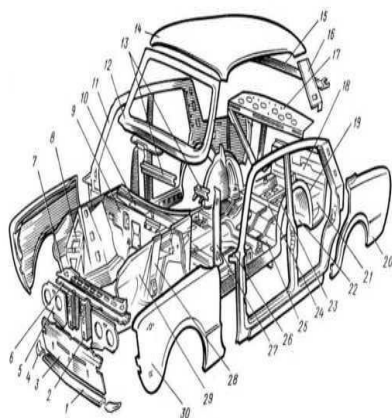
Рис. 1.3. Элементы основы кузова
