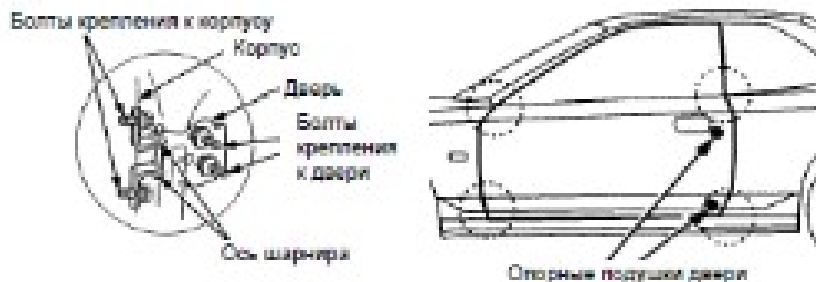
Рис. 5.4. Крепление шарнира Рис. 5.5. Опорные подушки
