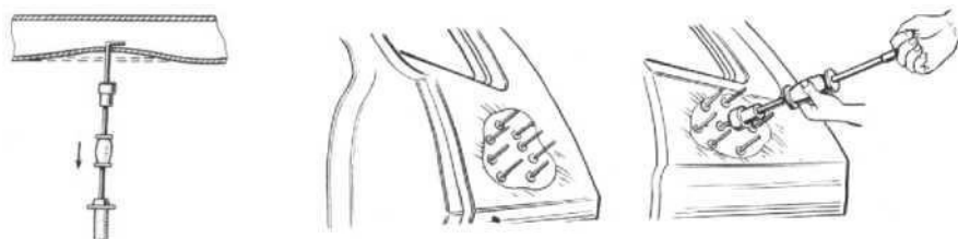
Рис. 6.3. Применение инерционного молотка
