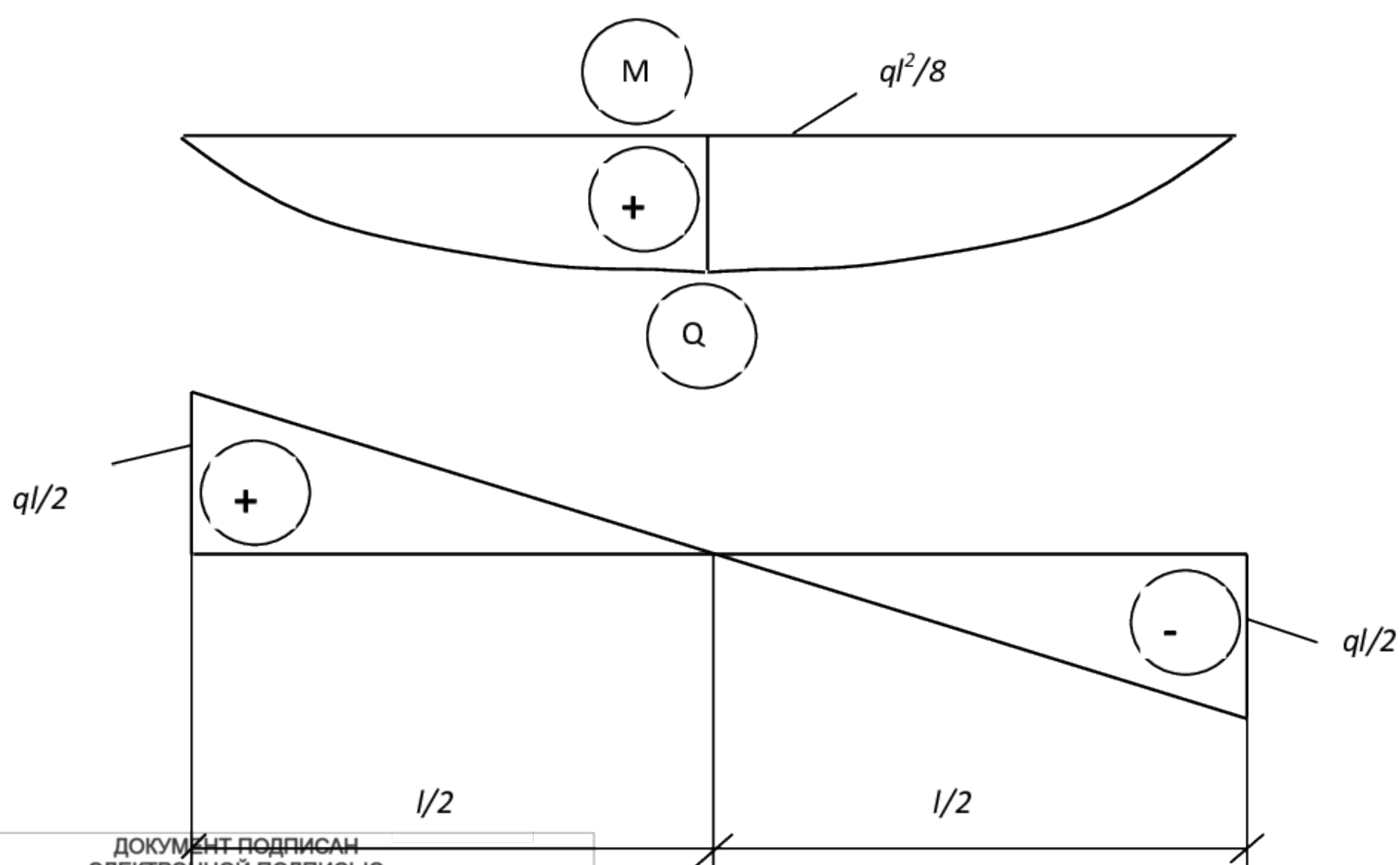
Рисунок 2 – Расчетная схема плиты и эпюры расчетных усилий (изгибающих моментов M и поперечных сил Q )
