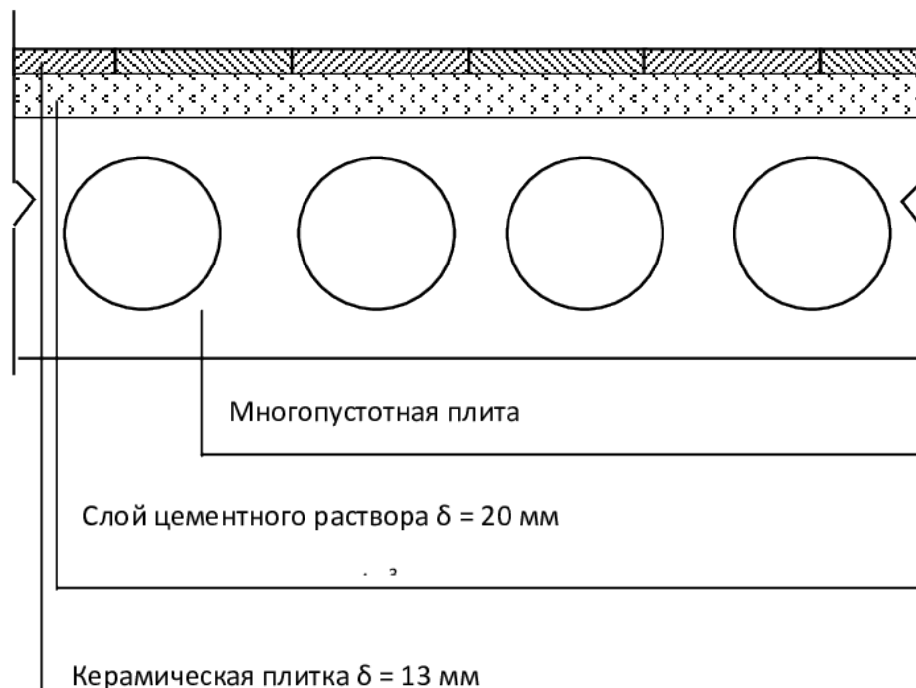
Рисунок 2 - Разрез конструкции пола
