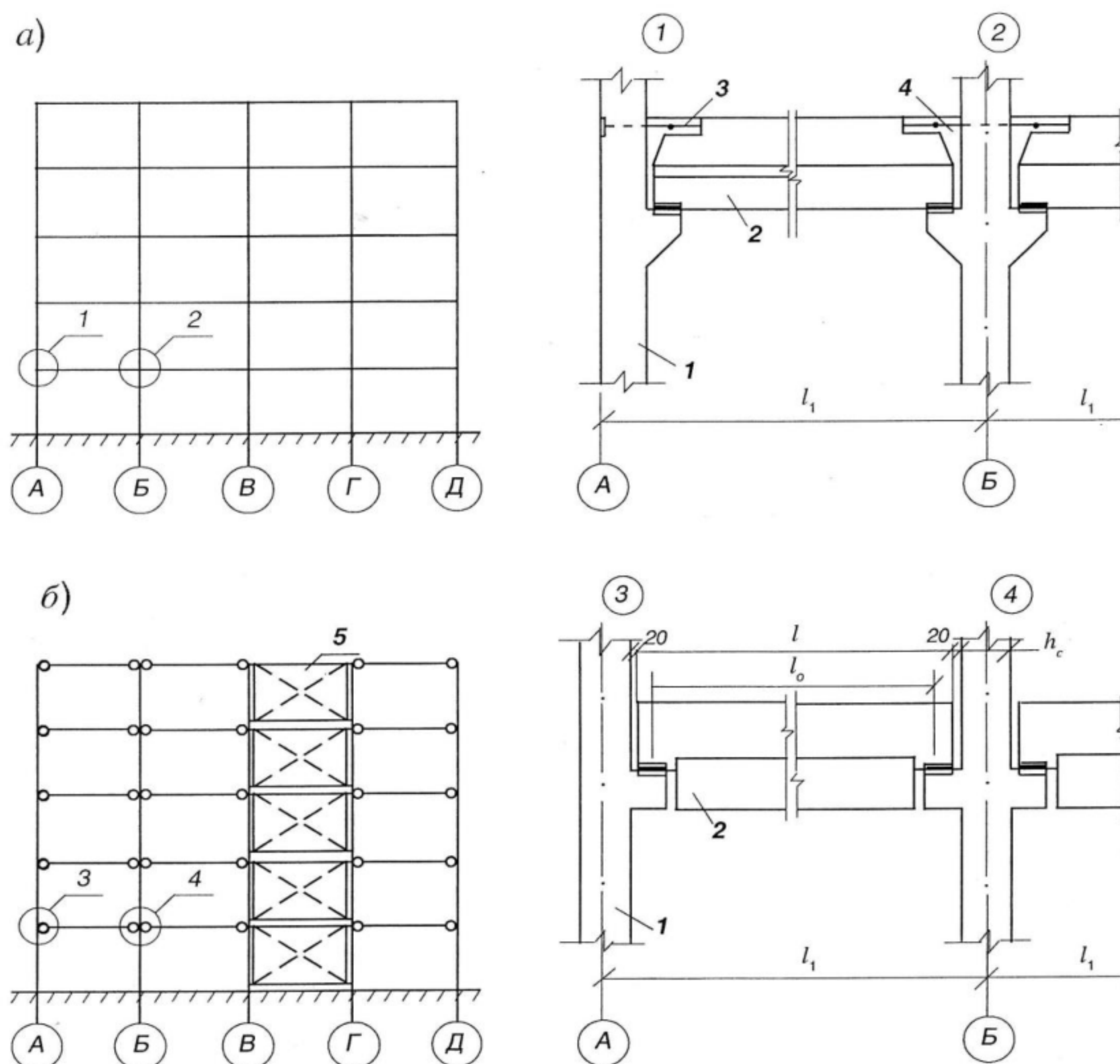
Рисунок 1 – Схемы рамного (а) и связевого (б) каркаса
