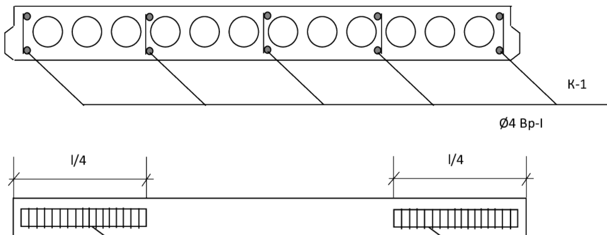
Рисунок 6 - Размещение поперечной конструктивной арматуры в поперечном и продольном сечениях плиты (К-1 – сварные каркасы)
