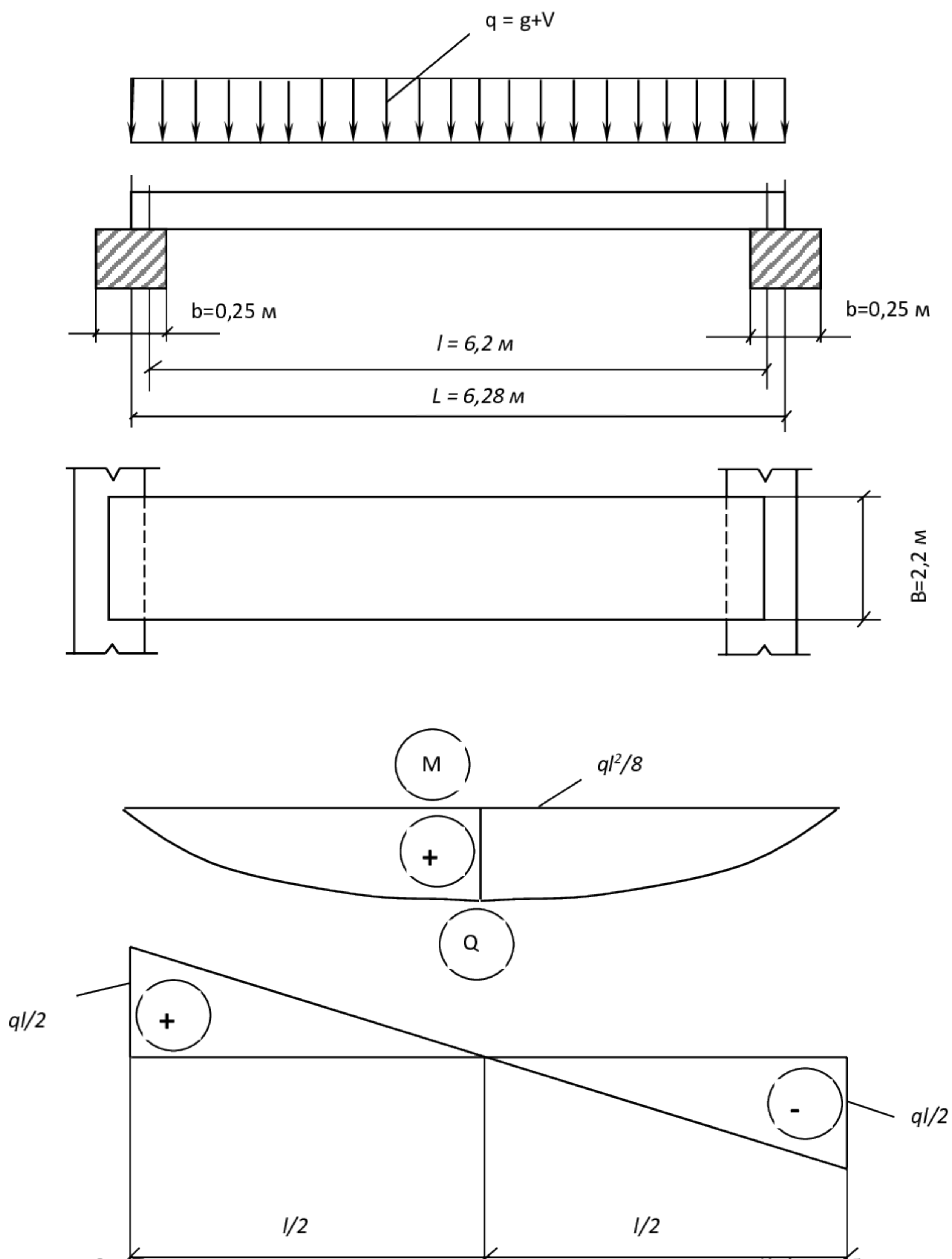
Рисунок 2 - Расчетная схема плиты и эпюры расчетных усилий (изгибающих моментов M и поперечных сил Q )
