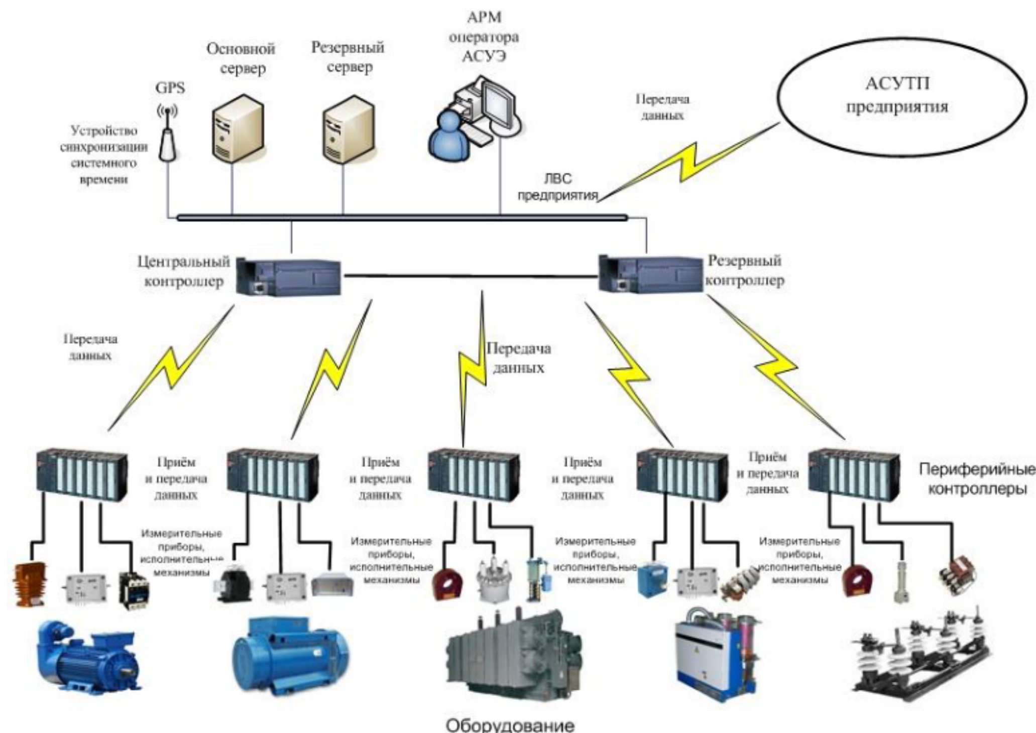
Рисунок 3 - АСУ ТП предприятия
