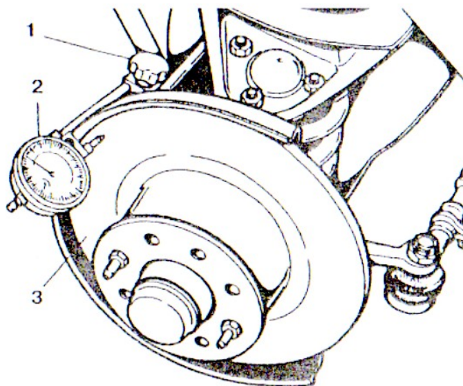
Рис. 3. Проверка осевого биения тормозного диска: 1 – магнитная подставка; 2 – индикатор; 3 – тормозной диск.
