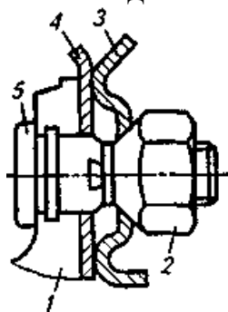
Рис. 9 Крепление колеса легкового автомобиля: 1 — ступица; 2 — гайка; 3 — диск колеса; 4 — тормозной барабан; 5 — болт
