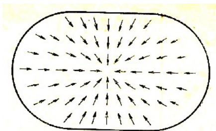
Рис. 13 Направление касатель- ных сил в плоскости контакта шины
