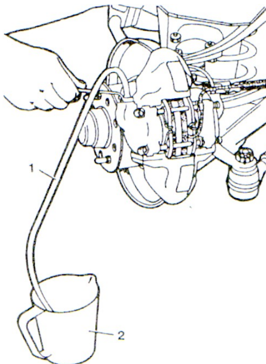
Рис. 2. Удаление воздуха из трубопроводов системы гидравлического привода тормозов левого переднего колеса: 1 – шланг для подкачки; 2 – ёмкость для тормозной жидкости.
