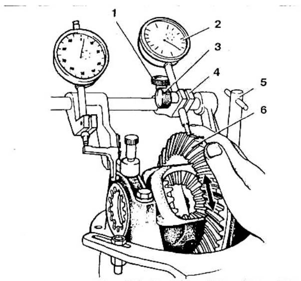
Рис. 9. Проверка бокового зазора в зацеплении шестерен главной передачи приспособлением А.95688/R:
