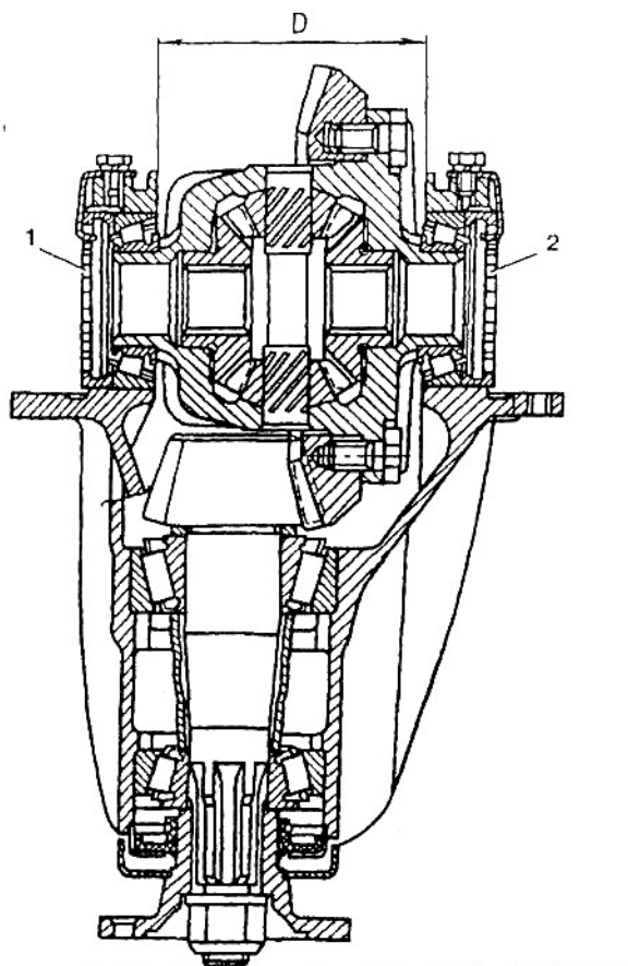
Рис. 10. Схема проверки предварительного натяга подшипников коробки дифференциала:
