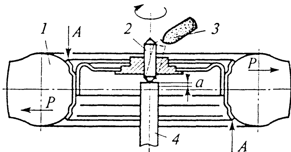
Рис. 1. Схема динамической балансировки колеса:
