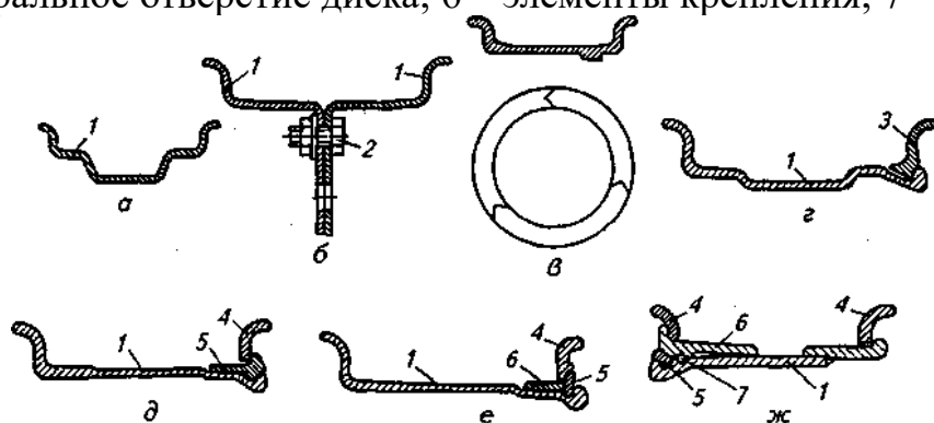
Рис. 8 Основные типы ободьев колес: а — неразъемный глубокий симметричный; б — разъемный посередине; в — сегментный типа «триллекс», разделенный по радиусу на три сегмента; г — разъемный двухкомпонентный; д — разъемный трехкомпонентный; е — четырехкомпонентный; ж — пятикомпонентный; 1 — основание обода; 2 — соединительный элемент; 3 — разъемное бортовое кольцо; 4 — съемное бортовое кольцо; 5 — пружинное замочное кольцо; 6 — посадочное кольцо; 7 — уплотнитель под бескамерную шину
