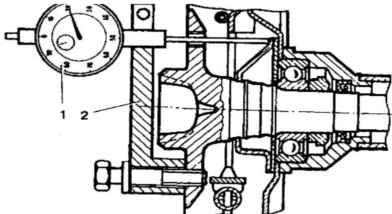
Рисунок 7 - Замер осевого люфта полуоси со снятым колесом и тормозным барабаном
