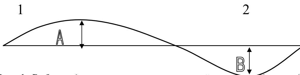
Рис. 1. Рабочая диаграмма телескопической стойки подвески (амортизатора задней подвески).
