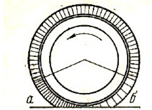
Рис 12 Окружная деформация шины при передаче крутящего момен- та; a — зона сжатия; б — зона рас- тяжения
