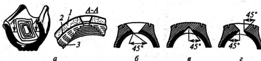
Рис. 1. Способы вырезки поврежденных участков покрышки: а — в ступенчатую рамку; б — внутренним конусом; в — наружным конусом; г — встречным конусом; 1 — протектор; 2 — брекер; 3 — каркас
