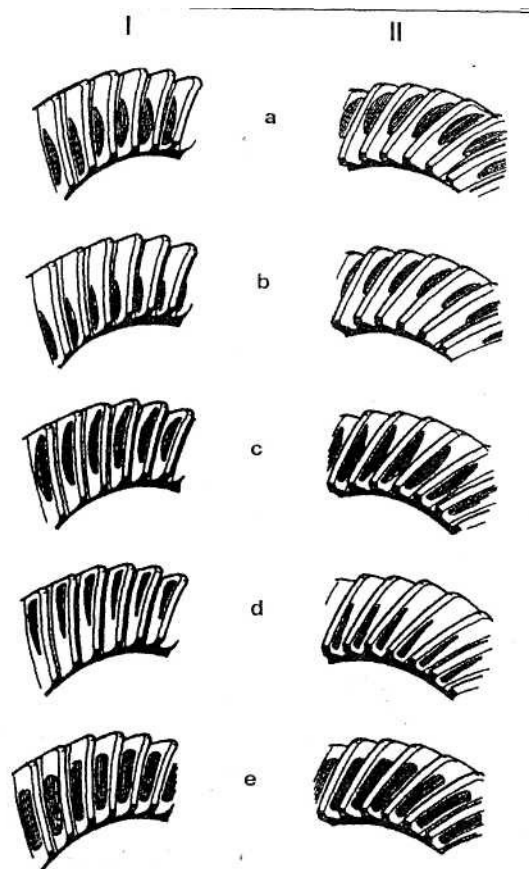
Рис. 11. Расположение пятна контакта в зацеплении шестерен главной передачи: I - сторона переднего хода; II - сторона заднего хода; а и b- неправильный контакт в зацеплении шестерен: отодвиньте ведущую шестерню от ведомой уменьшив толщину регулировочного кольца; с и d — неправильный контакт: придвиньте ведущую шестерню к ведомой, увеличив «толщину регулировочного кольца; е - правильный контакт в зацеплении шестерён
