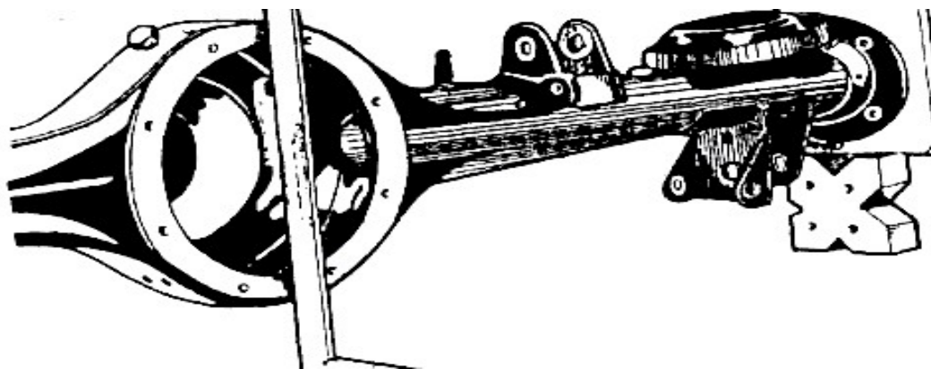
Рис 6 - Проверка перпендикулярности поверхности крепления редуктора
