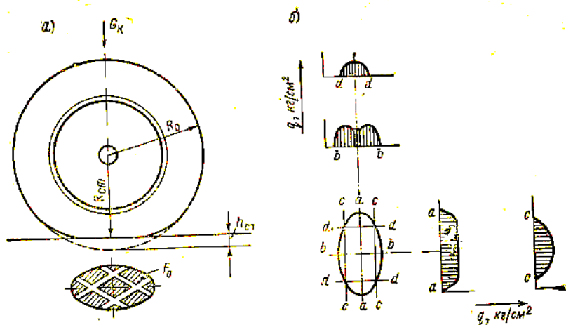
Рис. 11 Радиальная деформация шины:
