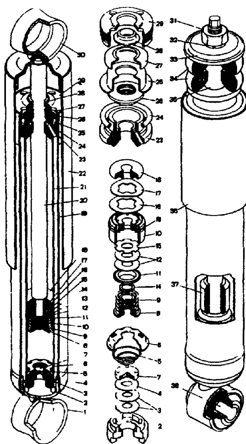
Рис. 16. Амортизаторы передней и задней подвесок.
