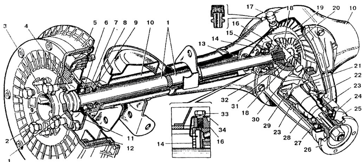
Рисунок 3- Задний мост
