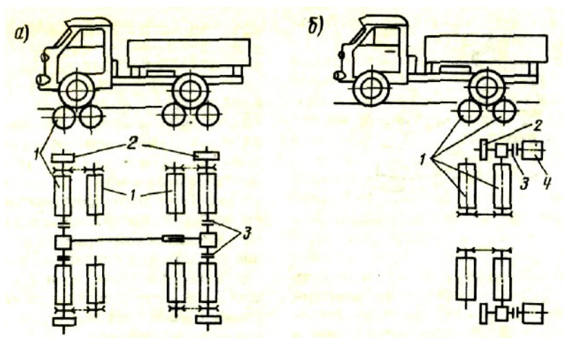
Рисунок 2 - Инерционные тормозные стенды с беговыми барабанами: а — с приводом от ведущих колес автомобиля. б — с приводом от электродвигателей
