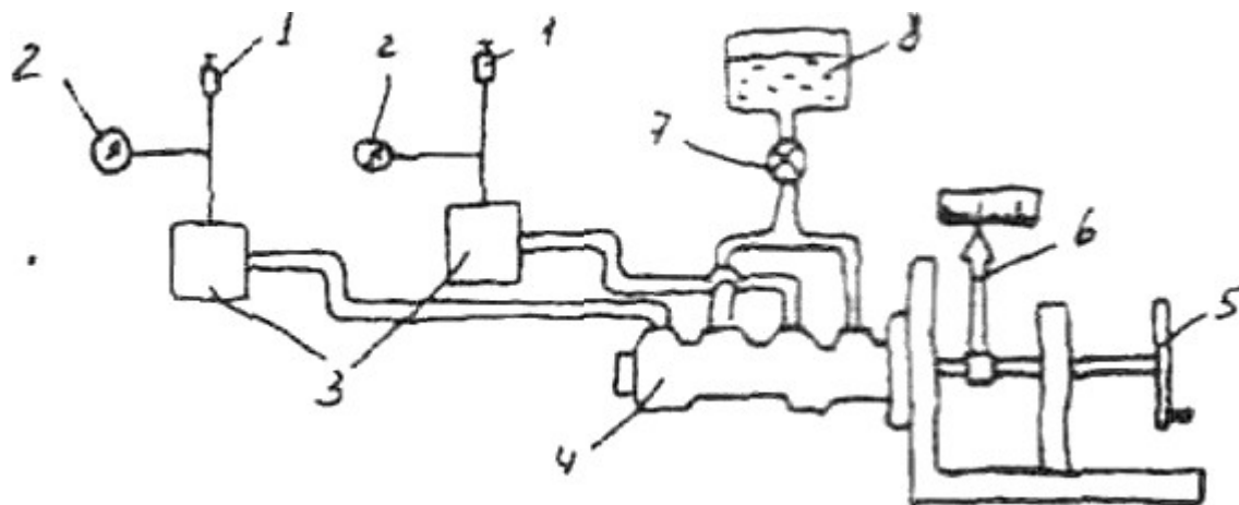
Рис. 1. Схема проверки герметичности главного цилиндра:
