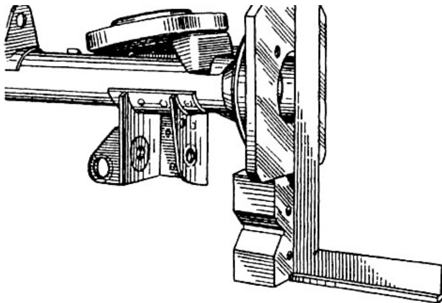
Рис. 4. Проверка вертикальных деформаций балки заднего моста с помощью угольника по наружной поверхности фланца А.70172
