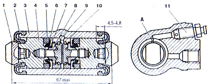
Рис. 1. Схема заднего рабочего тормозного цилиндра автомобиля ВАЗ-2107
