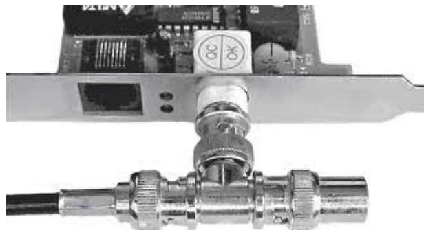
Рис. 2. Т-коннектор, присоединенный к сетевой карте
