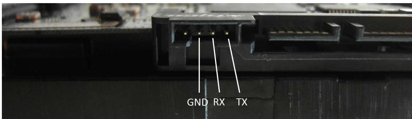
ис. 2. Разъем для подключения через последовательный порт. Одной тайной меньше
