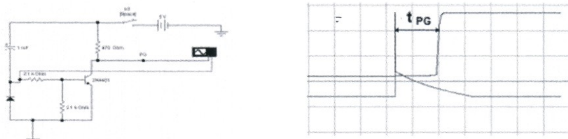
Рисунок 2 - Схема выработки сигнала PG
