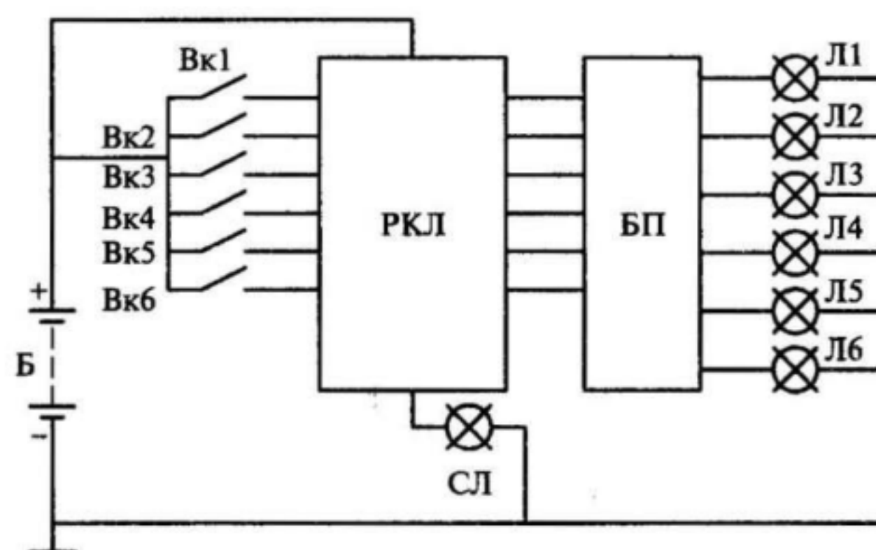
Рис. 7.15. Функциональная схема реле контроля ламп световых приборов: Б — аккумуляторная батарея; Вк1... Вк6 — выключатели цепей подконтрольных ламп; БП — блок предохранителей; РКЛ — реле контроля исправности ламп; Л1... Л6 — подконтрольные лампы световых приборов; СЛ — сигнальная лампа
