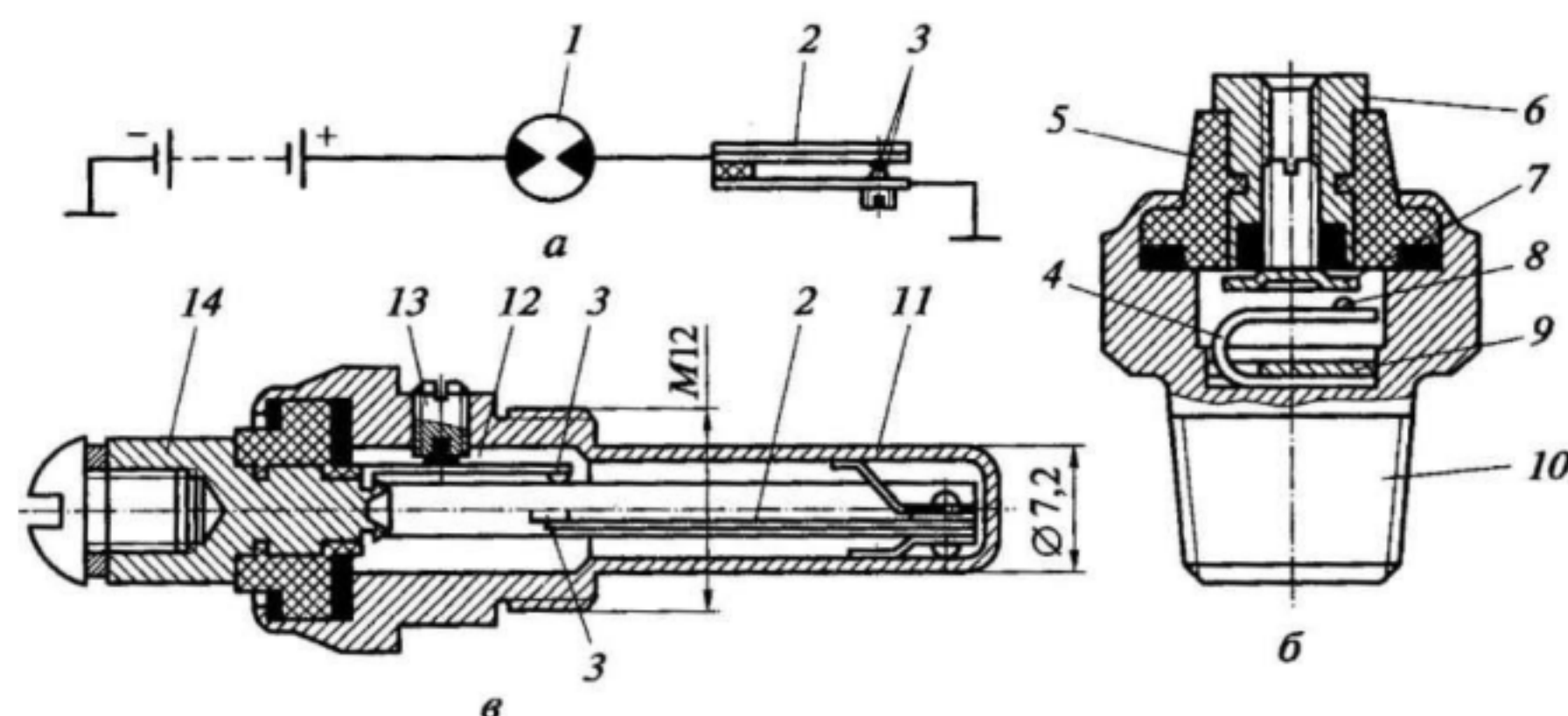
Рис. 7.2. Схема сигнализации аварийной температуры:
