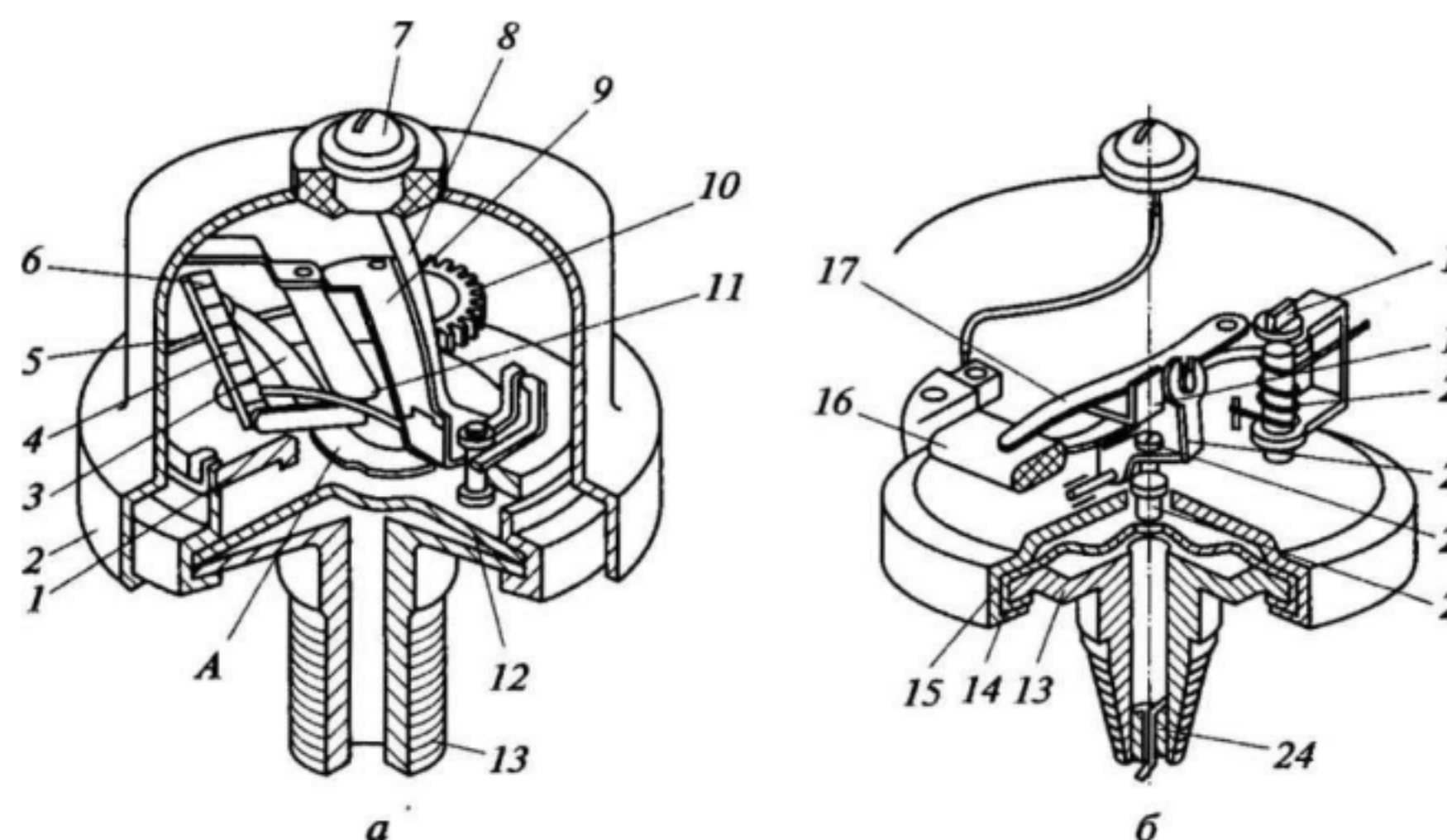
Рис. 7.5. Датчики давления:
