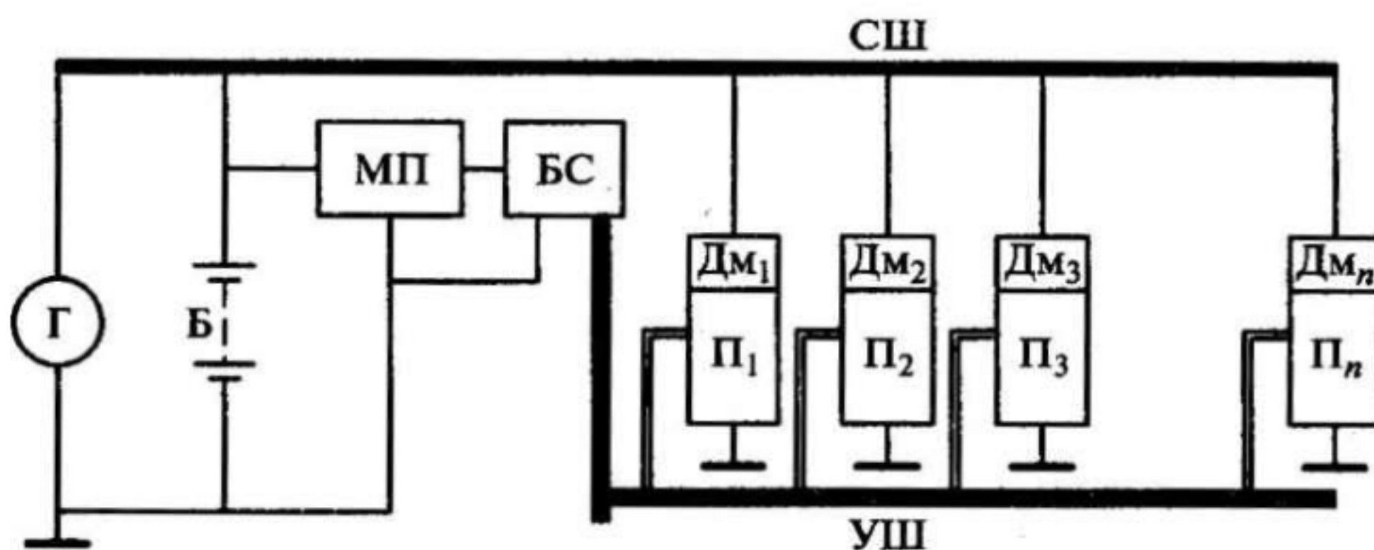
Рис. 9.1. Функциональная схема варианта мультиплексной системы.
