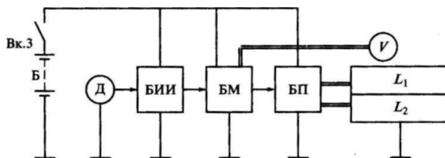
Рис. 7.12. Функциональная схема электронного спидометра: Б — аккумуляторная батарея; Вк.З — включатель зажигания; Д — датчик импульсов; БИИ — блок измерения импульсов; БМ — блок установки масштаба; БП — блок памяти; V — стрелочный магнитоэлектрический прибор измерения скорости; L_1 и L_2 — информационные узлы счетчика пути от конкретного места и от начала эксплуатации
