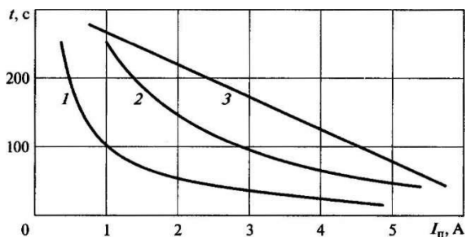
Рис. 9.2. Ампер-секундные характеристики:
