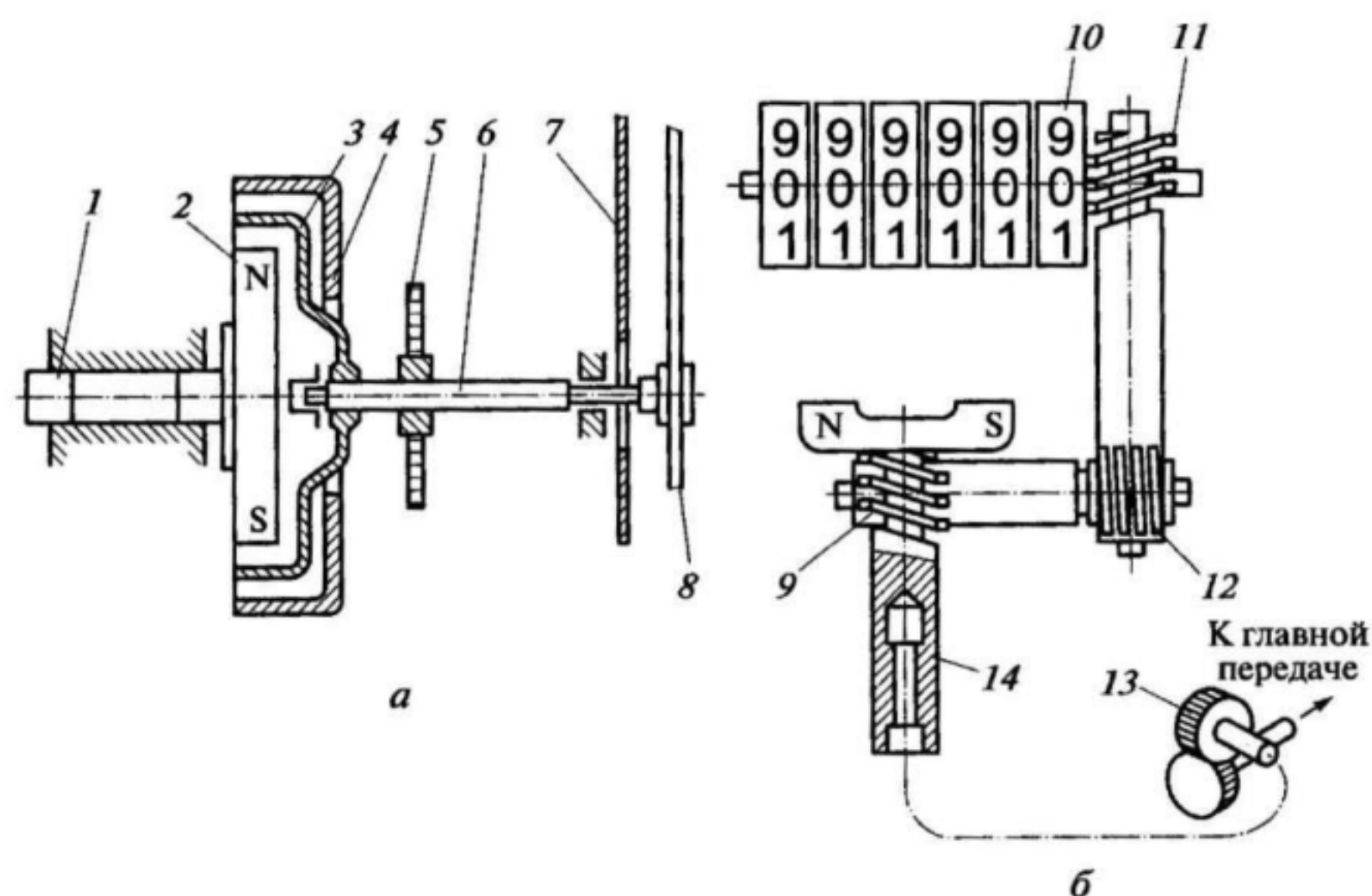
Рис. 7.9. Схема действия спидометра с приводом от гибкого вала: а — магнитоиндукционный скоростной узел; б — привод счетного узла; 1 — приводной валик; 2 — постоянный магнит; 3 — алюминиевая катушка; 4 — магнитный экран; 5 — возвратная пружина; 6 — ось стрелки; 7 — шкала; 8 — стрелка; 9 — ведущий червяк; 10 — начальный барабанчик счетного узла; 11 — ведомый червяк; 12 — промежуточный червяк; 13 — винтовой редуктор; 14 — входной валик
