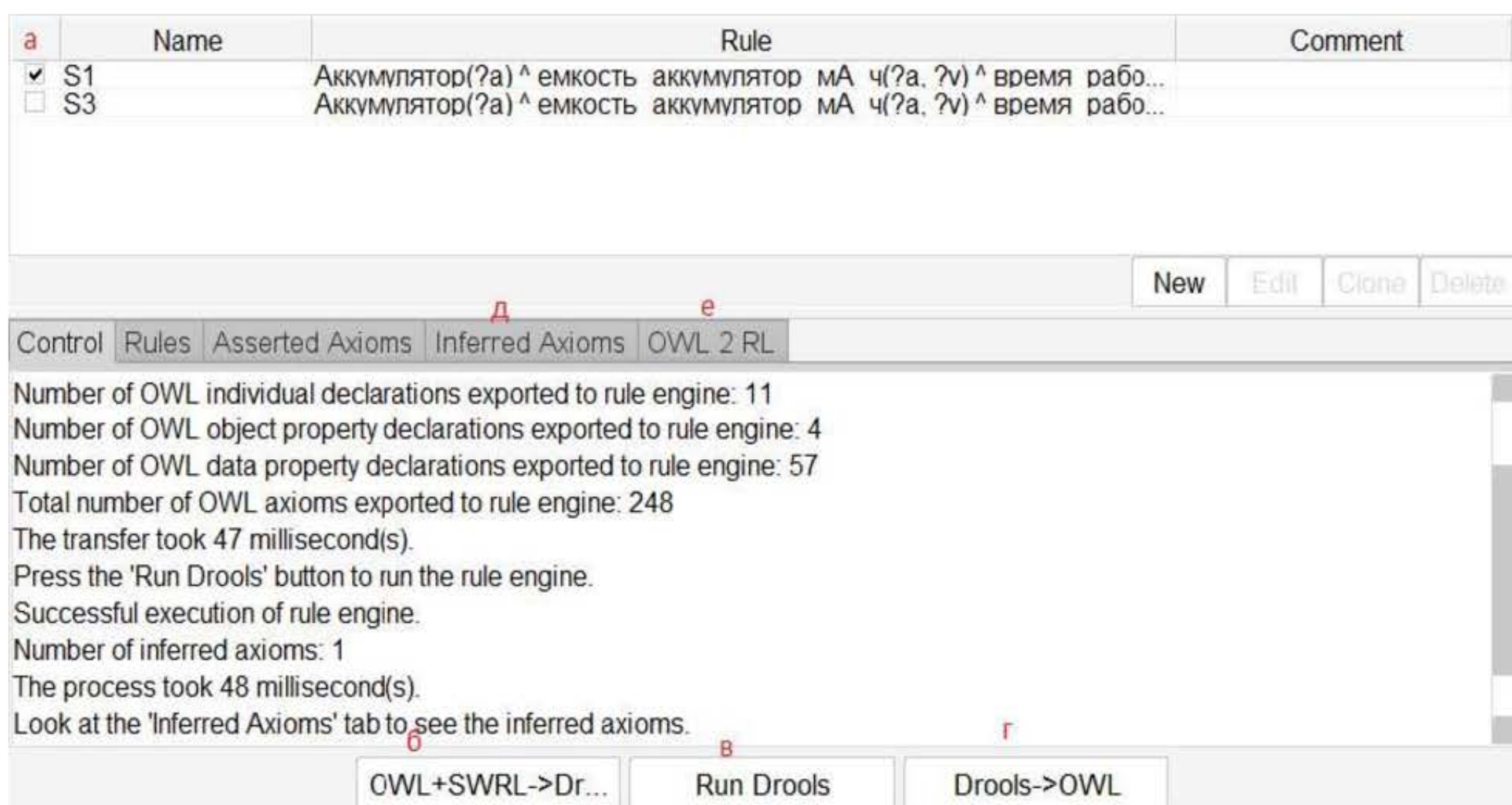
Рис. 26 Вкладка SWRL в системе Protégé (а – активность правила; б – кнопка и списка правил; в – запуск вывода на основе правил; г – внесение выведенных понятий в онтологию; д – список
