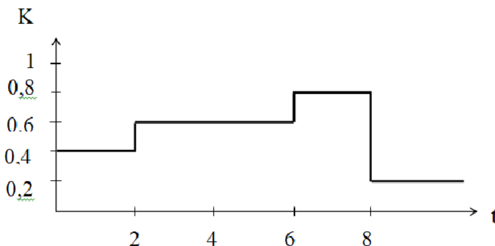
Рисунок 2.1- График нагрузки трансформатора
