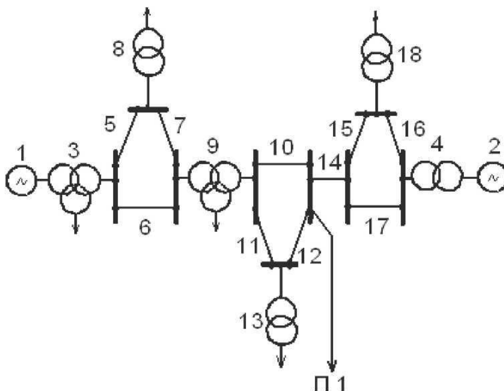
Рис.3. Схема системы электроснабжения потребителя III
