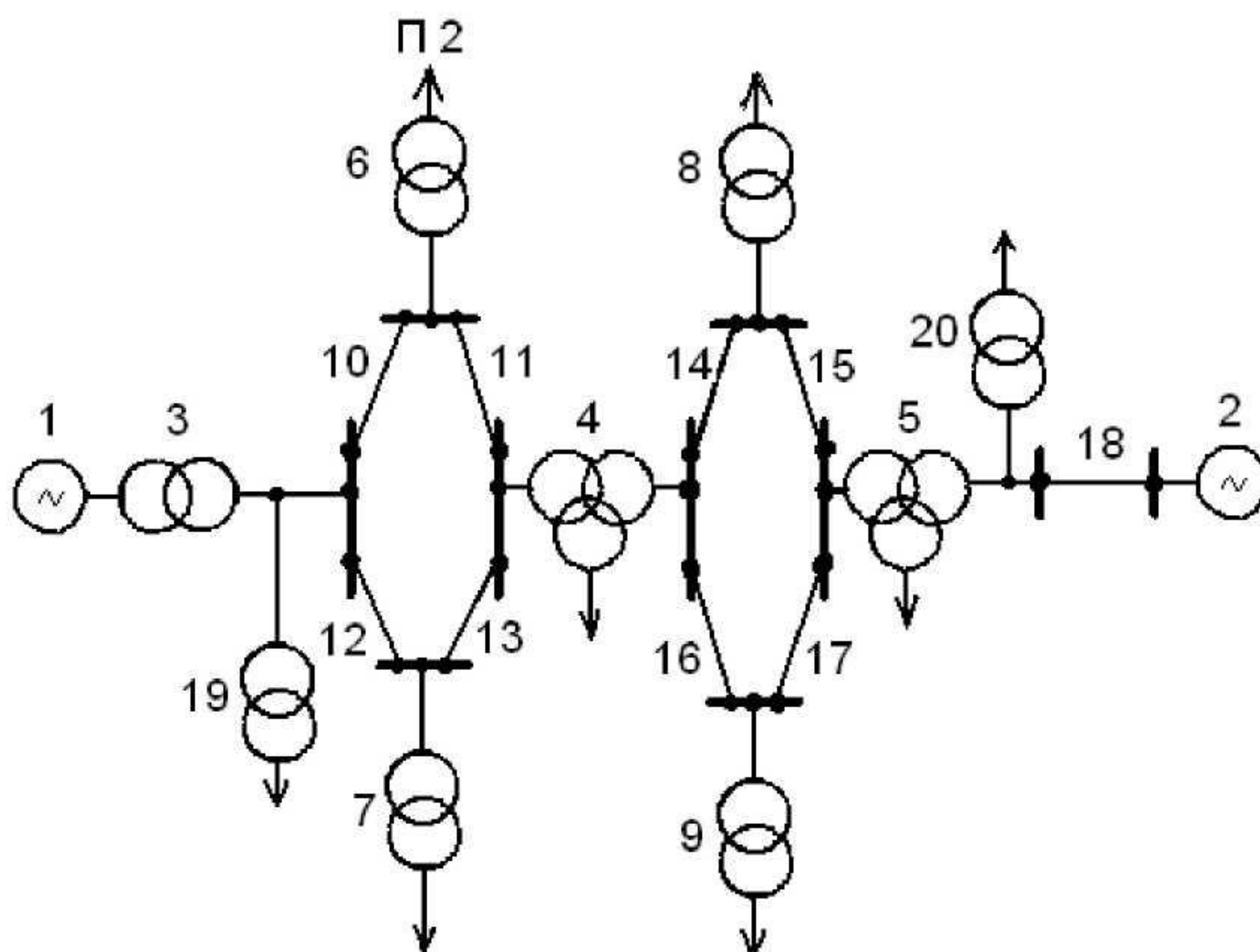
Рис.4. Схема системы электроснабжения потребителя П2
