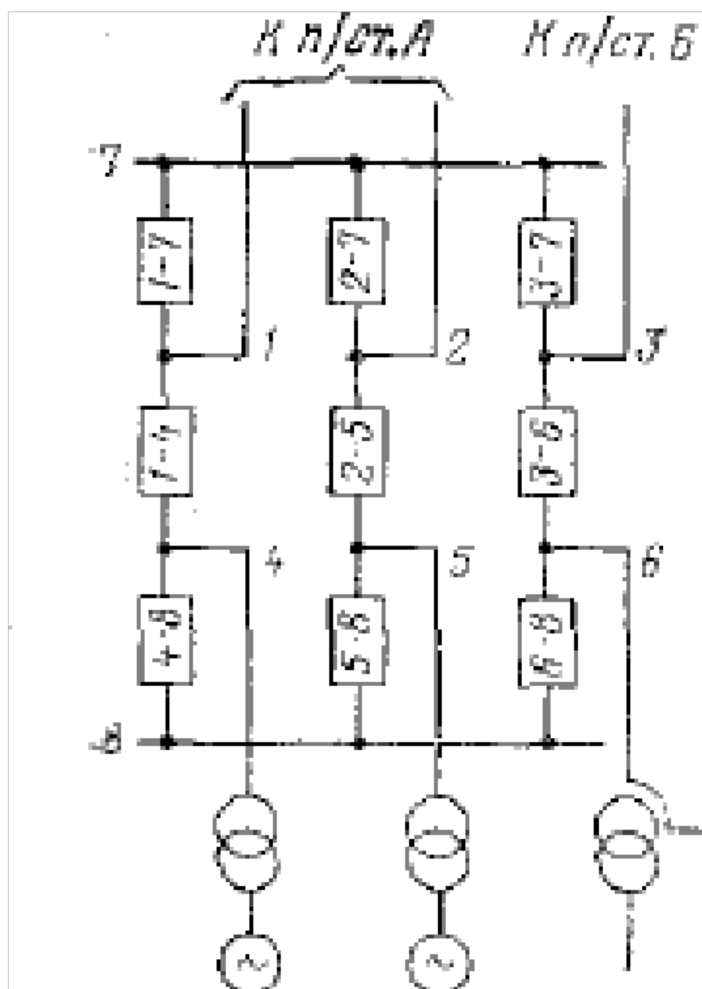
Рис. 4.1. Схема распределительного устройства
