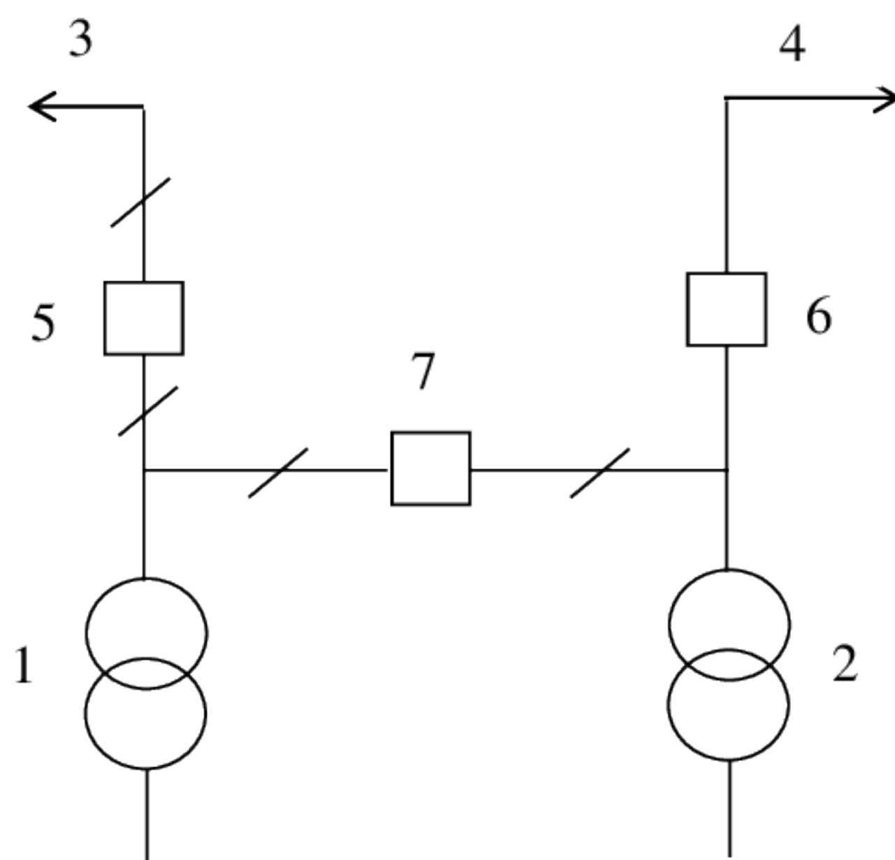
Рисунок 1.1- Расчетная схема подстанции
