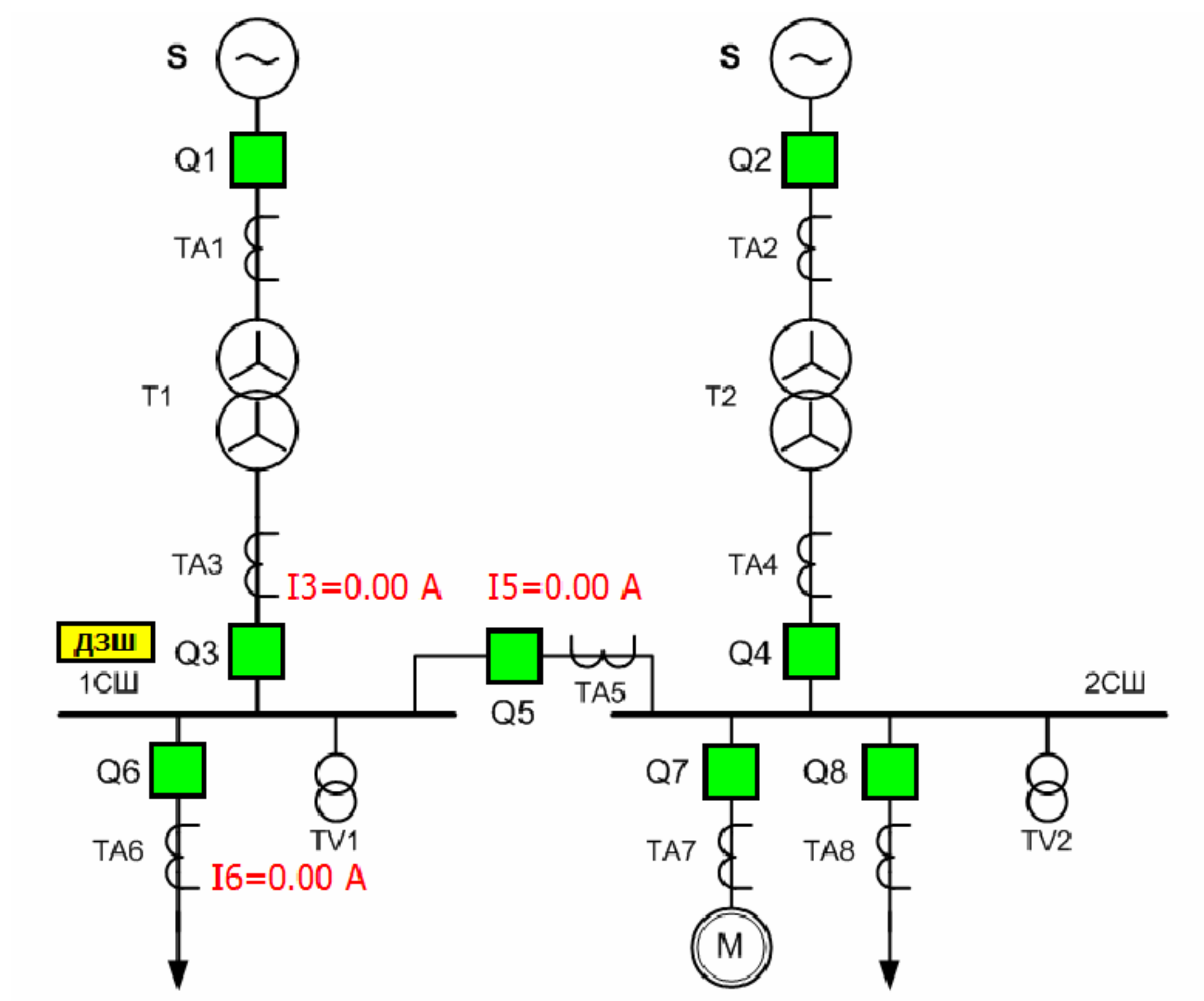
Дифференциальная защита сборных шин. Мнемосхема
