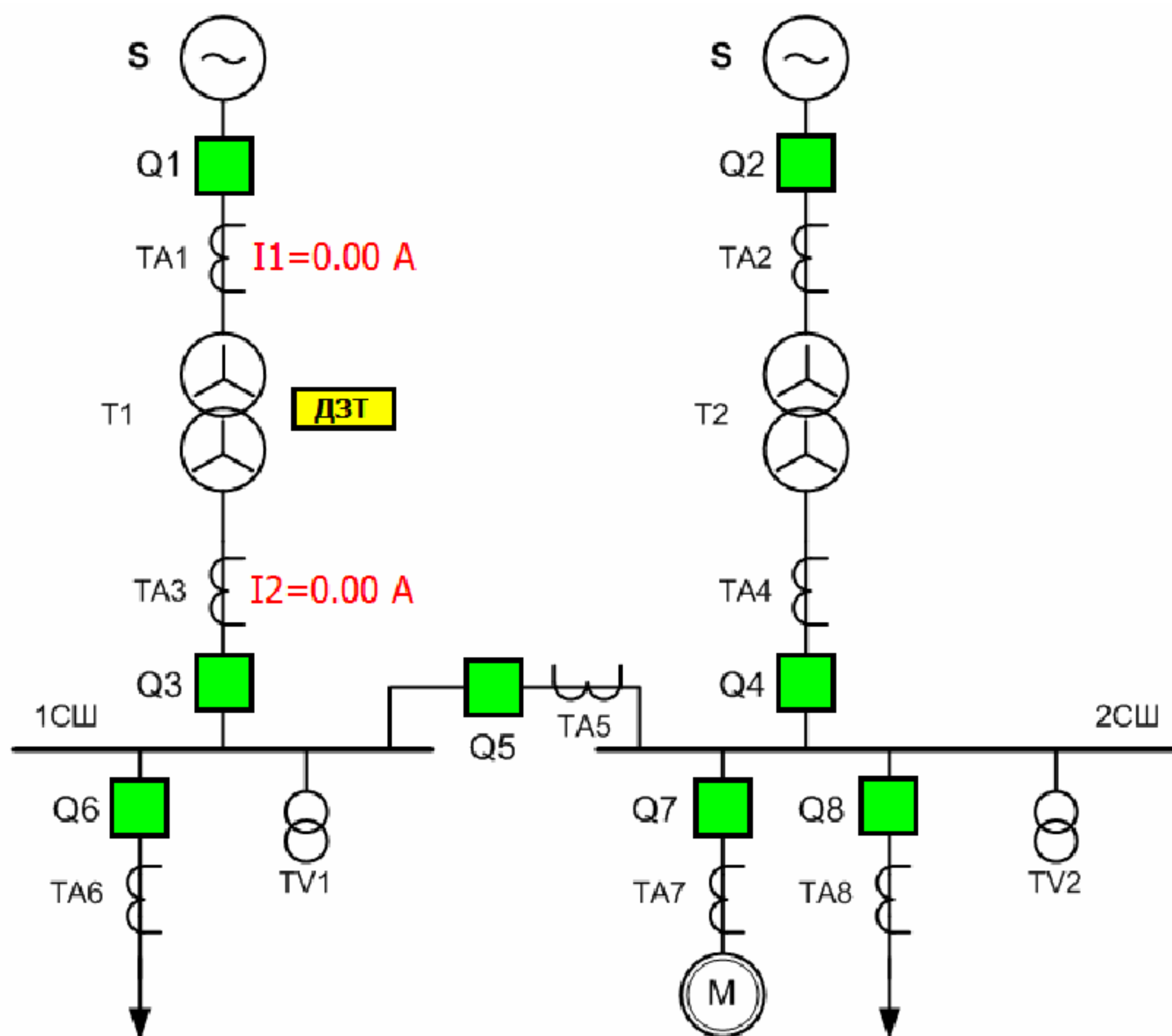
Дифференциальная защита трансформатора. Мнемосхема
