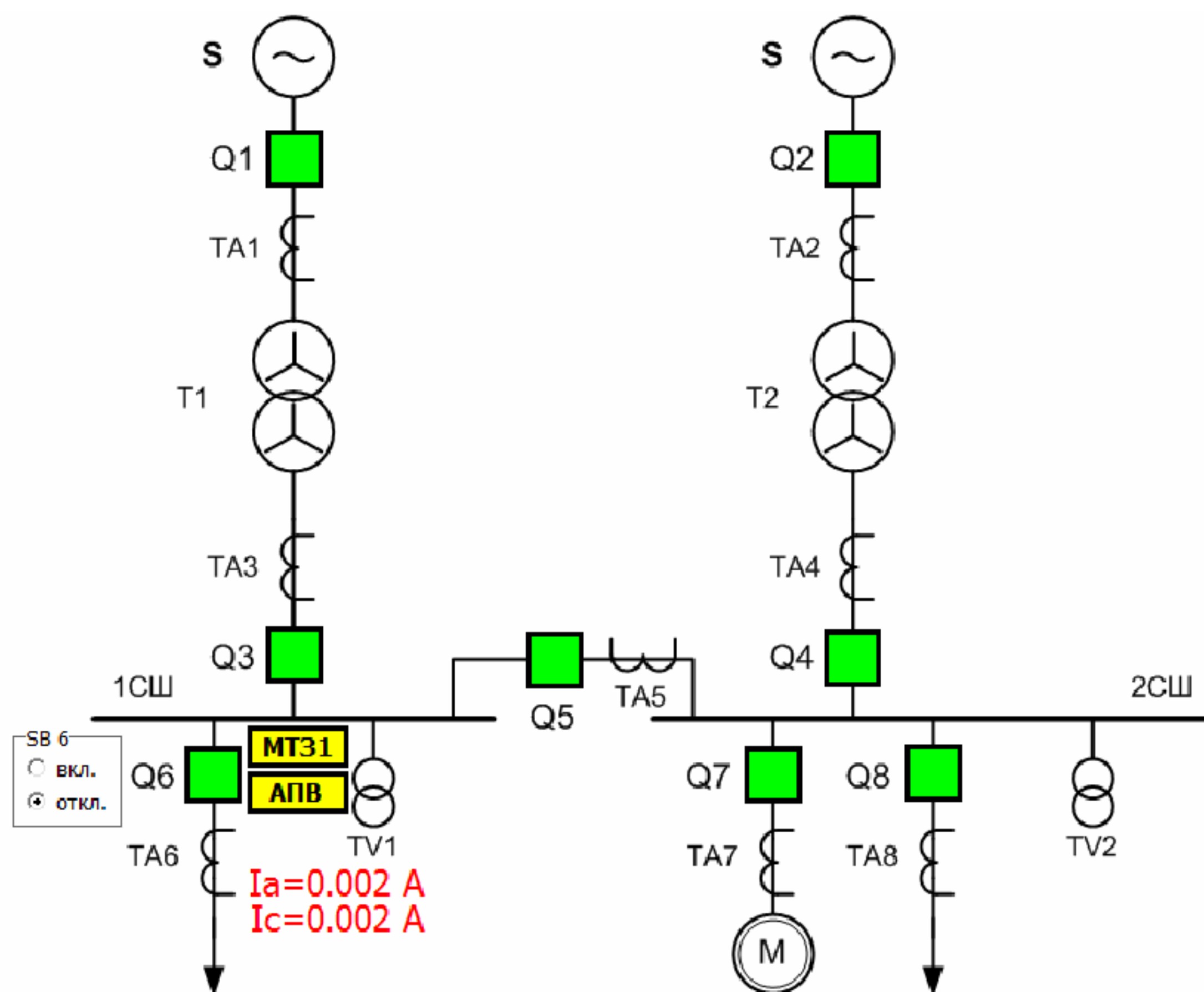
Автоматическое повторное включение линии электропередачи. Мнемосхема
