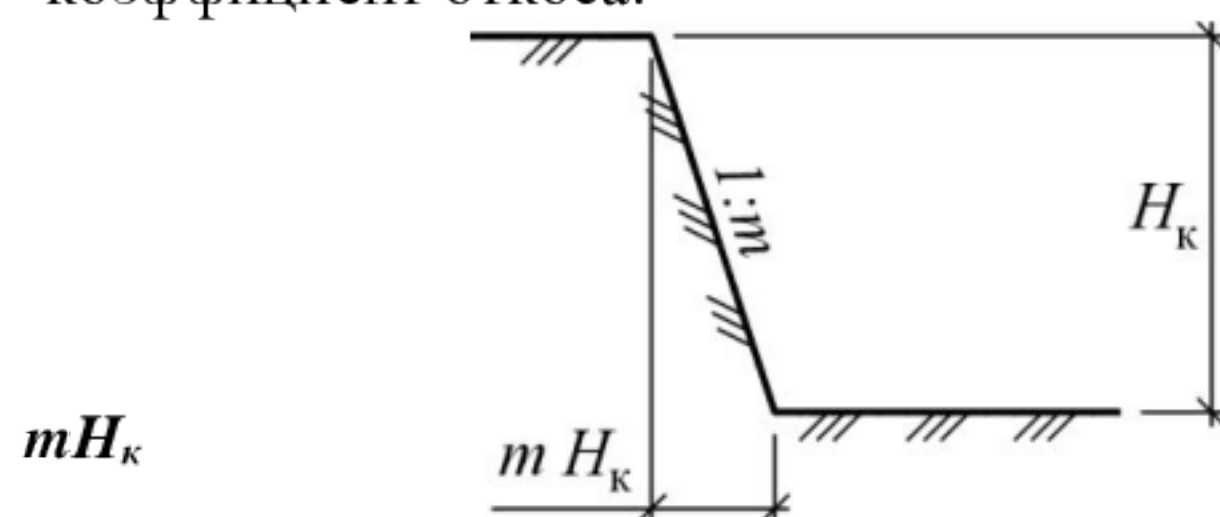
Рис. 3. Схема откоса
