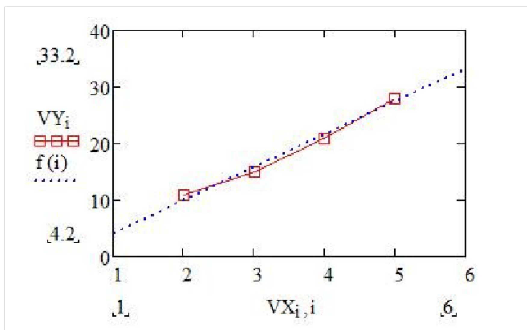
Рисунок 4.2 -Линейная регрессия
