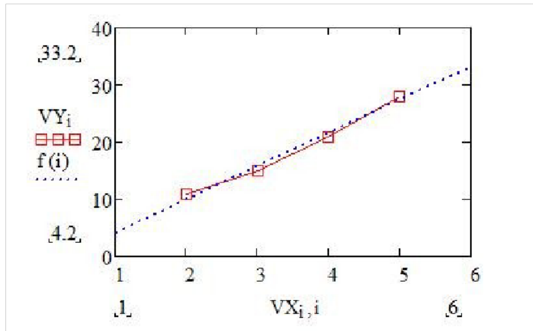
Рисунок 4.2 -Линейная регрессия
