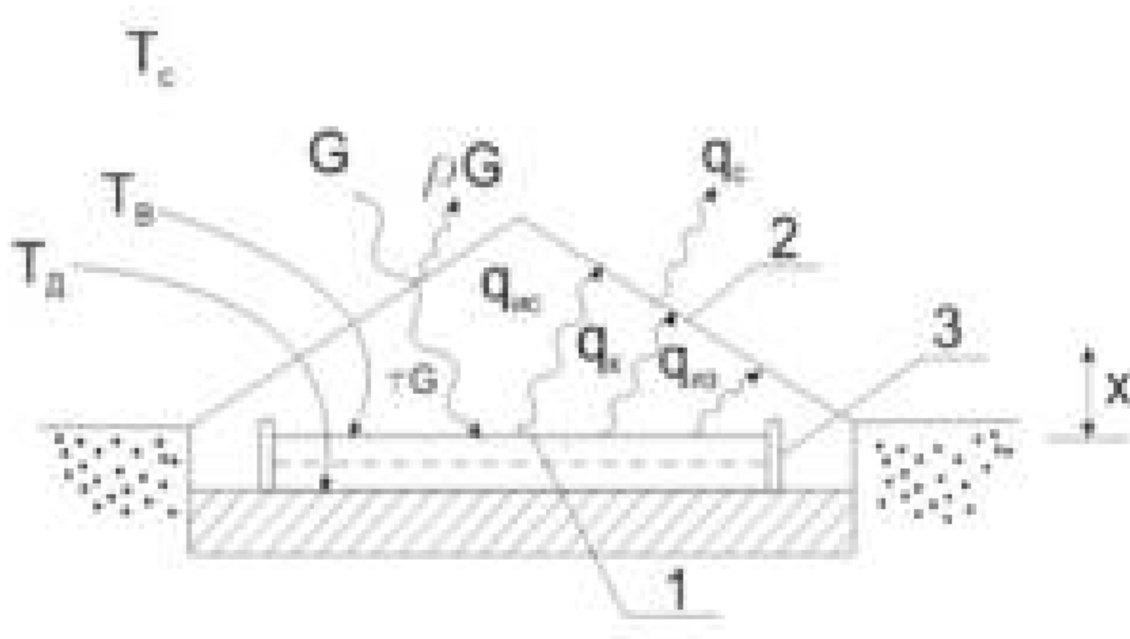
Рисунок 1 – Потоки тепла в солнечном дистилляторе.
