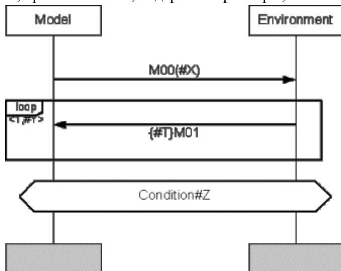
Рис. 10.7. Макроподстановки
