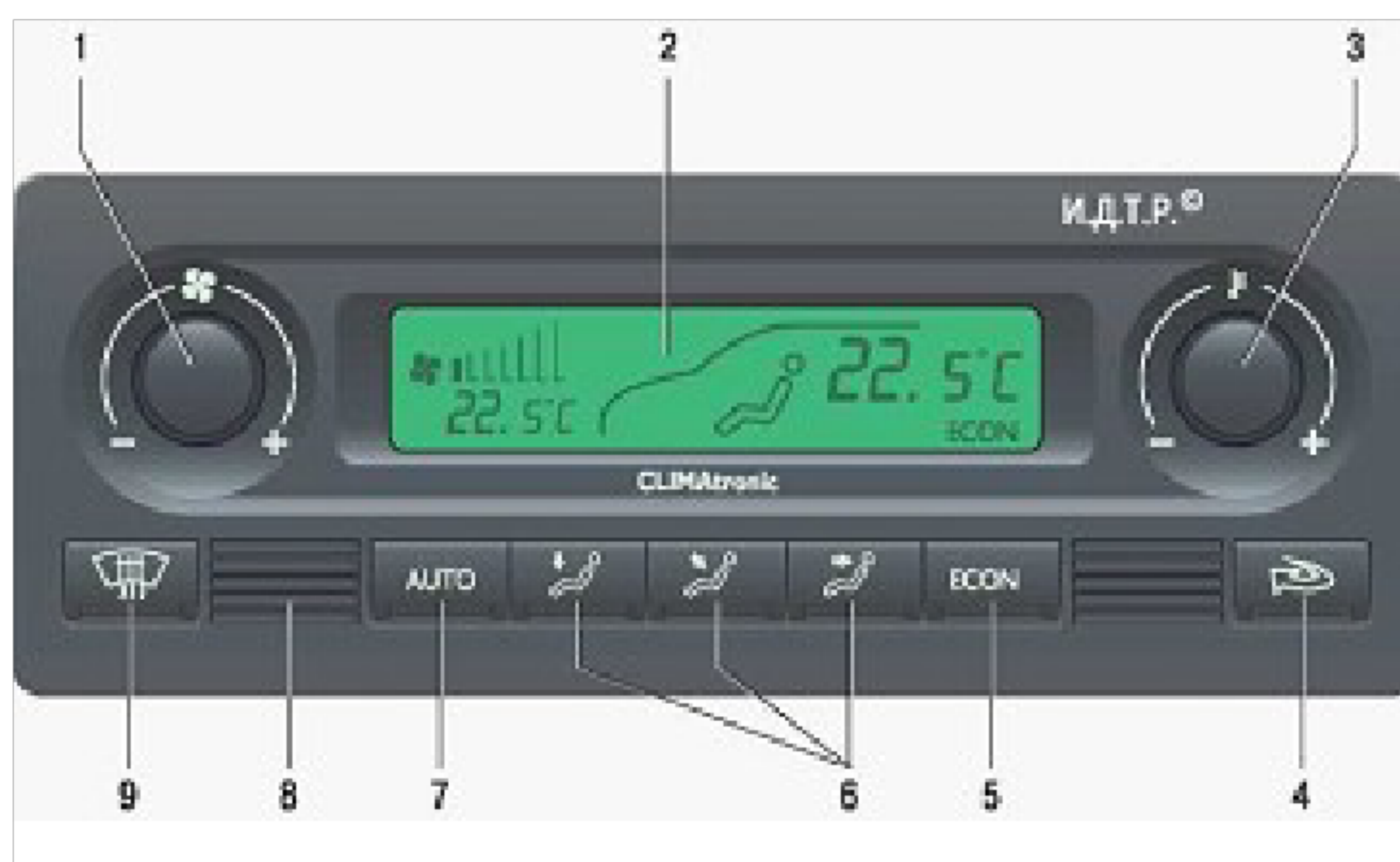
Рис. 5. Блок автоматического управления системой отопления(кондиционирования) и вентиляции салона: 1 - переключатель режимов работы электровентилятора воздухонагнетателя; 2 - дисплей; 3 - регулятор температуры поступающего в салон воздуха; 4 - выключатель режима рециркуляции; 5 - выключатель кондиционера; 6 - переключатели распределения потоков воздуха; 7 - выключатель автоматического режима
