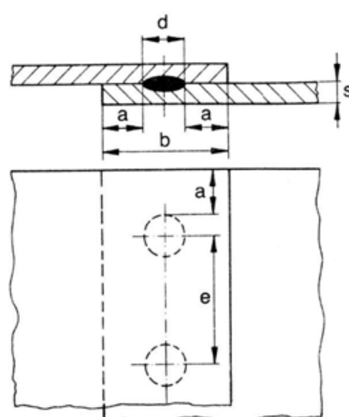
Рис. 14. Геометрические параметры контактно точечной сварки:
