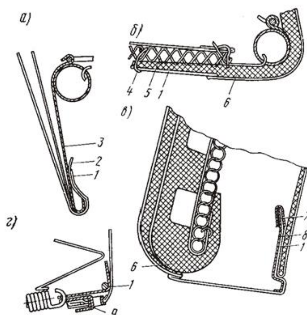
Рис. 3. Крепление обивки сидений:
