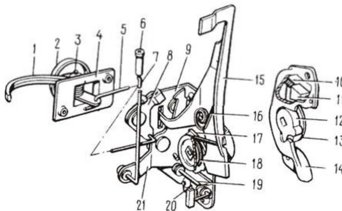
Рис. 1. Замок передней левой двери:
