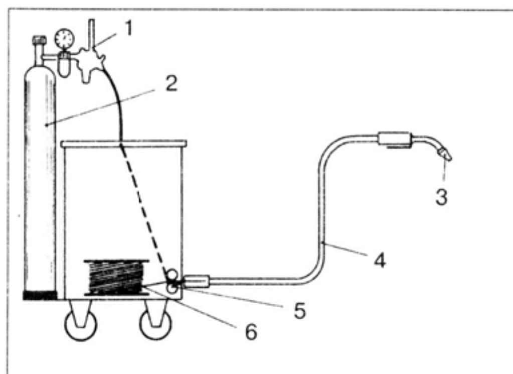
Рис. 10. Схема аппарата для сварки в среде защитного газа:
