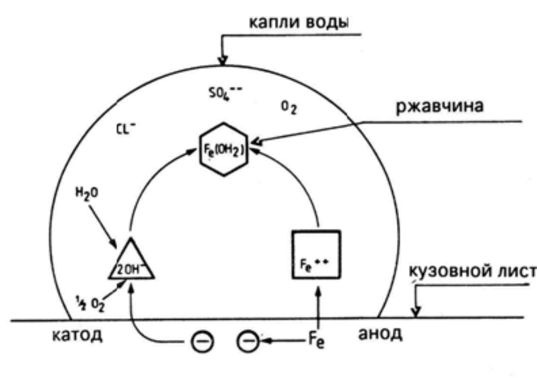
Рис. 18. Схематичное изображение процесса коррозии
