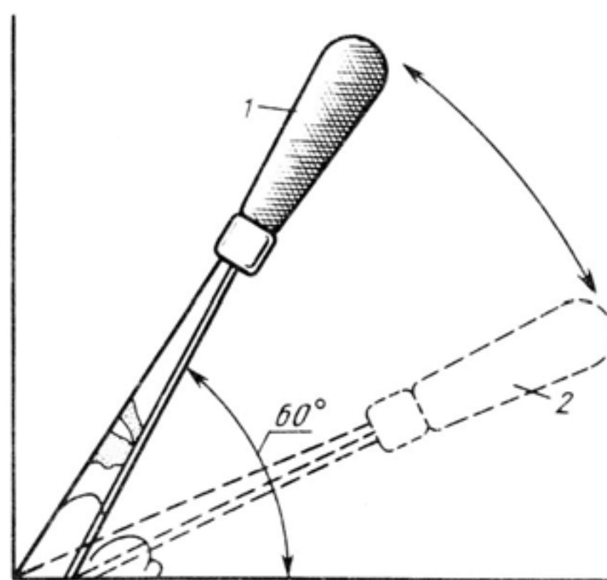
Рис. 15. Положение шпателя при шпатлевании: 1 – хорошо; 2 – плохо
