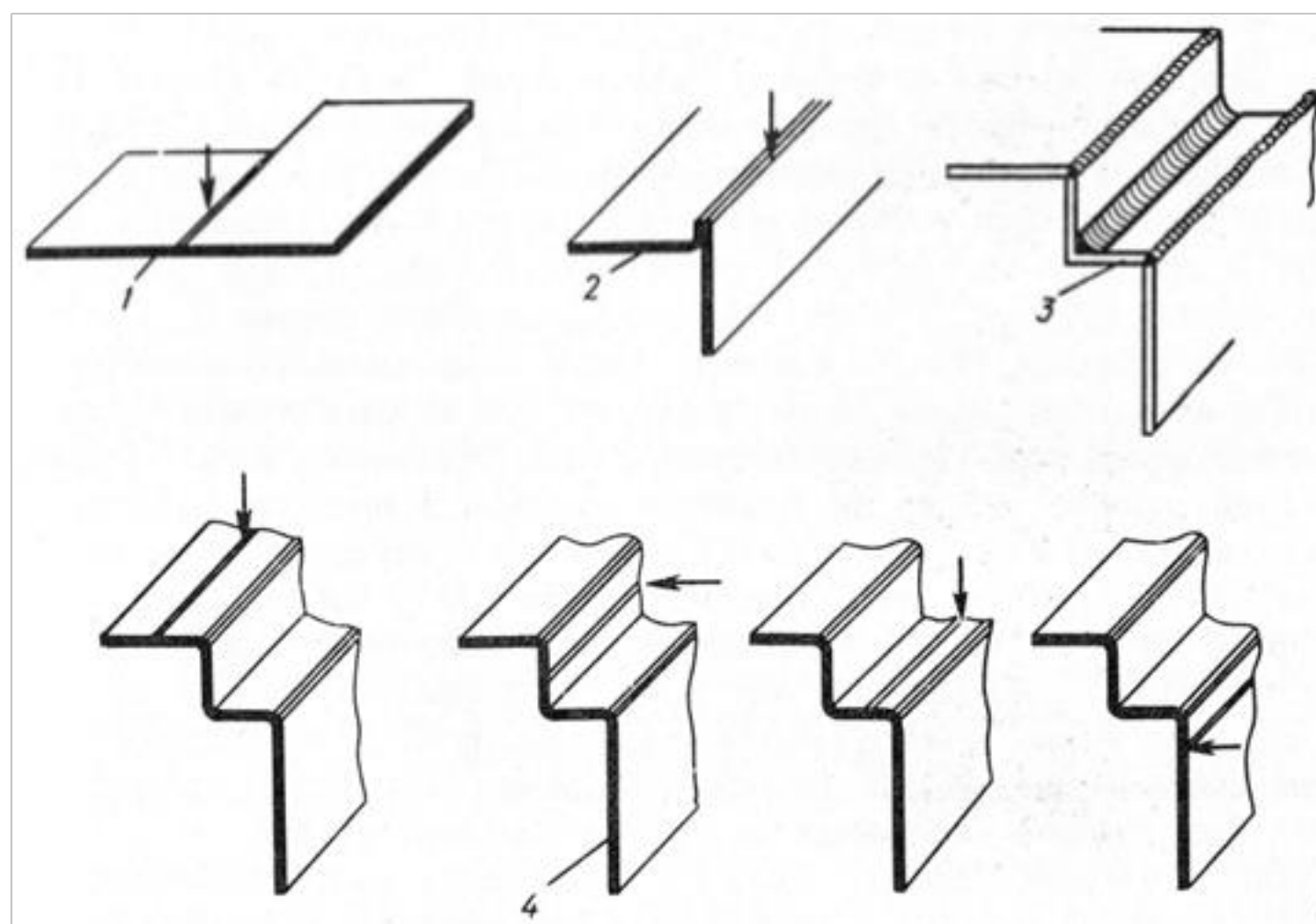
Рис. 6. Подготовка кромок тонких листов под сварку: 1 – сварка встык; 2 – сварка с отбортовкой кромки; 3 – сварка внутренних или наружных углов не подвергается рихтовке; 4 – хорошее расположение сварочного шва, позволяющего производить рихтовку
