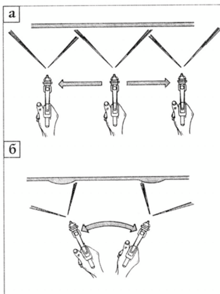
Рис. 17. Правильное (а) и неправильное (б) положение пистолета-распылителя
