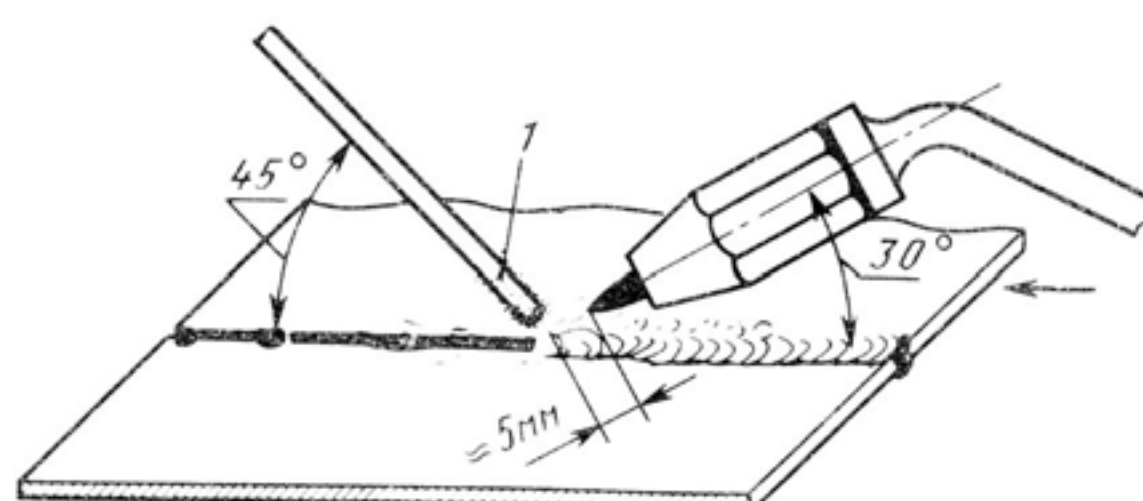
Рис. 5. Расположение горелки и припоя при пайке латунным припоем: I – пороховый флюс, нанесенный на конец припоя или прутка, покрытый флюсом
