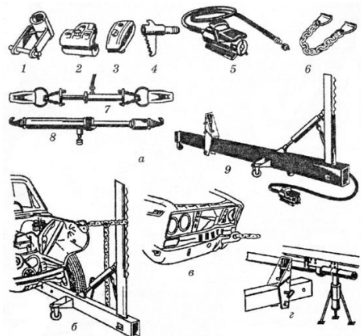
Рис. 17. Приспособления для выполнения правки деформированного участка кузова:
