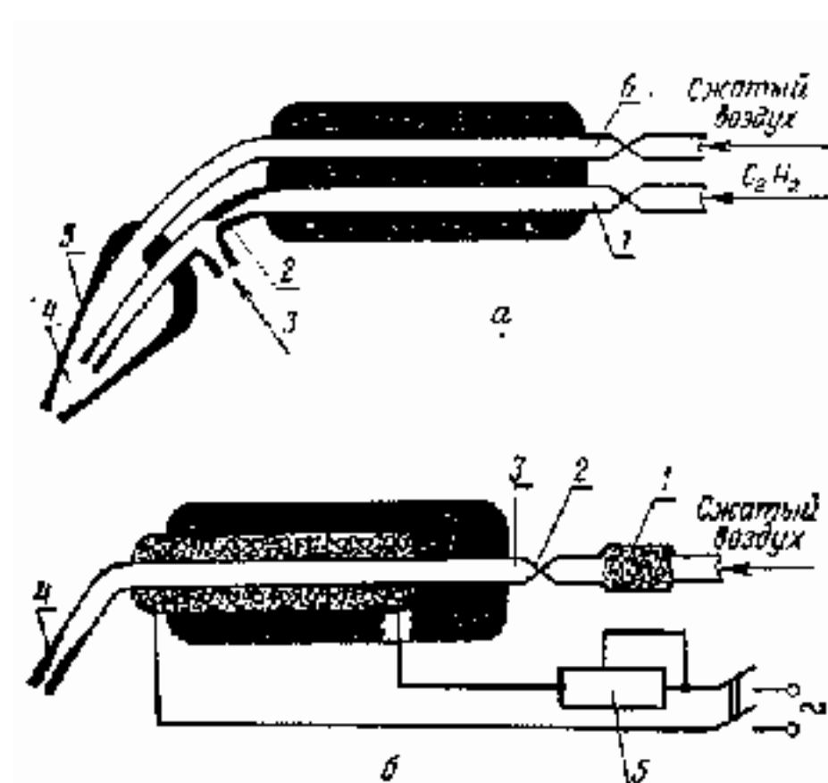
Рис. 2. Схема горелок для сварки термопластов горячими газами: а – газовая горелка ГГП-1-56; б – газозлектрическая горелка
