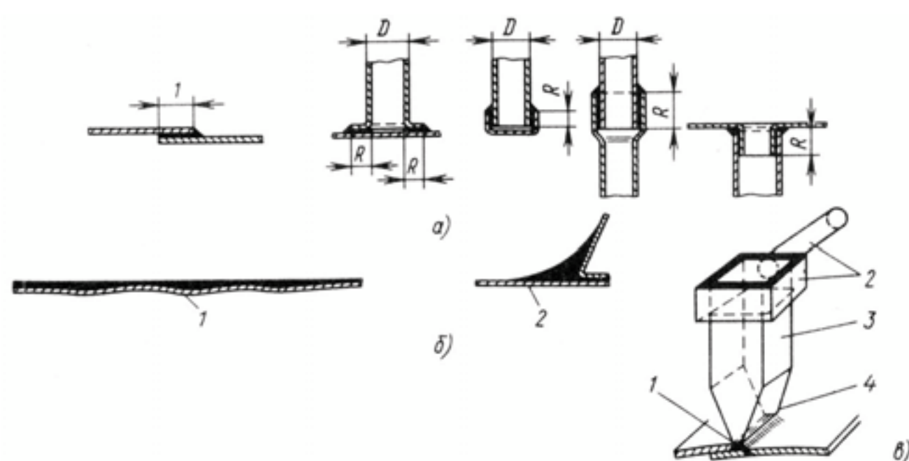
Рис. 3. Пайка оловянным припоем:
