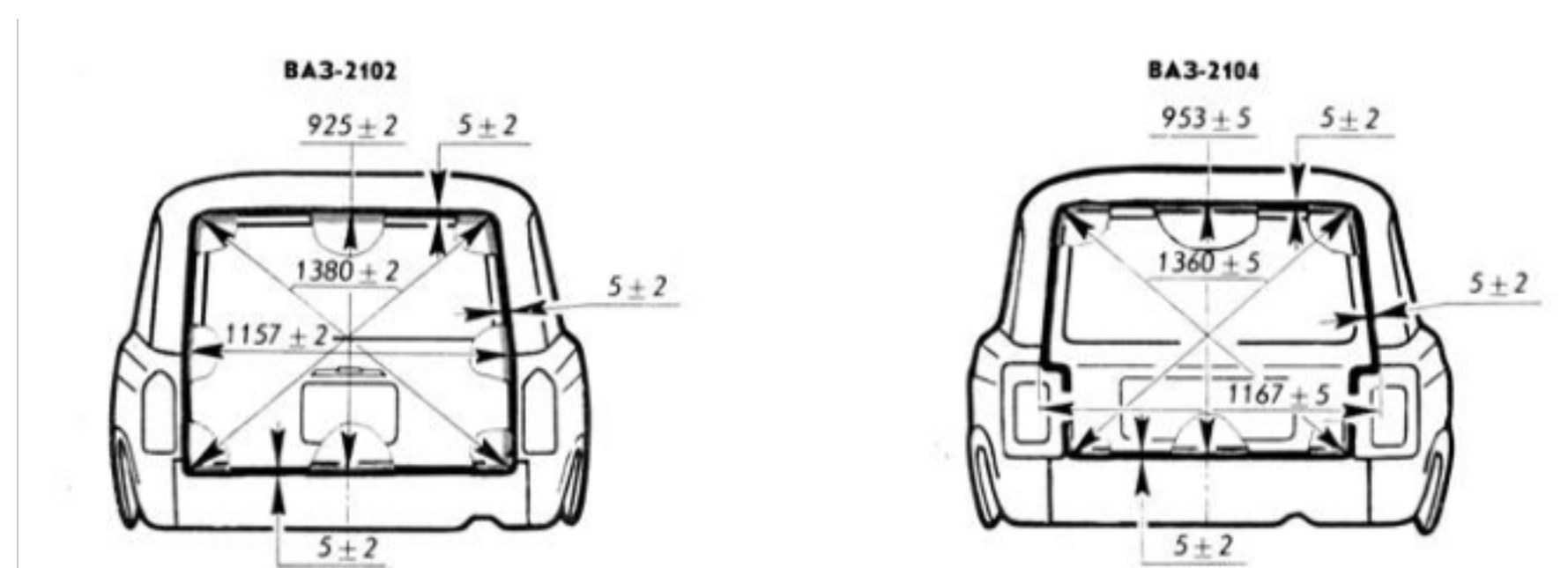
Рис. 6. Размеры проемов и зазоры сопрягаемых деталей кузова автомобилей моделей ВАЗ-2101 - 2107
