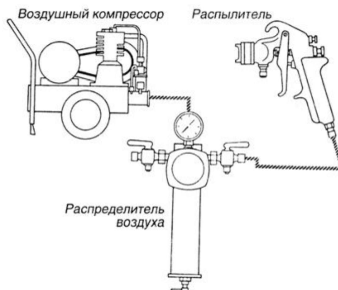
Рис. 16. Установка для нанесения лакокрасочных материалов распылением
