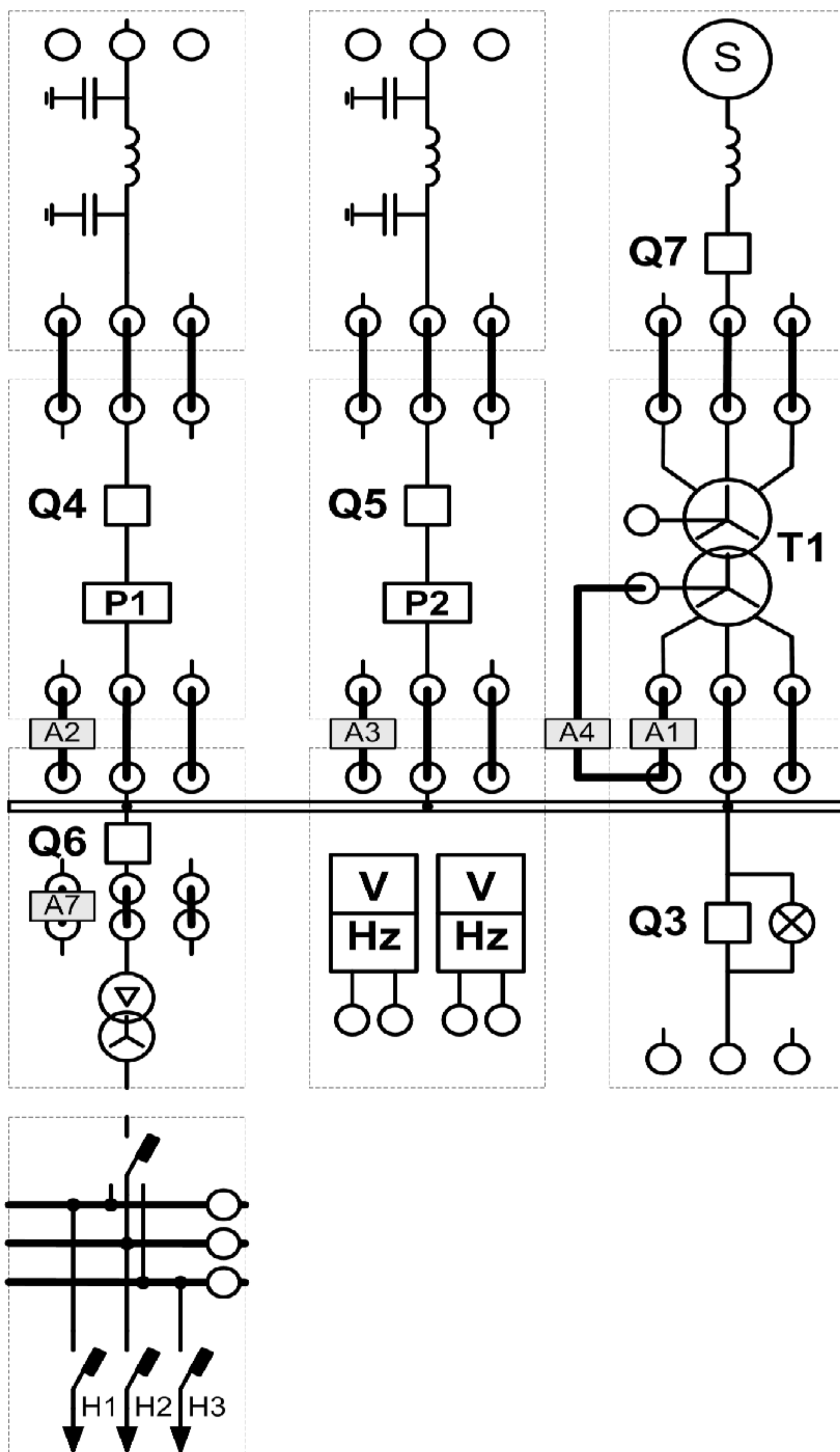
Рисунок 5.1 – Принципиальная схема «Балансирующий узел нагрузкой»
