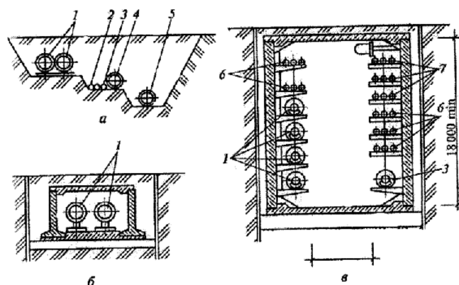
Рис. 2. Способы размещения инженерных сетей: а) в общей траншее; б) в непроходном коллекторе; в) в проходном коллекторе; 1 – теплосеть; 2 – газопровод; 3 – водопровод; 4 – водосток; 5 – канализация; 6 – кабели связи; 7 – силовые кабели.
