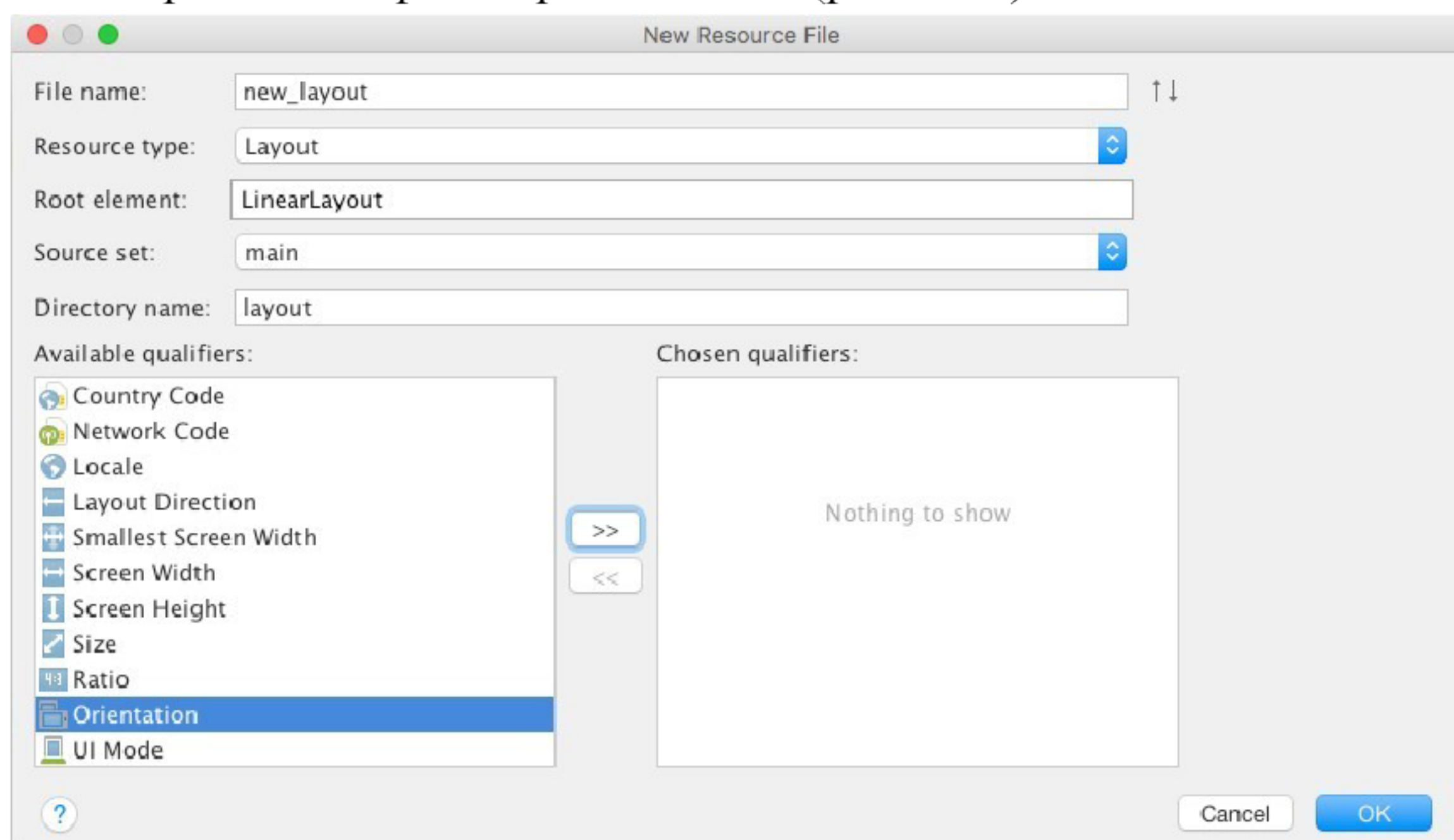
Рис. 5.10. Создание layout-файла с квалификатором
