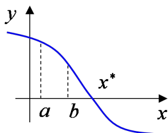
Рисунок 1 – Корни нелинейного уравнения
