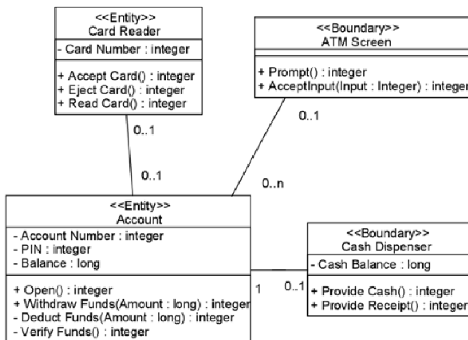
Рисунок 3.9 - Пример диаграммы классов
