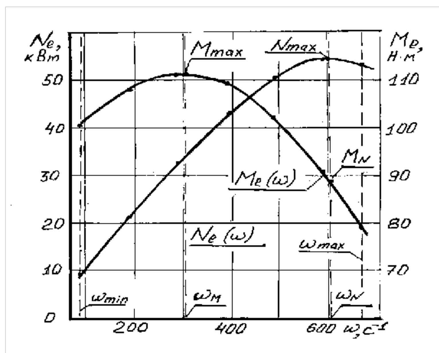
Рисунок 1- Внешняя скоростная характеристика двигателя автомобиля М-412 И Э
