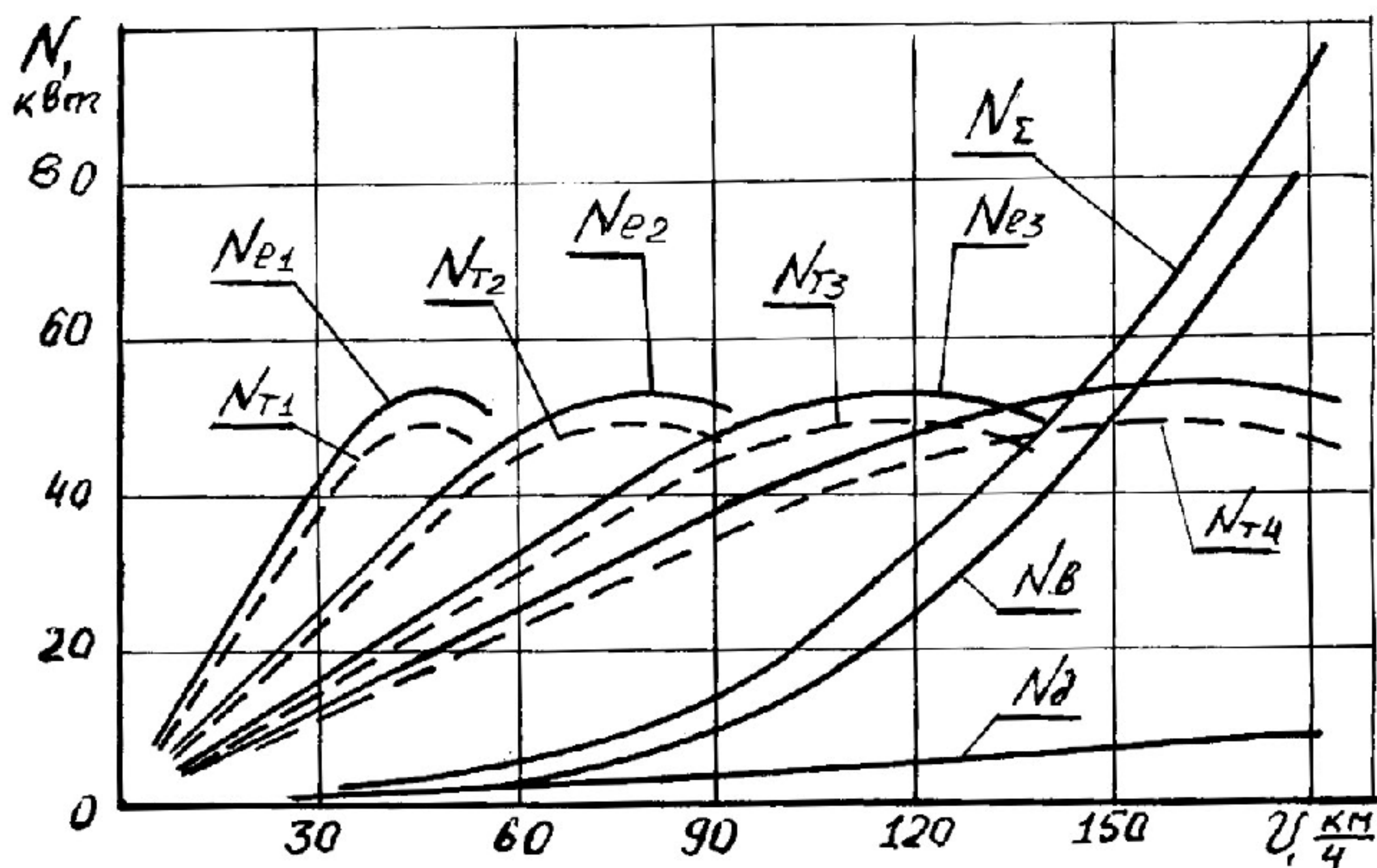
Рисунок 4- Графики мощностного баланса автомобиля М-412 И Э
