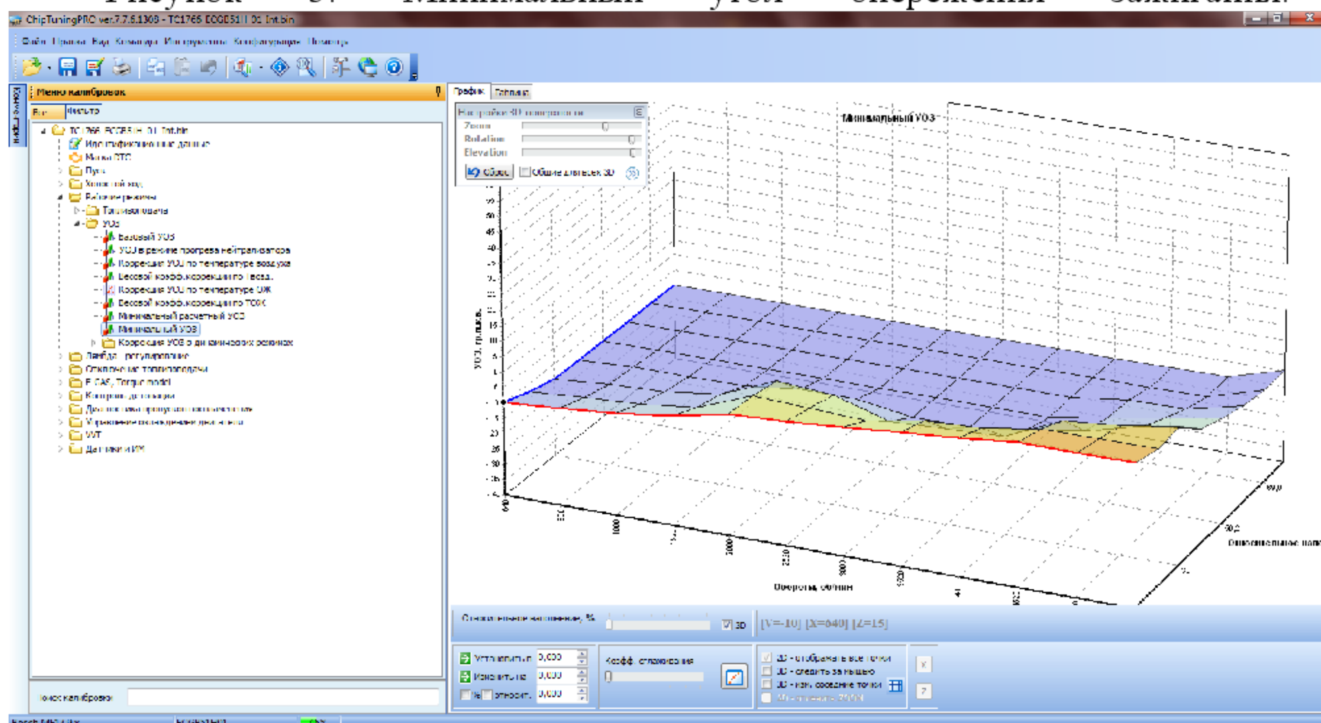
Рисунок 5. Минимальный угол опережения зажигания.
