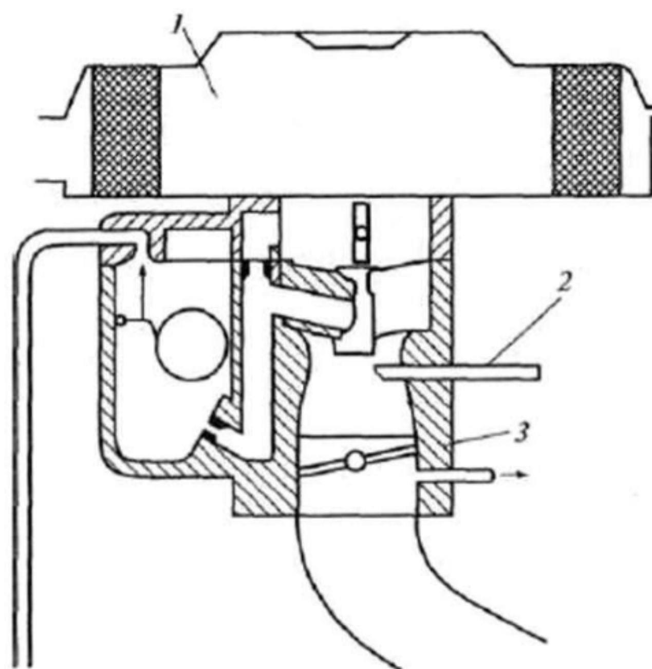
Рис. 4.6. Схема подачи газа через штуцер: 1 - воздушный фильтр; 2 - штуцер для подвода газа; 3 - корпус карбюратора
