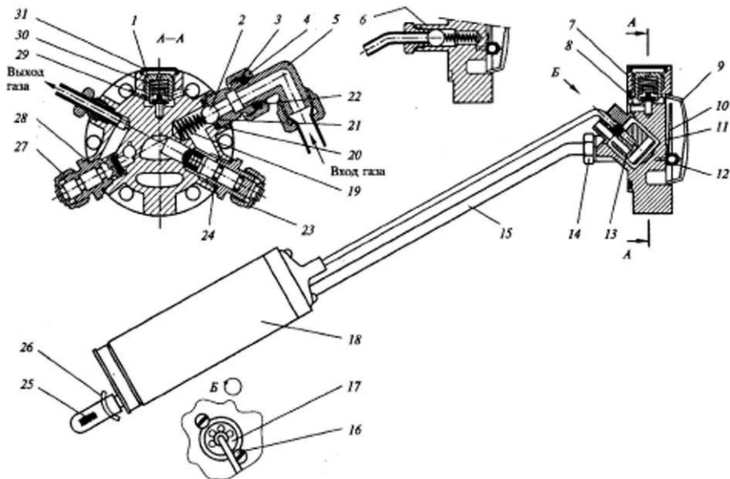
Рис.1.1. Мультиклапан: 1 - предохранительный клапан; 2 - шарик; 3 - штуцер входной; 4 - гайка; 5 - переходник; 6 - скоростной клапан; 7 - корпус; 8 - прокладка; 9 - прозрачный корпус; 10 - магнитная стрелка; 11 - шкала; 12 - ось стрелки; 13 - автоматический клапан; 14 - штуцер; 15 - трубка забора газа; 16 - регулировочный винт; 17 - опора клапана; 18 - поплавков; 19 - пружина; 20, 22, 24 и 28 - прокладки; 21 - седло клапана; 23 - заправочный вентиль; 25 - сетка фильтра; 26 - стопорное кольцо; 27 - расходный вентиль; 29 - вставка клапана; 30 - пружина; 31 - пломба
