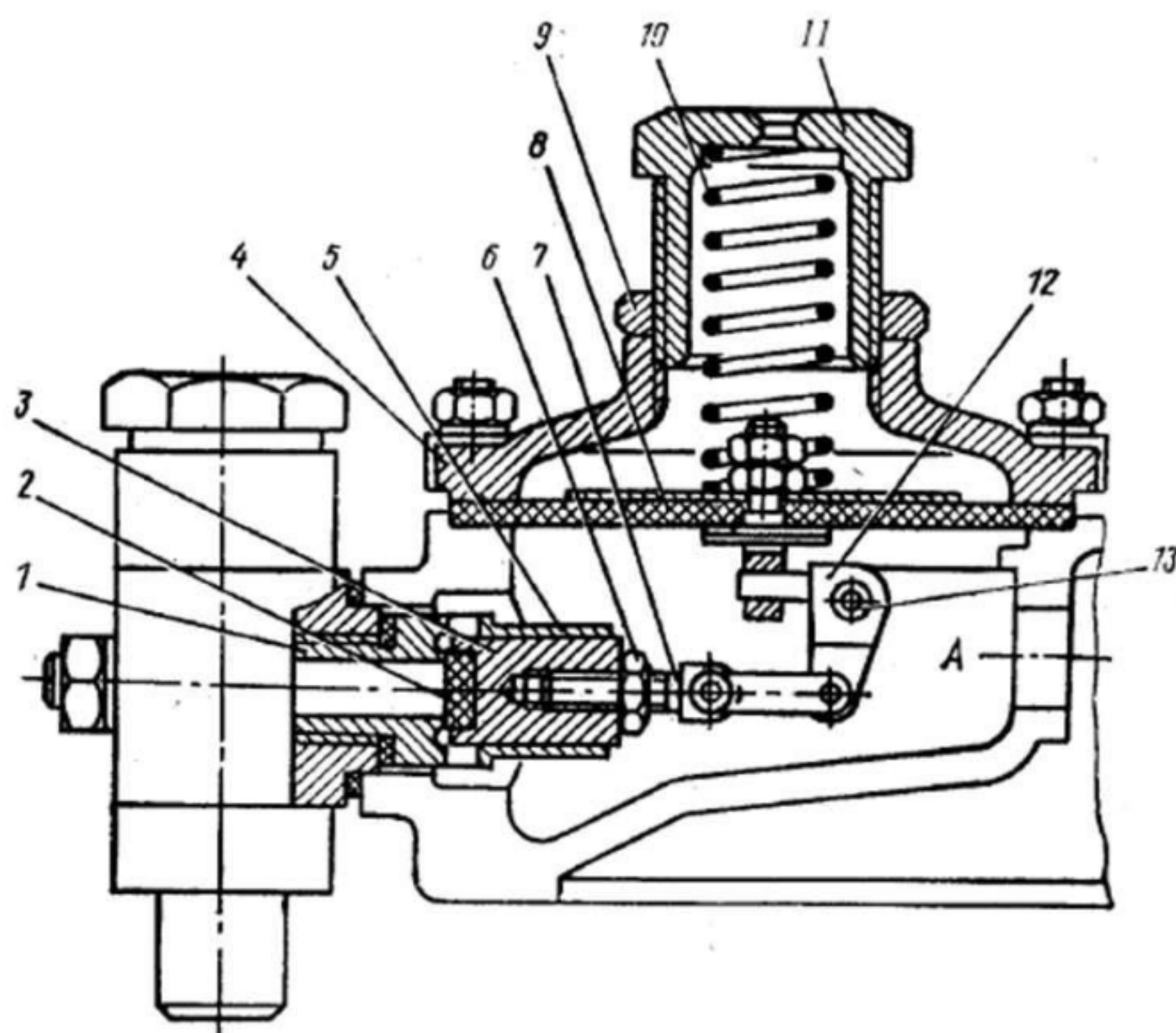
Рис. 3.2. Первая ступень редуктора: А-полость первой ступени 1-седло клапана; 2- уплотнитель; 3-клапан; 4-крышка; 5-направляющая клапана; 6-контргайка; 7-винт; 8-диафрагма; 9-контргайка; 10-пружина; 11- регулировочная гайка; 12-рычаг; 13-ось.
