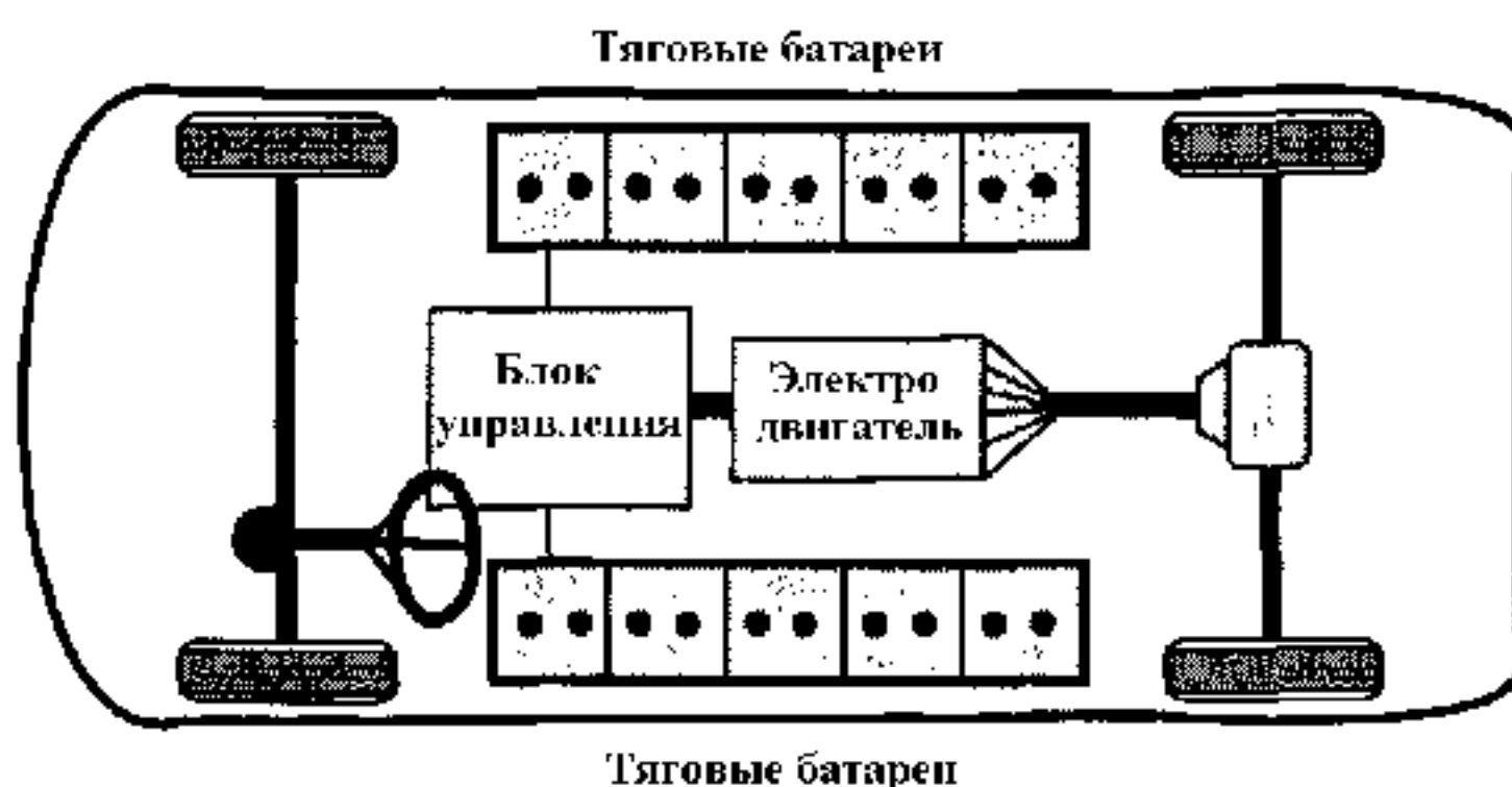
Рис. 1. Компоновочная схема электромобиля
