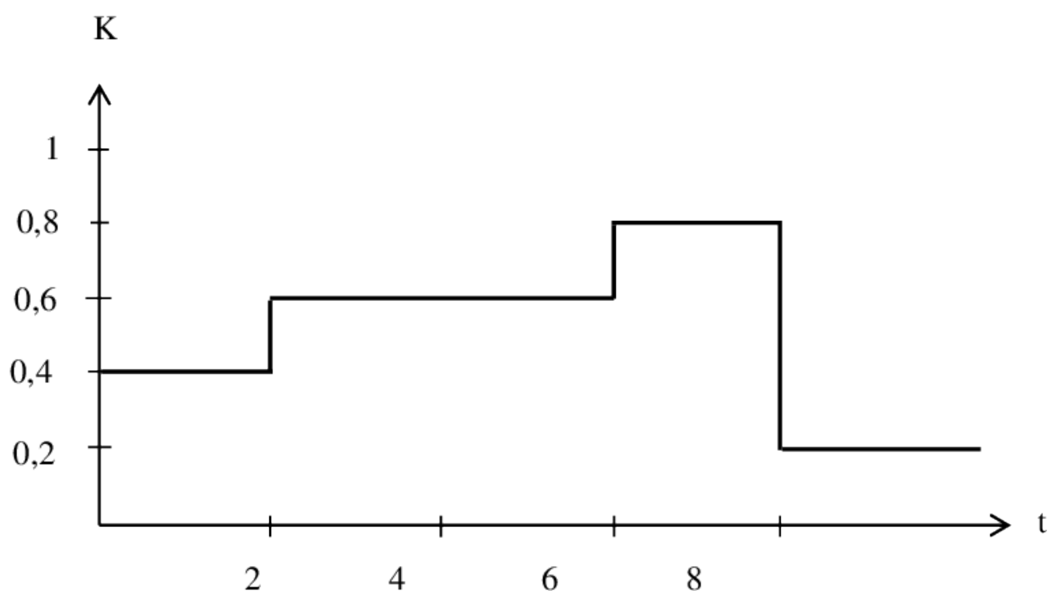
Рис. 2.1. График нагрузки трансформатора
