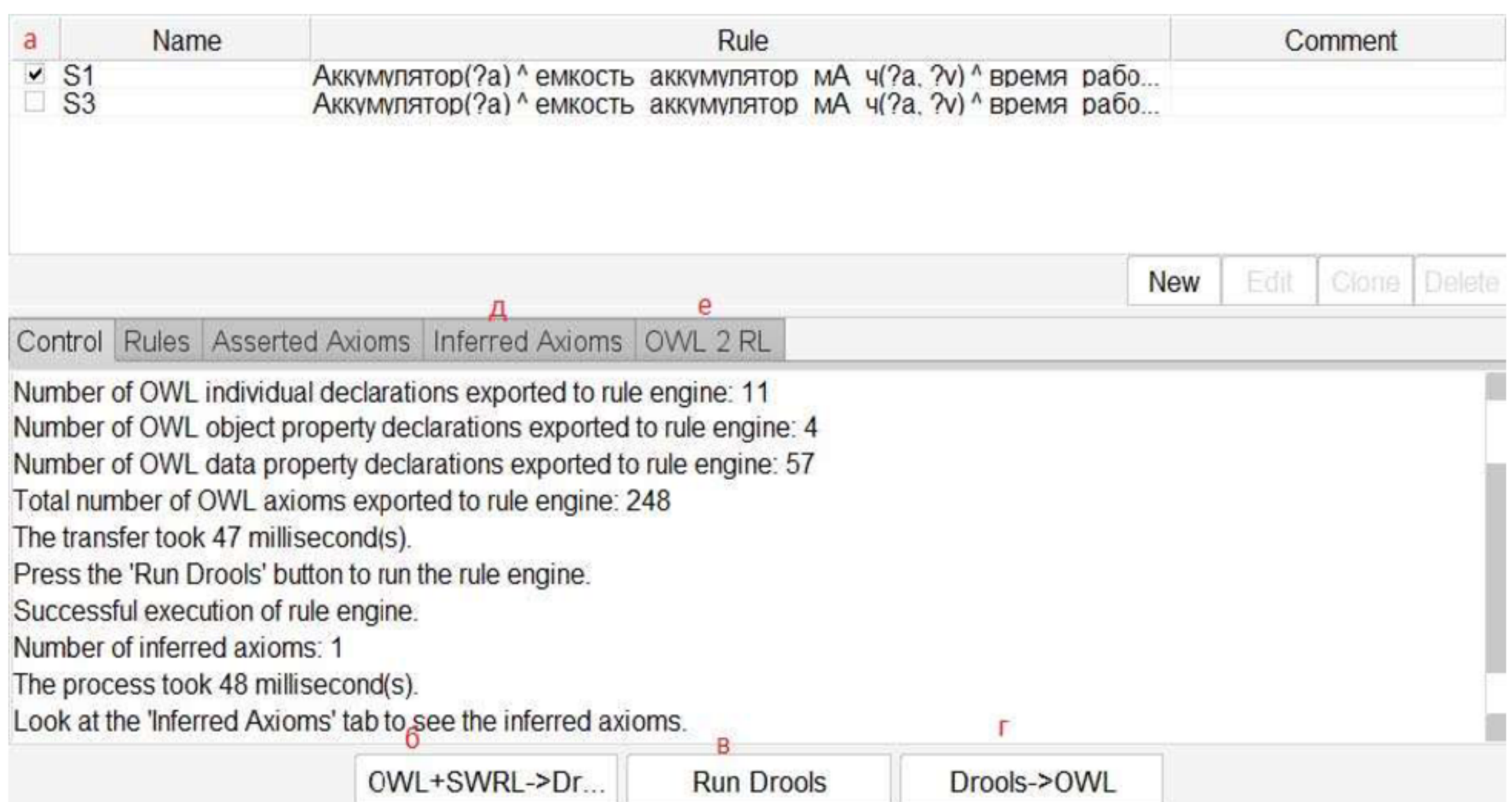
Рис. 26 Вкладка SWRL в системе Protégé (а – активность правила; б – кнопка загрузки правил; в – запуск вывода на основе правил; г – внесение выведенных понятий в онтологию; д – список правил; е – список правил)
