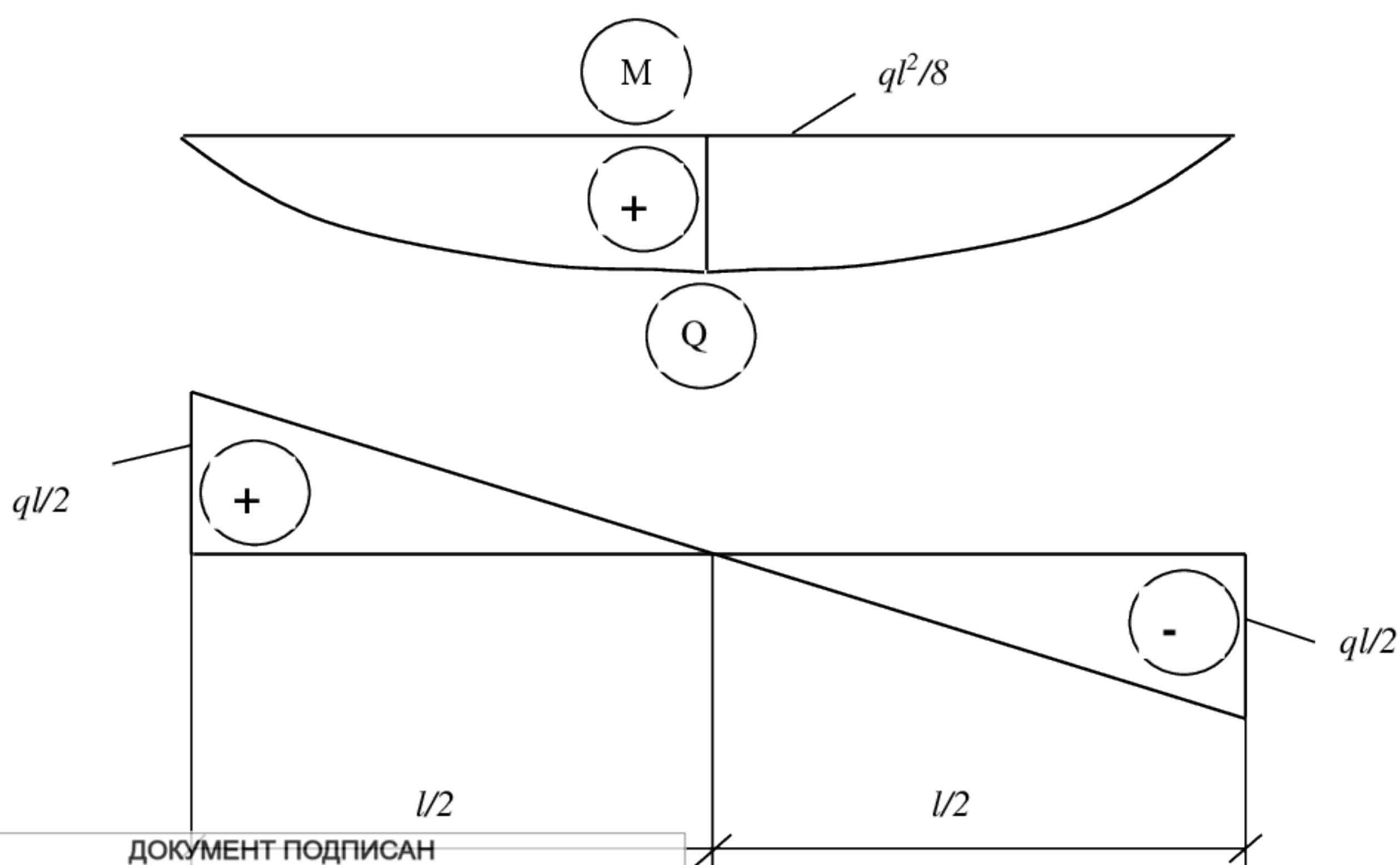
Рисунок 3 – Расчетная схема плиты и эпюры расчетных усилий (изгибающих моментов M и поперечных сил Q )
