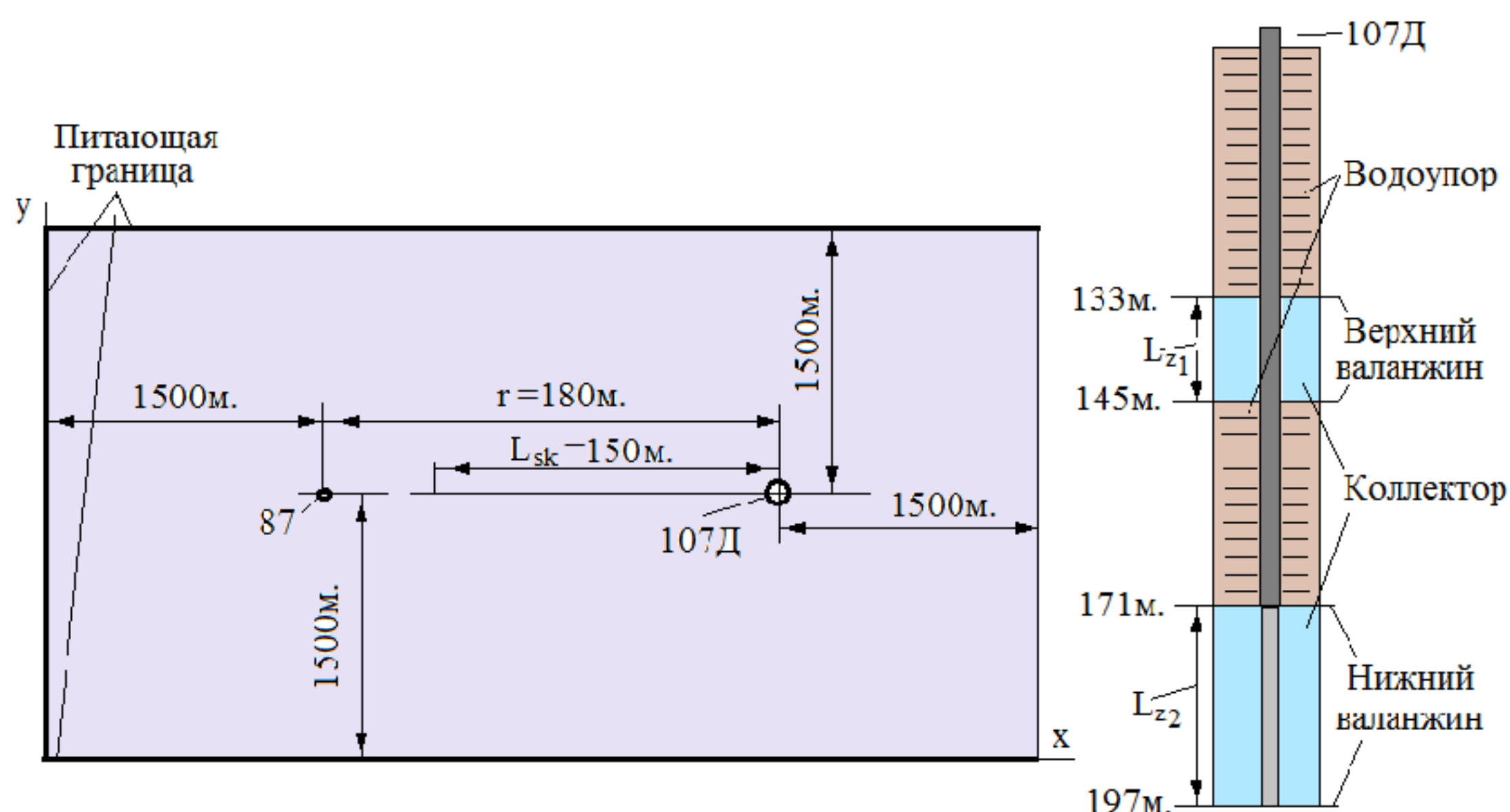
Рис. 4.1. Схема расположения скважин
