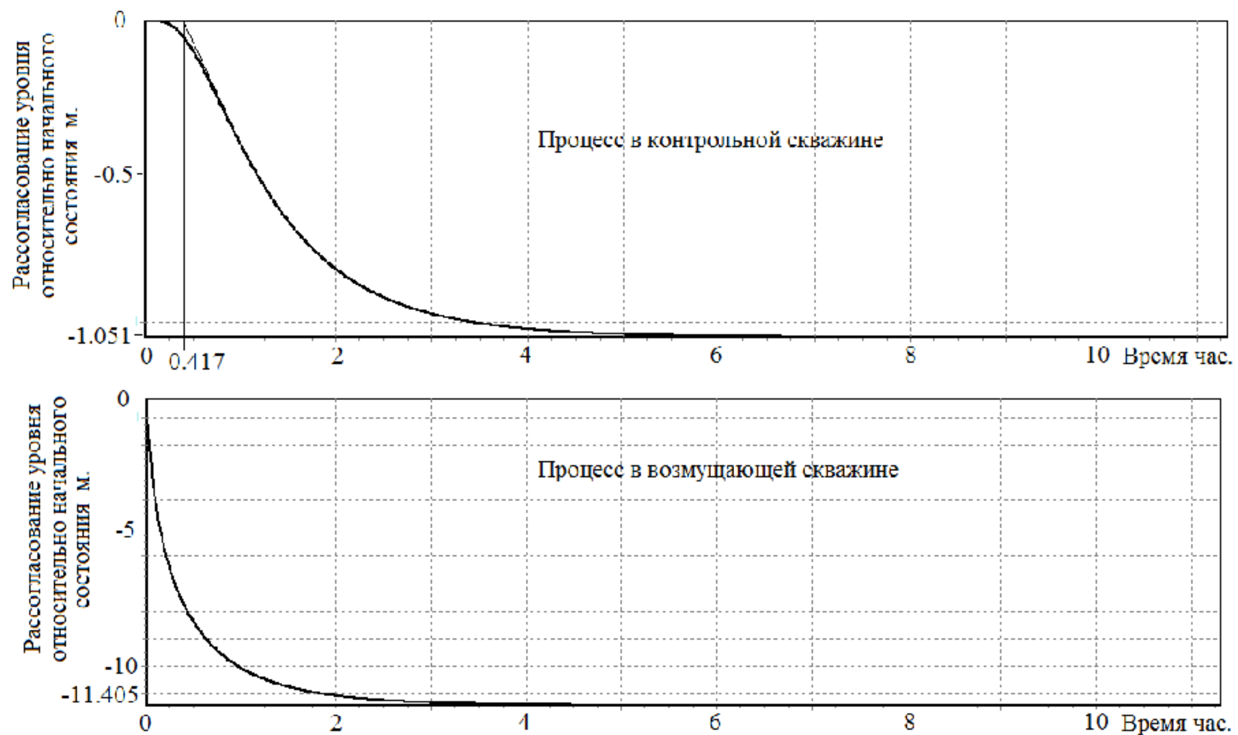
Рис.4.2. Переходные процессы в скорректированной модели
