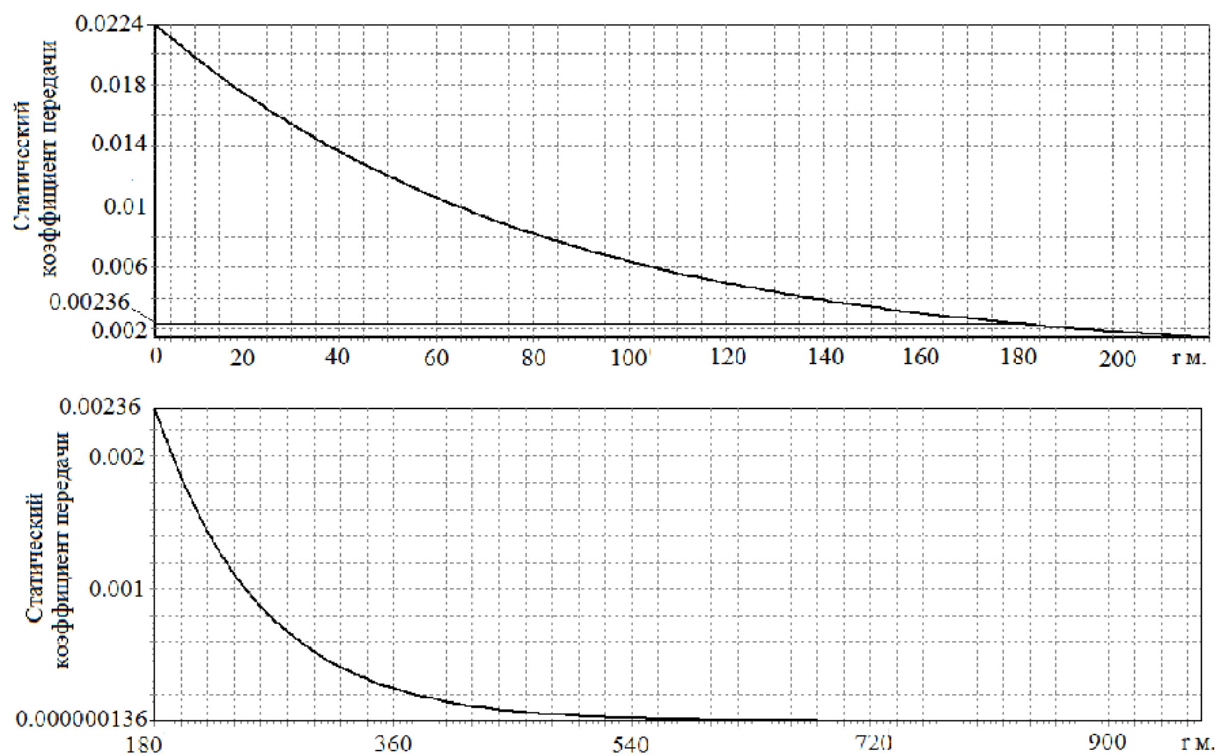
Рис.3.1. График коэффициента гидравлического взаимодействия скважин
