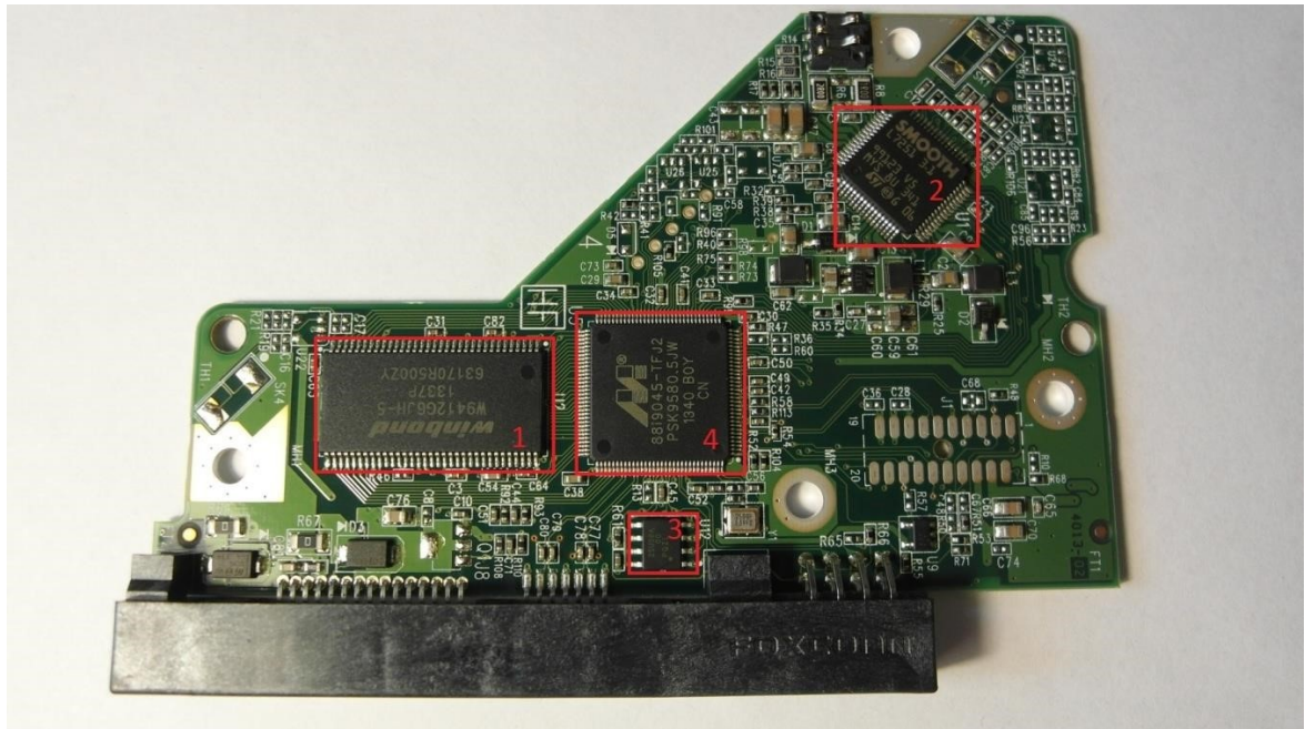
Рис. 1. Плата жесткого диска
