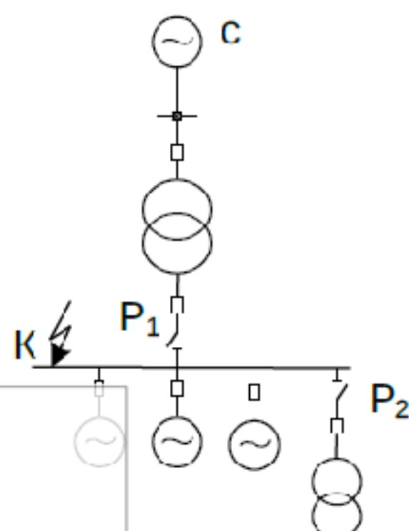
Рисунок 7 – Расчетная схема
