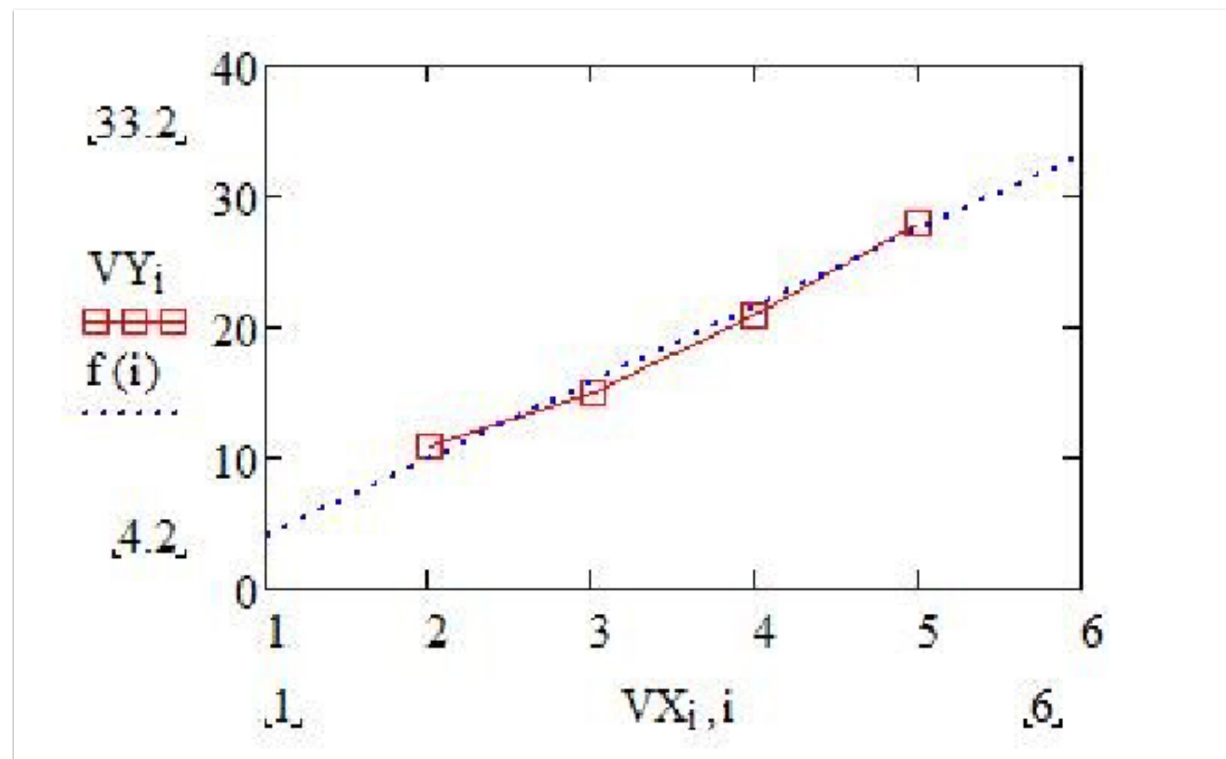
Рисунок 4.2 -Линейная регрессия
