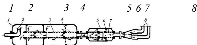
Рис. 1. Схема глушителя отработавших газов:
