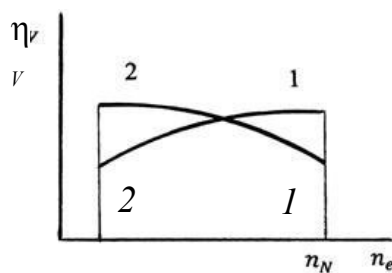
Рис. 2. График изменения коэффициента наполнения \eta при быстроходной и тихоходной регулировке фаз газораспределения: — частота вращения
