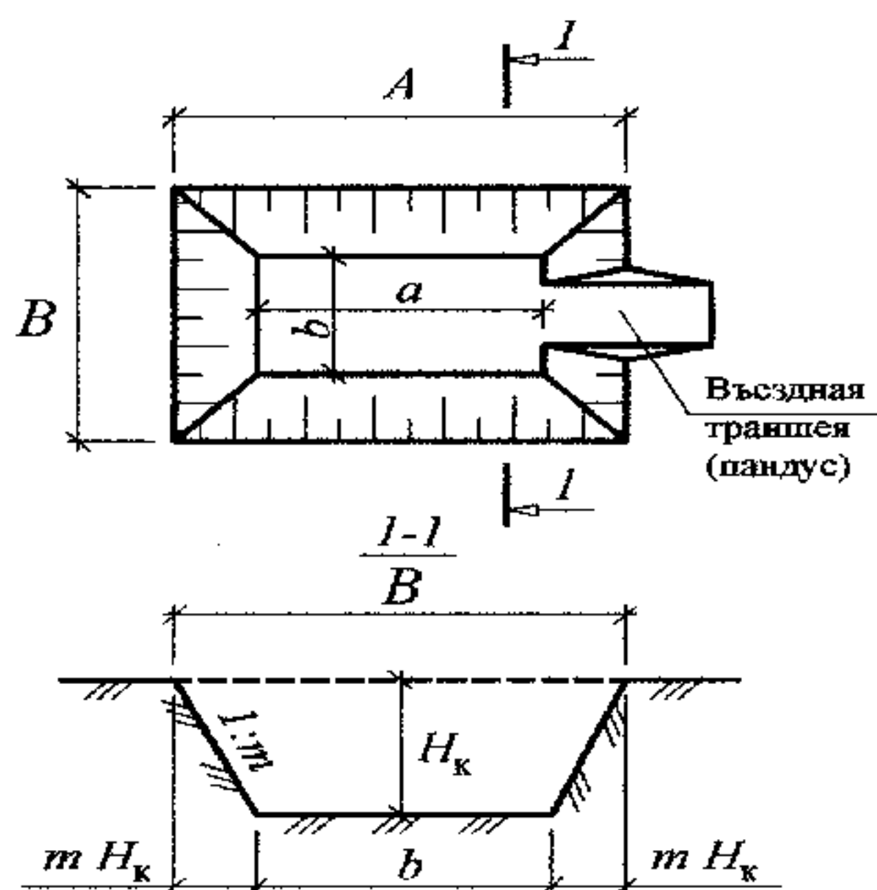
Рис. 5. Схема котлована
