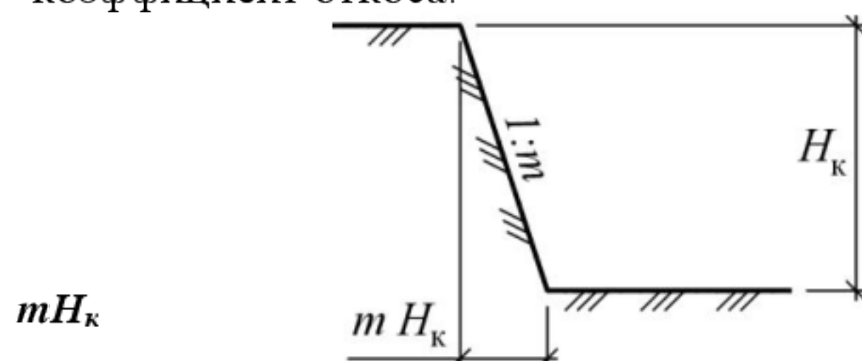
Рис. 3. Схема откоса
