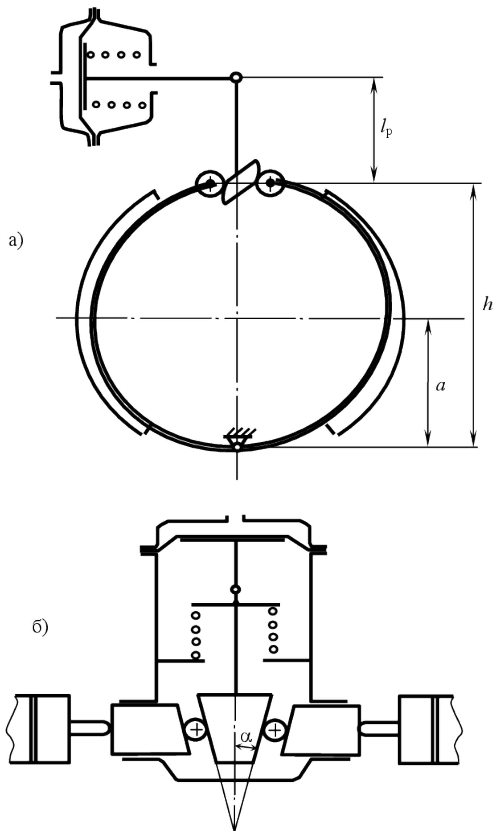
Рисунок 2.1 - Схемы тормозных механизмов: а – кулачковый; б - клиновым.
