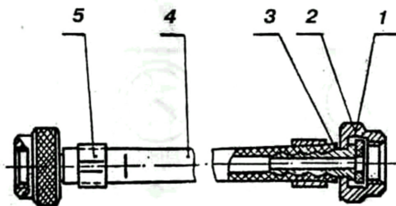
Рисунок 2.4 – Шланг: 1. Гайка. 2. Прокладка. 3. Ниппель. 4. Рукав. 5. Трубка.
