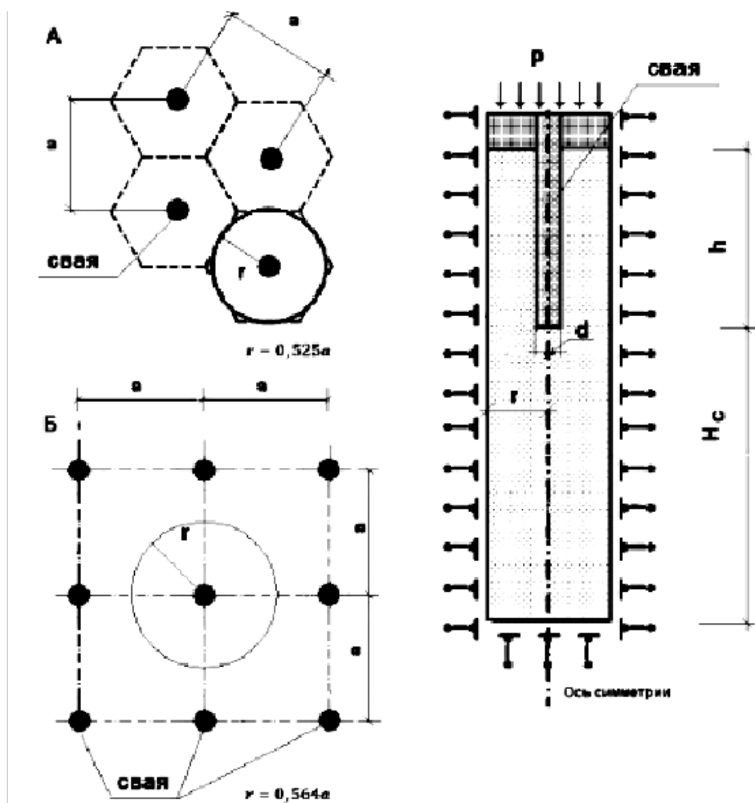
Рис. 3.16. Расчетная схема метода ячейки
