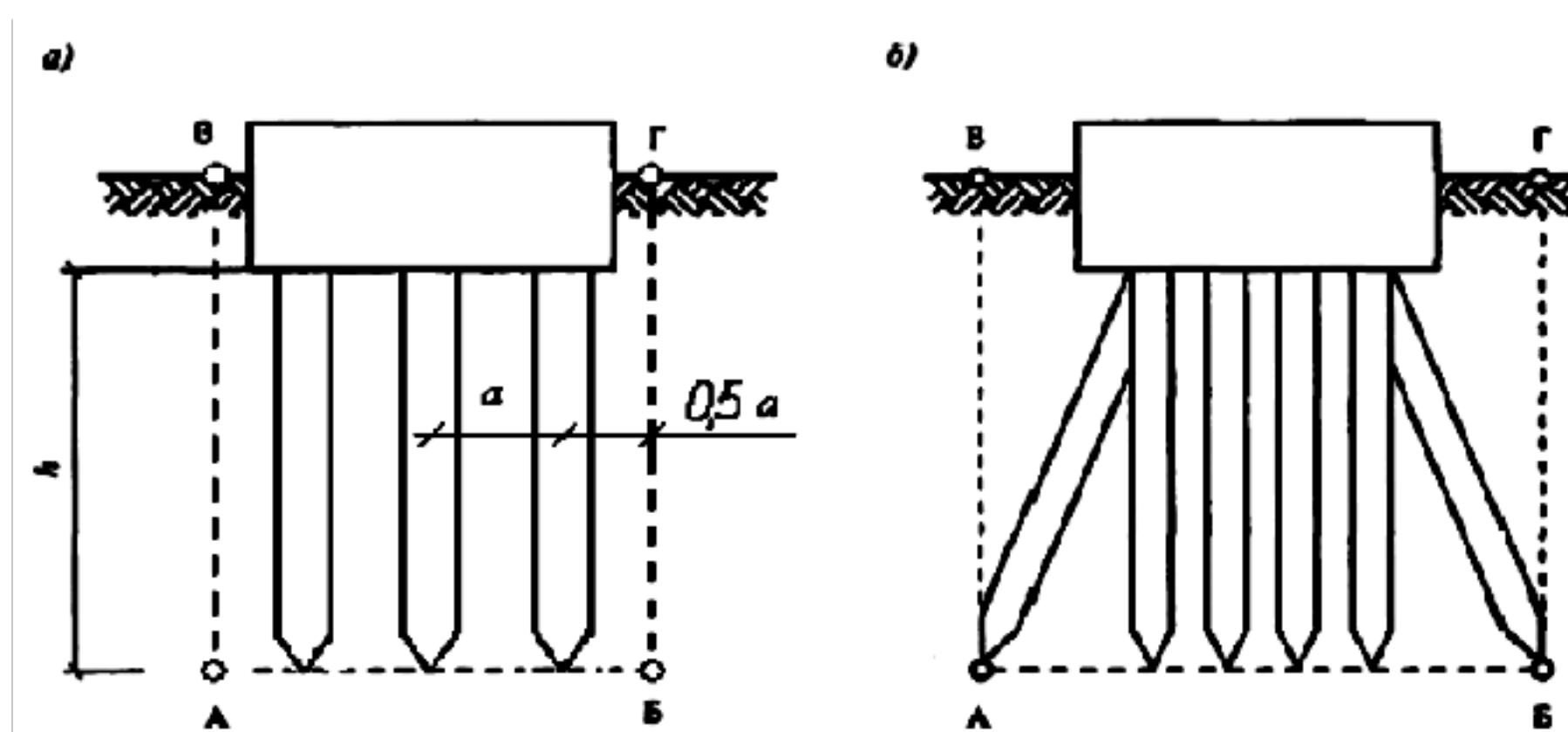
Рис. 3.15. Определение границ условного фундамента при расчете осадки свайных фундаментов
