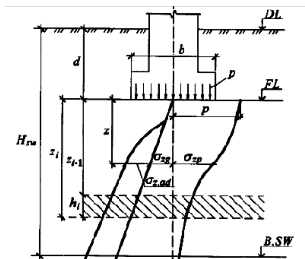
Рис. 3.5. Состояние напряжений в основании при набухании грунта
