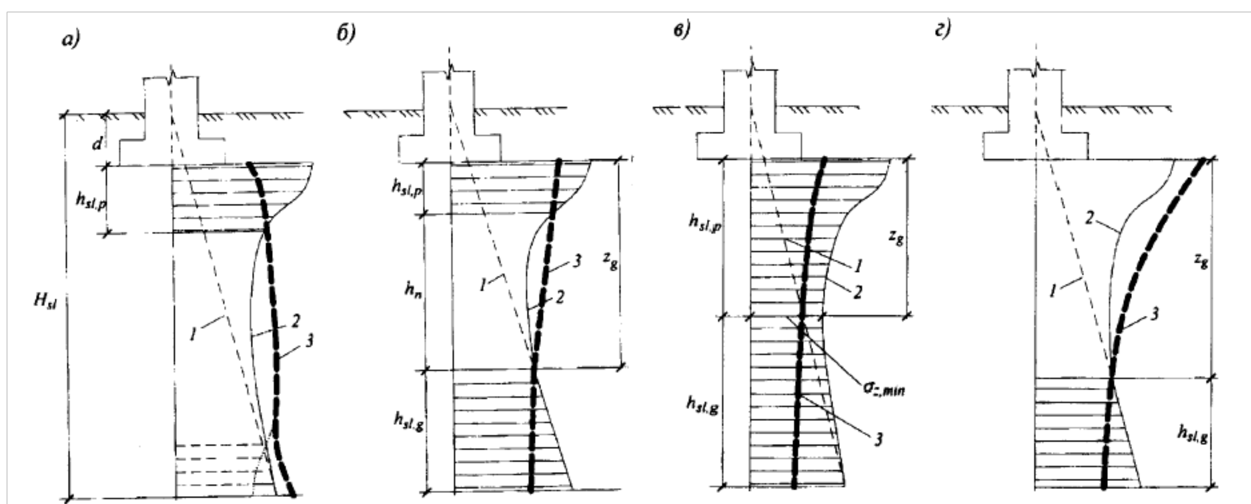
Рис. 3.4. Схемы к расчету просадок основания фундаментов: а - просадка от собственного веса \sigma_{sl,g} отсутствует (не превышает 5 см), возможна только просадка от внешней нагрузки \sigma_{sl,p} в верхней зоне просадки h_{sl,p} (I тип грунтовых условий); б, в, г - возможна просадка от собственного веса \sigma_{sl,g} в нижней зоне просадки h_{sl,g} начиная с глубины z_g (II тип грунтовых условий); б - верхняя и нижняя зоны просадки не сливаются, имеется нейтральная зона h_n ; в - верхняя и нижняя зоны просадки сливаются; г - просадка от внешней нагрузки отсутствует; 1 - вертикальные напряжения от собственного веса грунта \bar{\sigma}_{zg} ; 2 - суммарные вертикальные напряжения от внешней нагрузки и собственного веса грунта \bar{\sigma}_z = \bar{\sigma}_{zp} + \bar{\sigma}_{zg} ; 3 - изменение с глубиной начального просадочного давления p_{sl} ; H_{sl} - толщина слоя просадочных грунтов (просадочная толща); d - глубина заложения фундамента
