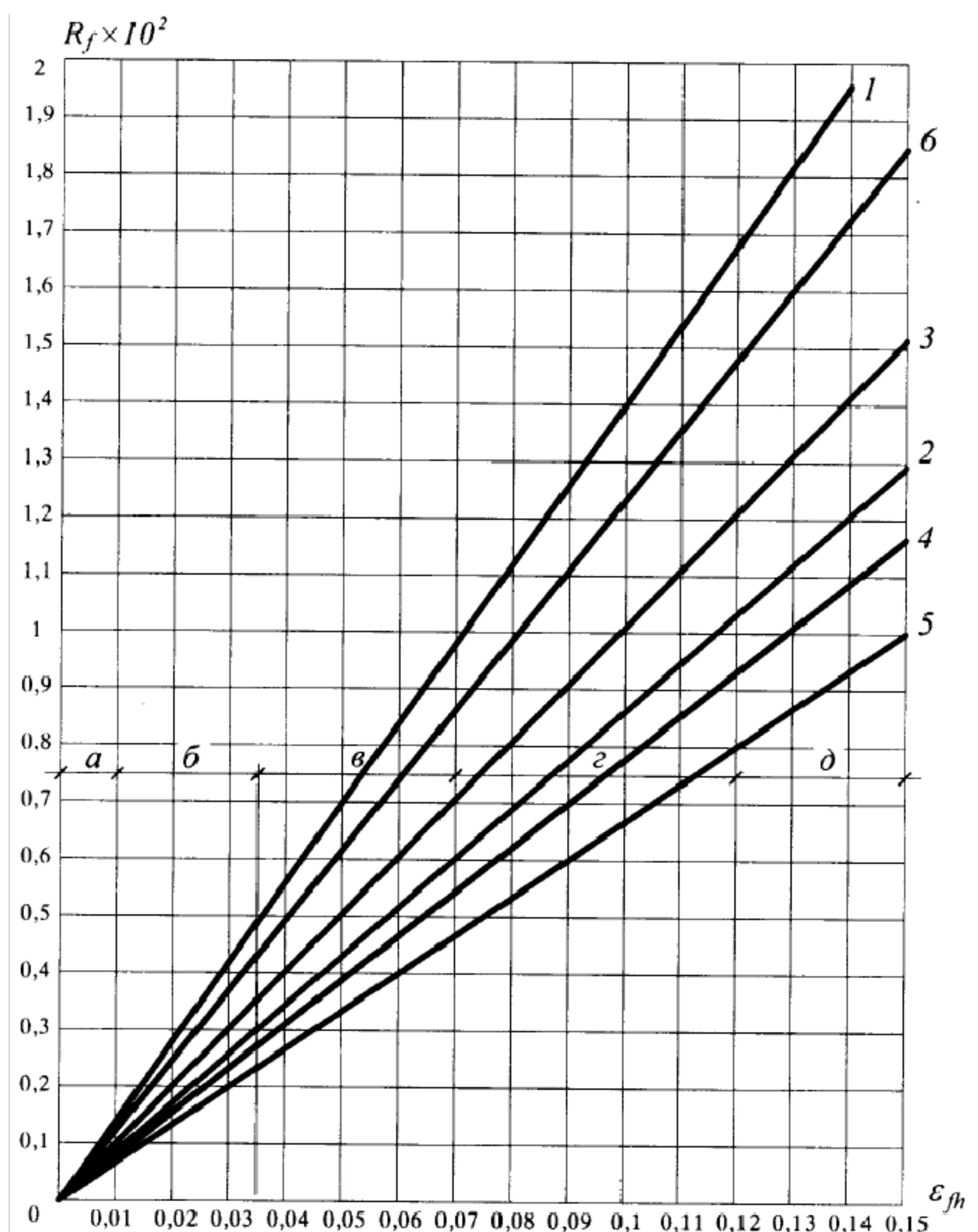
Рис. 3.11. Взаимосвязь параметра R_f и относительной деформации пучения \epsilon_{fh} 1, 2 - супеси; 3 - суглинки; 4 - суглинки с 0,07 < I_p \leq 0,13 ; 5 - суглинки с 0,13 < I_p \leq 0,17 ; 6 - глины (в грунтах 2, 4 и 5 содержание пылеватых частиц размером 0,05-0,005 мм составляет более 50 % по массе); а - практически непучинистый; б - слабопучинистый; в - среднепучинистый; г - сильнопучинистый; д - чрезмернопучинистый
