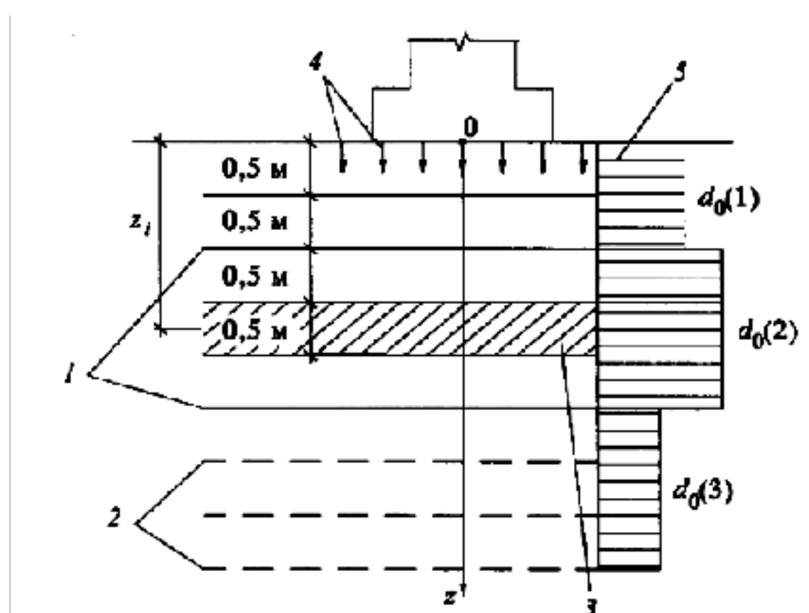
Рис. 3.7. Схема для расчета рассоления основания при вертикальной фильтрации 1 - границы слоев с различным содержанием гипса; 2 - границы расчетных слоев; 3 - расчетный слой; 4 - направление фильтрации; 5 - начальная эпюра относительного содержания гипса d_0(z)
