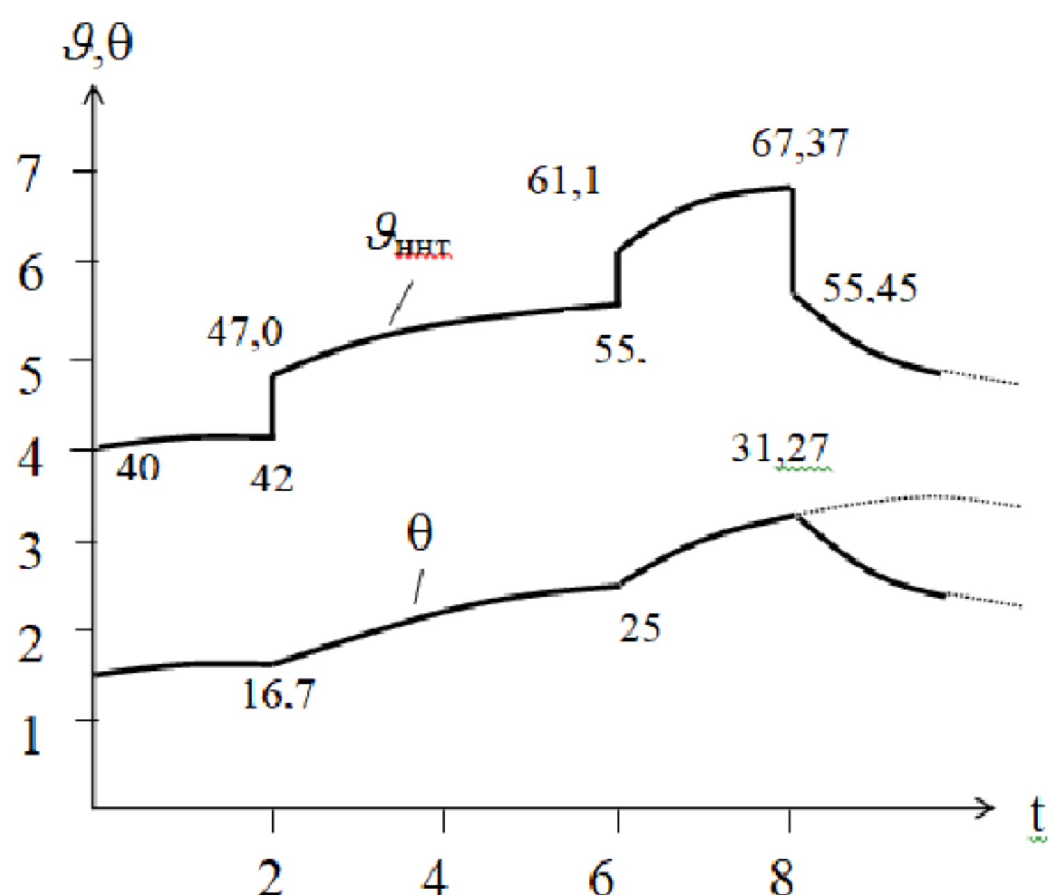
Рисунок 2.2 - Изменение температуры наиболее нагретой точки обмотки трансформатора
