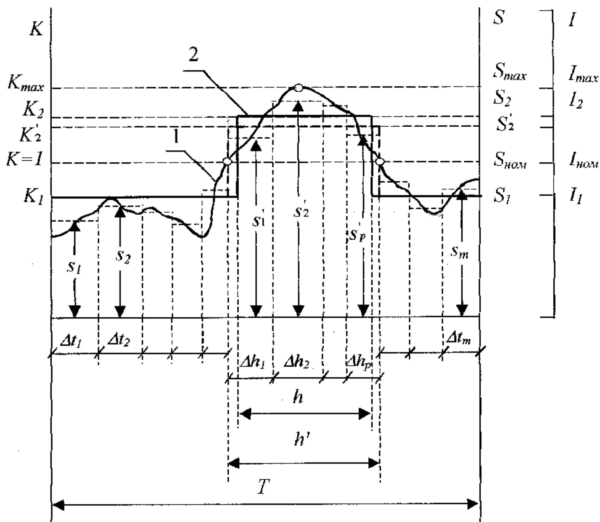
1 – заданный график нагрузки; 2 – двухступенчатый прямоугольный график нагрузки
