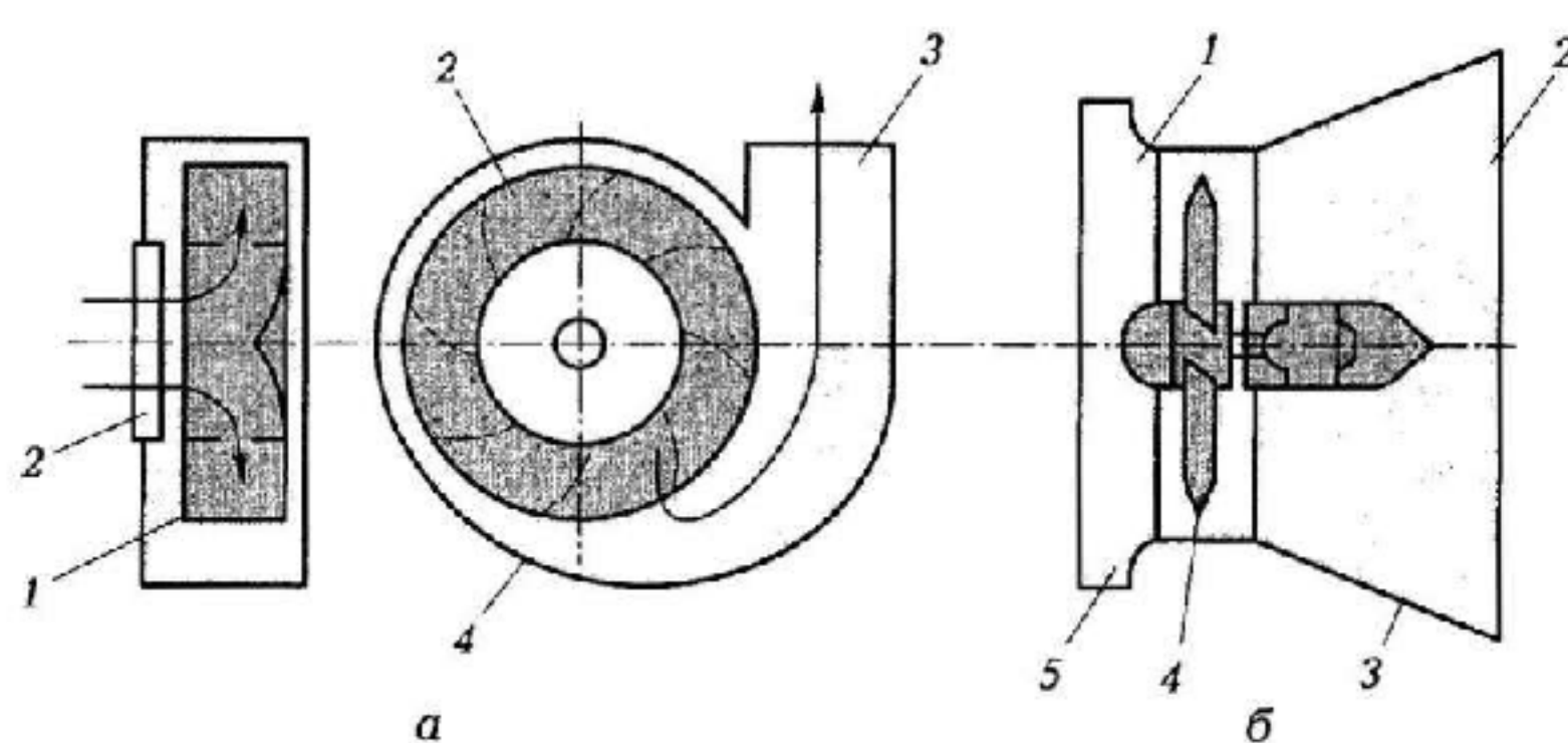
Рис. 3.4. Схемы вентиляторов:
