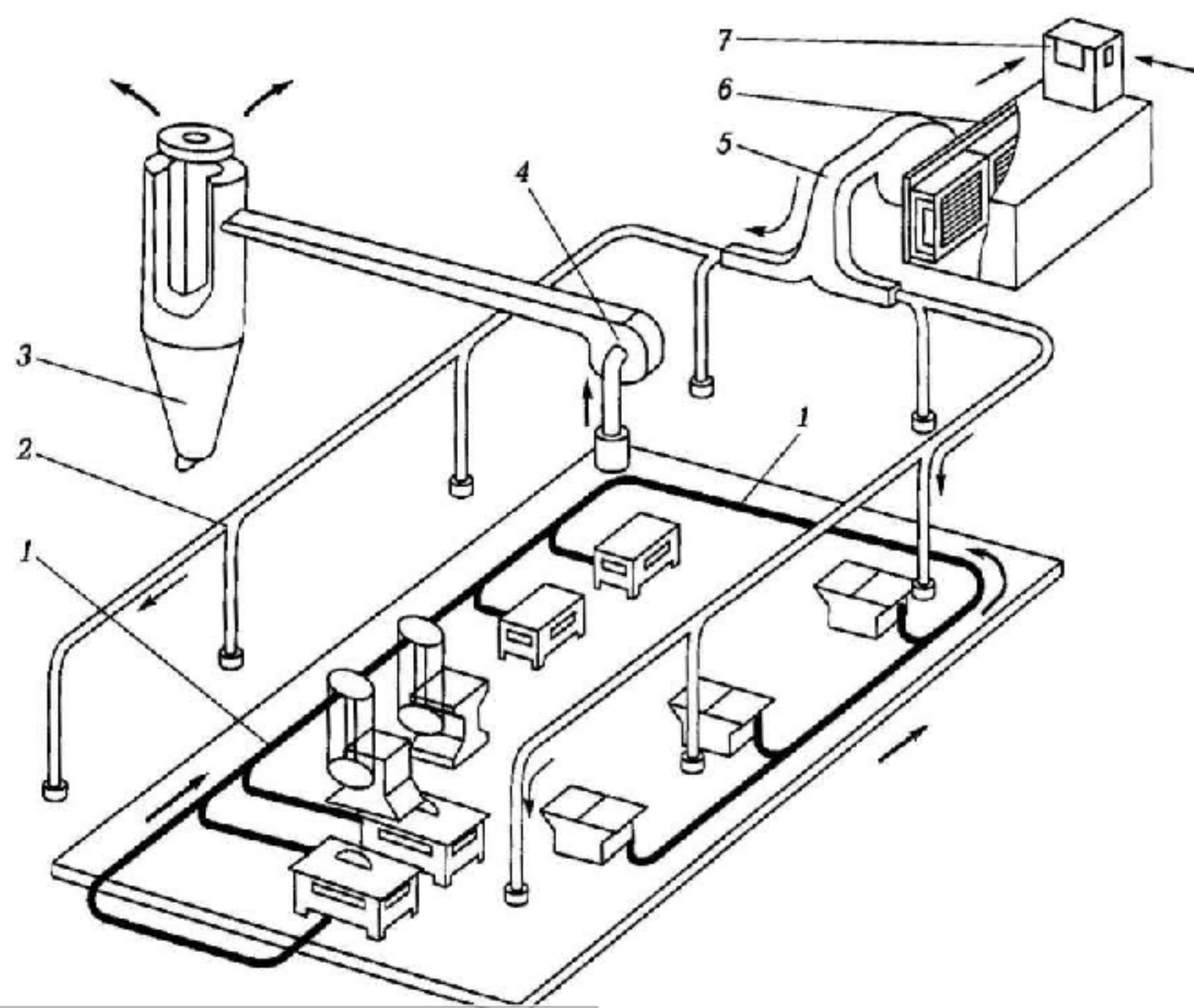
Рис. 3.3. Местная вытяжная вентиляция.
