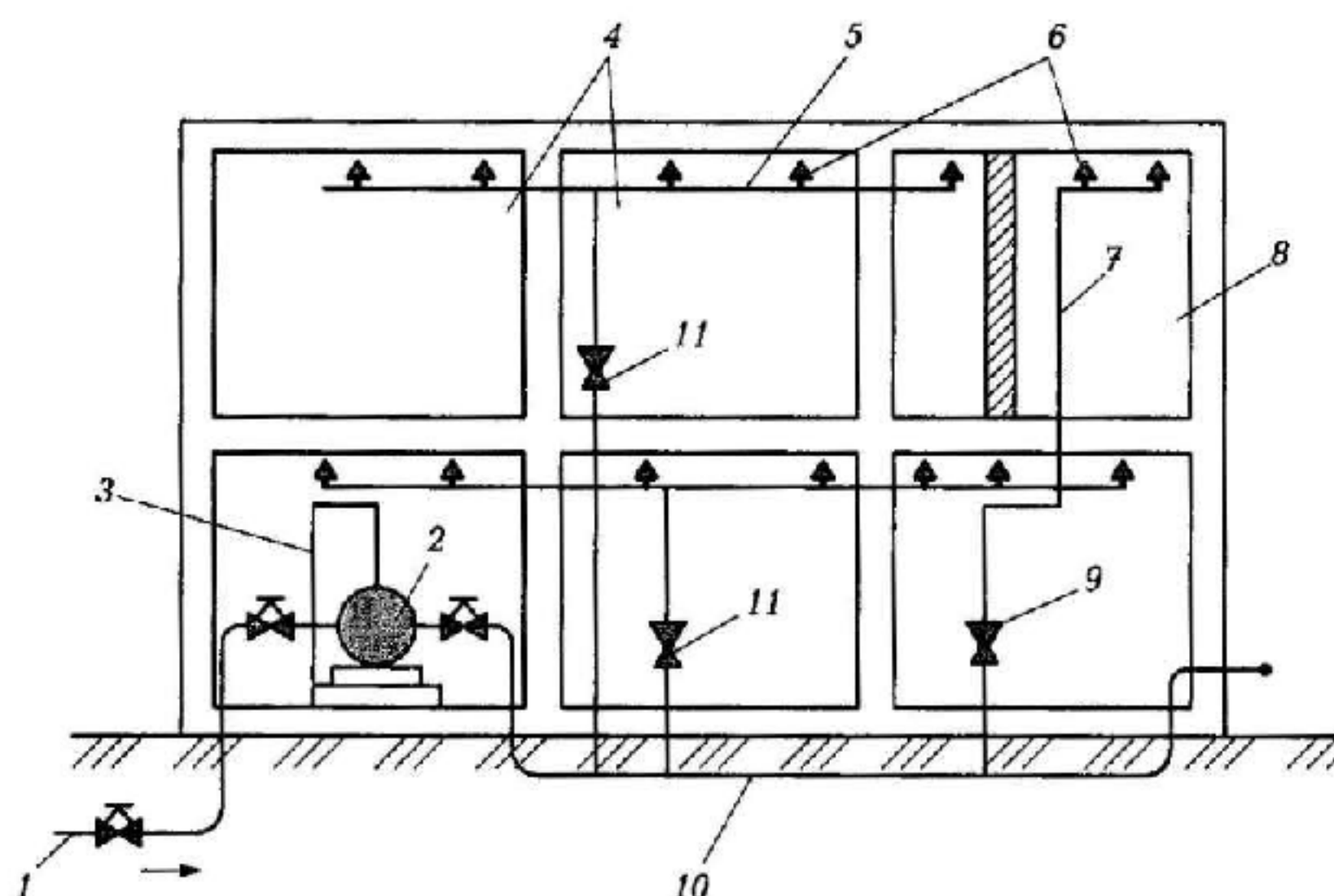
Рис. 9.1. Принципиальная схема стационарной спринклерной установки:
