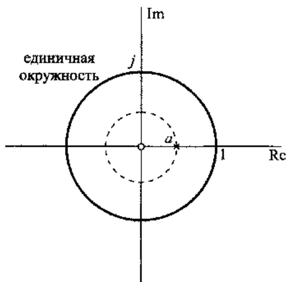
Рисунок 3. Схема нулей и полюсов в ОС.
