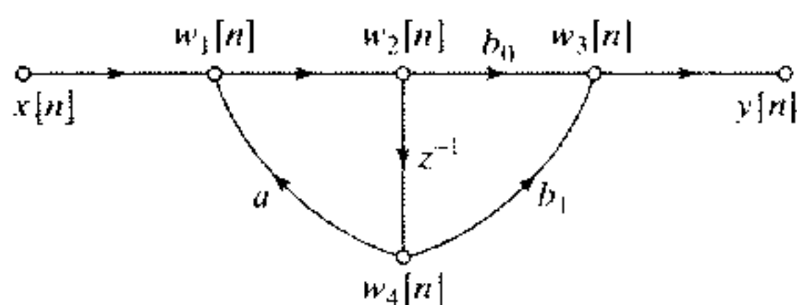
рис.4 Потоковый граф
