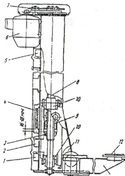
Рис. 7. Левая стойка двухстоечного подъемника с электро механическим приводом: 1 - аварийный выключатель; 2, 5 - концевые выключатели; 3 - страхующая гайка; 4 - электроклемник; 6 - электродвигатель; 7 - цепная передача; 8 - рабочий винт; 9 - грузовая гайка; 10 - опора винта; 11 - каретка; 12 - подхват; 13 - поворотная балка
