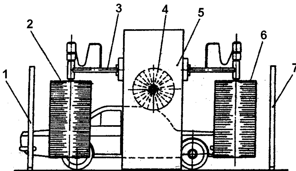
Рисунок 2.7 Схема portalной щёточной установки, модель М – 130.
