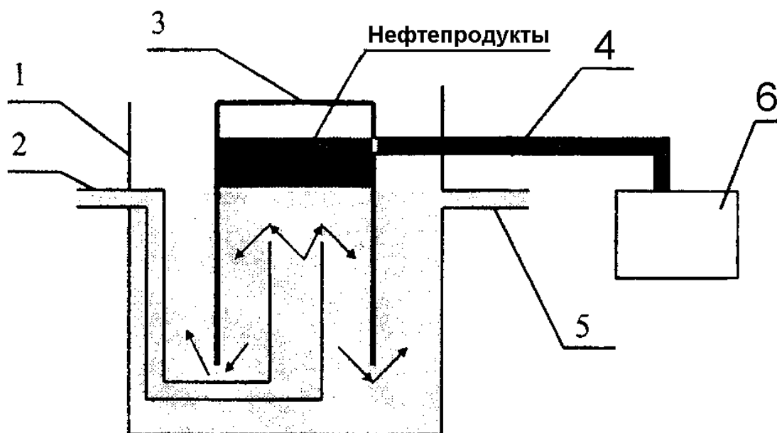
Рисунок 3.2 Схема маслобензоуловителя.
