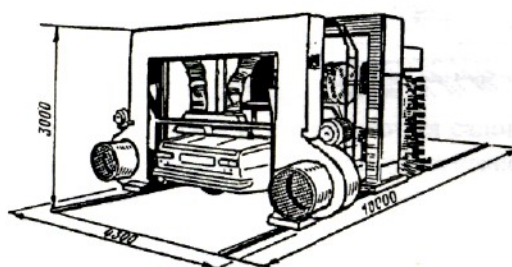
Рис. 12. Моечная установка GM-100, сушикой GS-100, с раздвижными воздушными коллекторами
