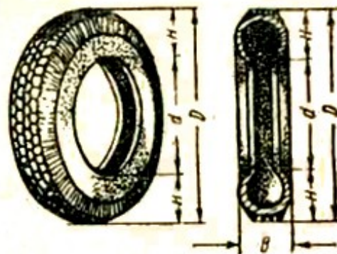
Рис. 2. Обозначение размеров
