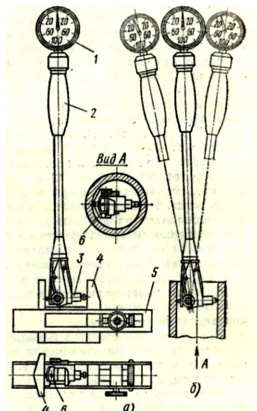
Рис. 8. Индикаторный нутромер:
