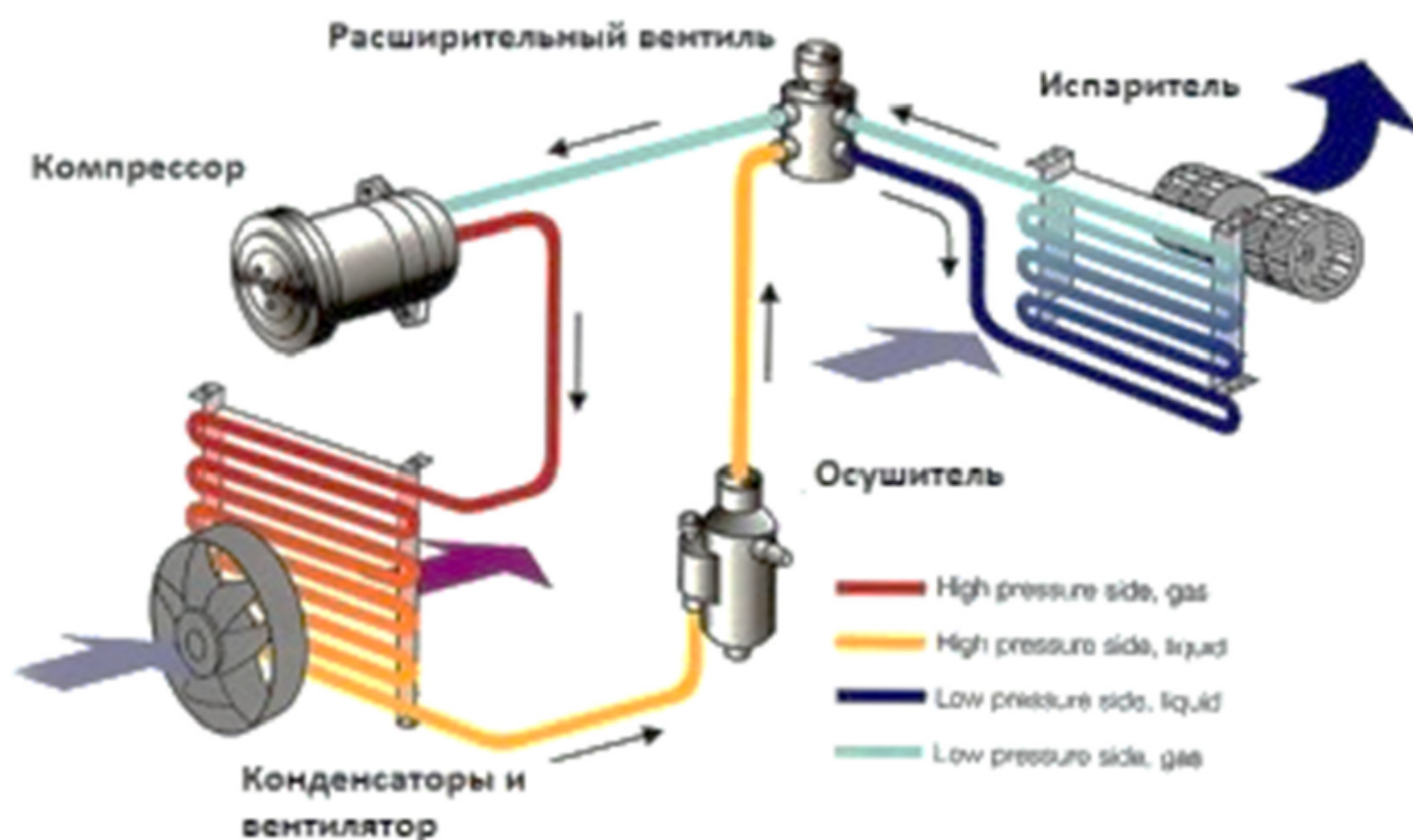
Рис. 3. Система кондиционирования.
