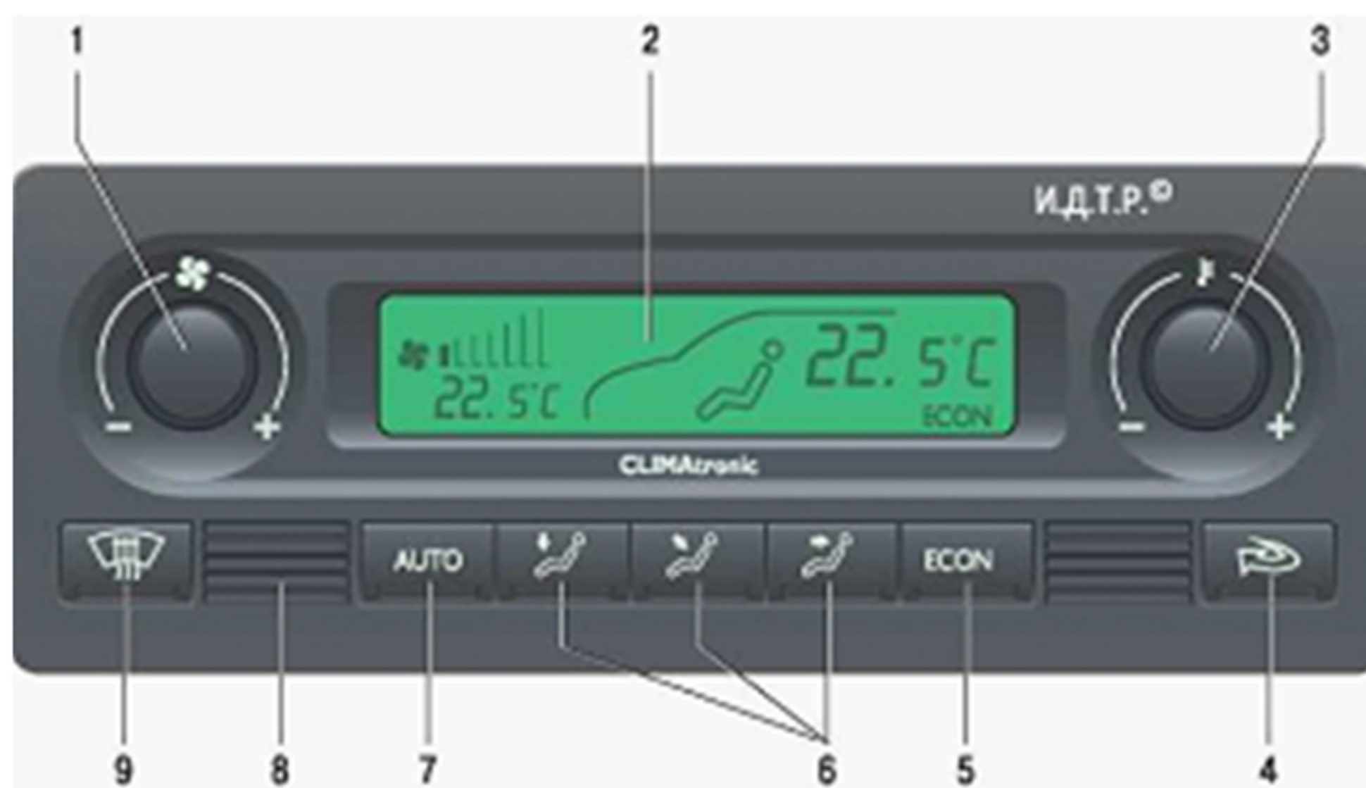
Рис. 5. Блок автоматического управления системой отопления(кондиционирования) и вентиляции салона: 1 - переключатель режимов работы электровентилятора воздухонагнетателя; 2 - дисплей; 3 - регулятор температуры поступающего в салон воздуха; 4 - выключатель кондиционера; 5 - выключатель рециркуляции; 6 - переключатели распределения потоков воздуха; 7 - выключатель автоматического режима
