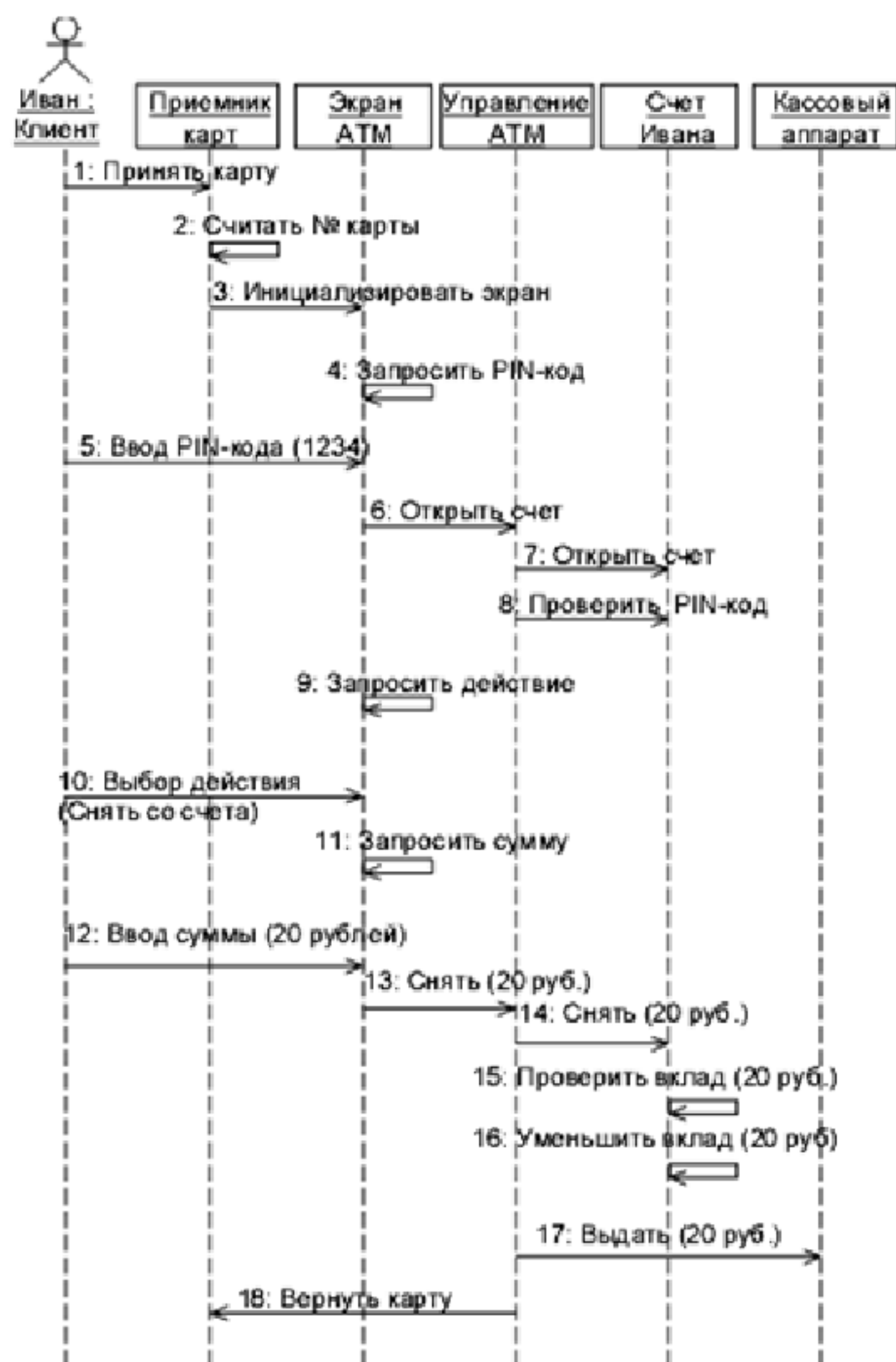
Рисунок 2.7 - Пример диаграммы последовательности
