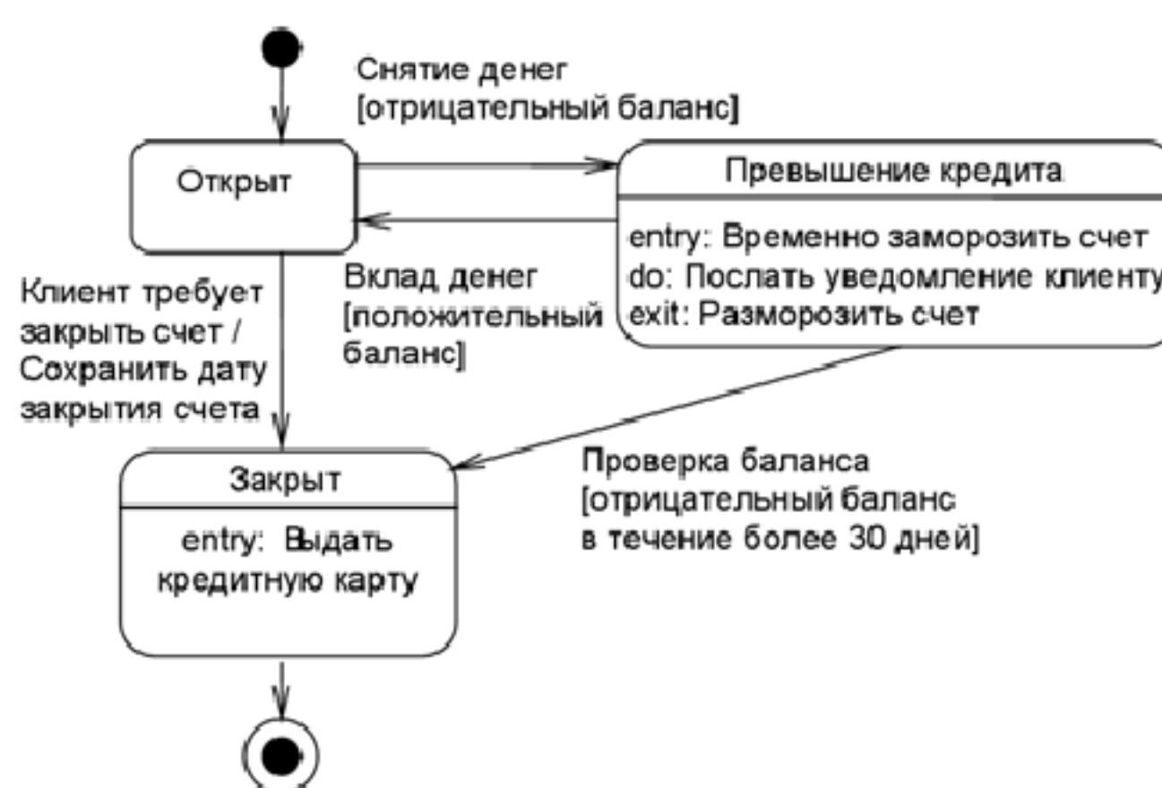
Рисунок 2.18 - Пример диаграммы состояний
