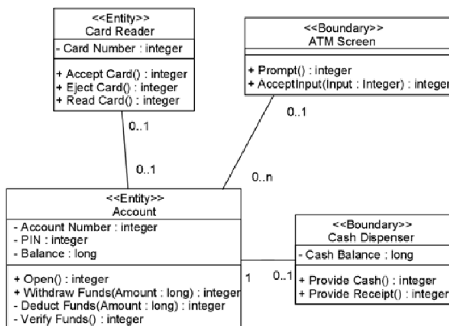
Рисунок 2.9 - Пример диаграммы классов
