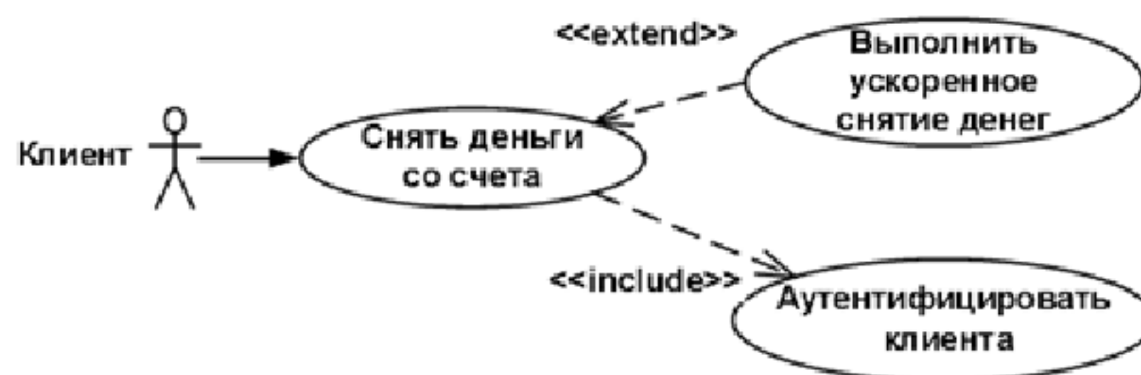
Рисунок 2.5 - Пример связи включения и расширения
