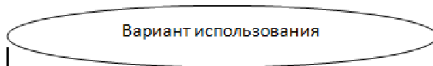
Рисунок 2.2 - Вариант использования
