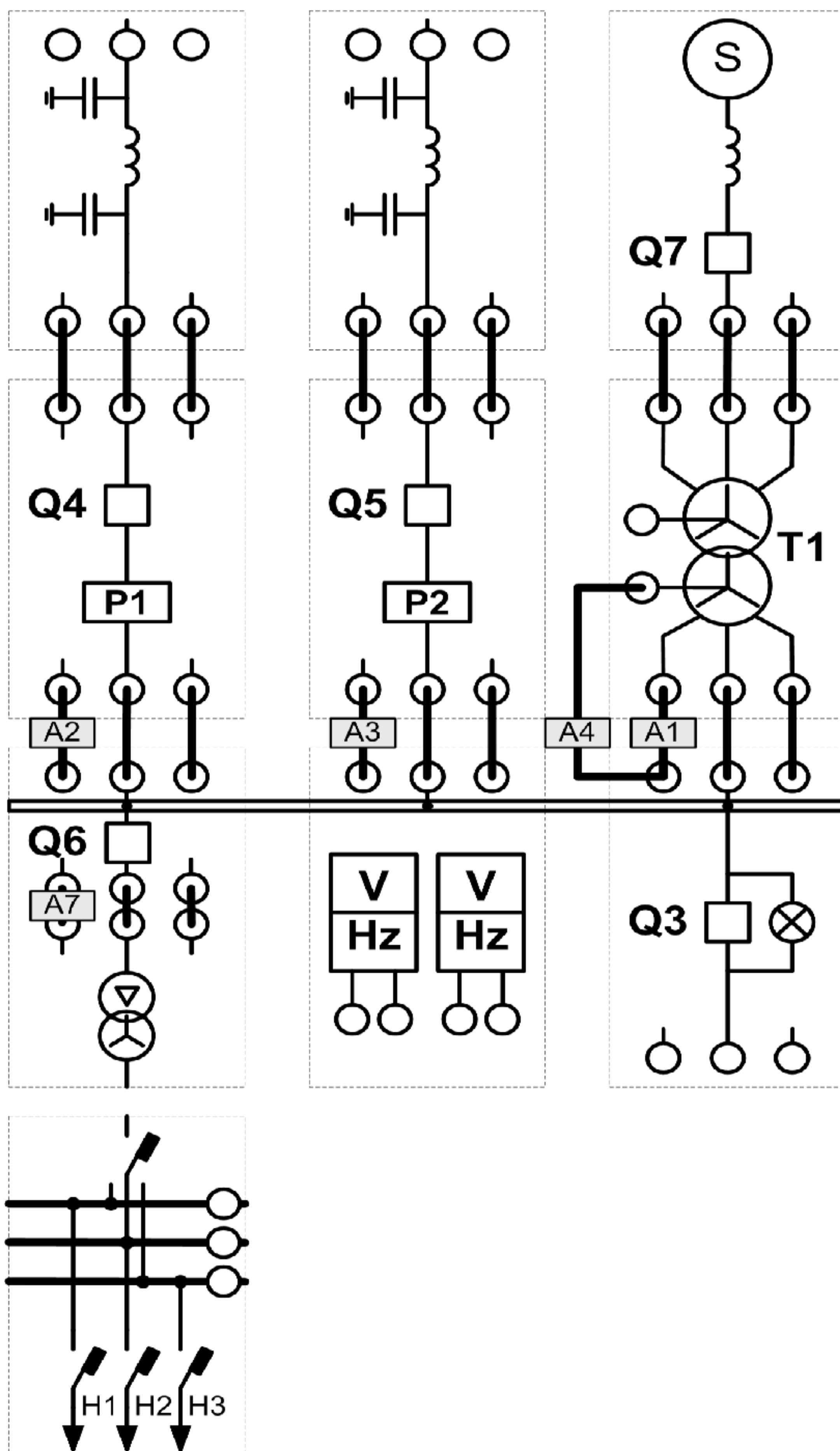
Рисунок 1. Принципиальная схема «Балансирующий узел нагрузкой»
