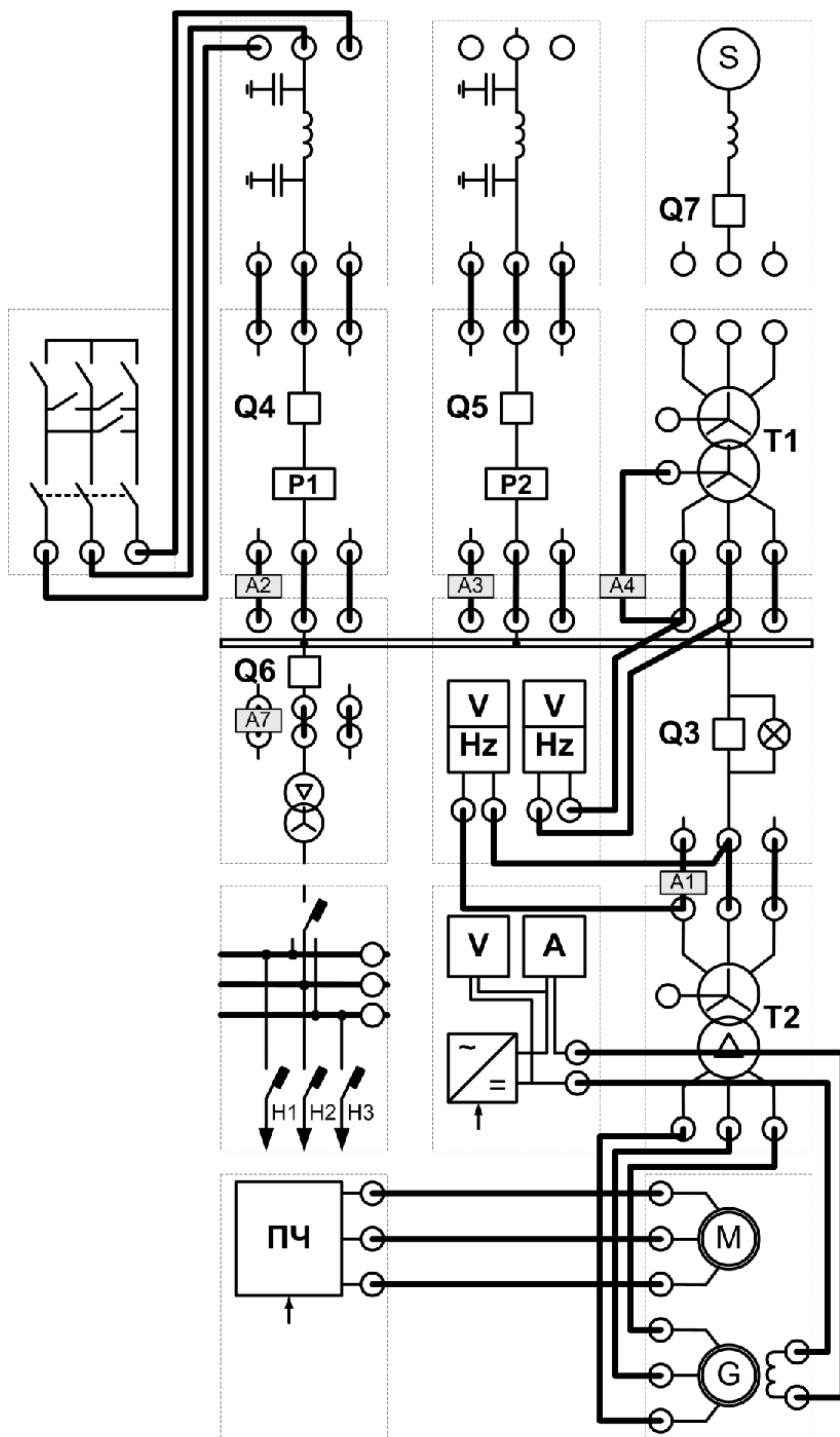
Рисунок 6.1. Электронная схема «Узел с генерацией мощности и нагрузкой»
