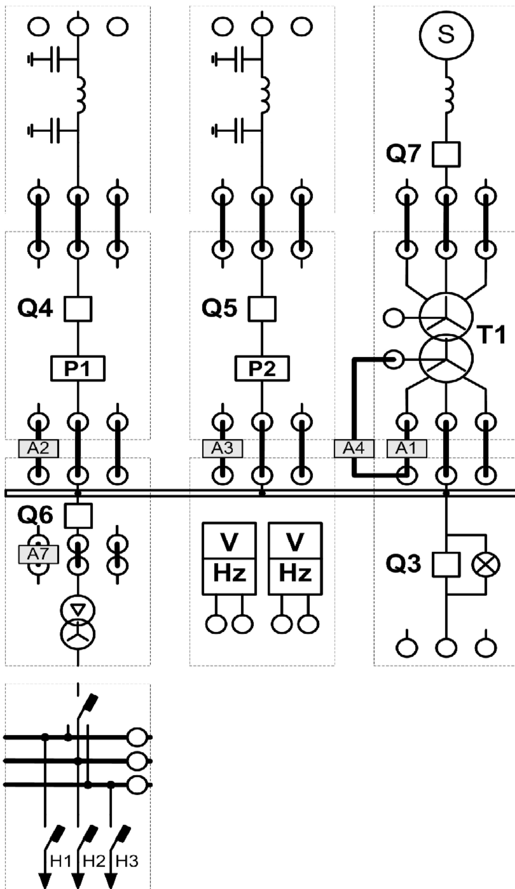
Рисунок 1. Специальная схема «Балансирующий узел нагрузкой»
