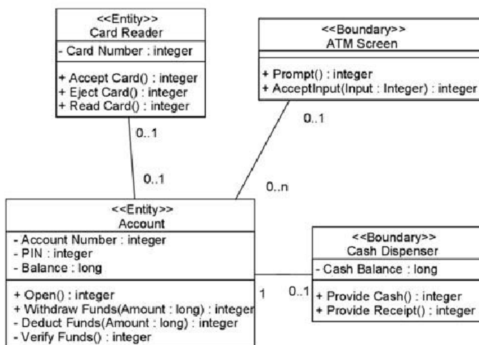
Рисунок 3.9 - Пример диаграммы
