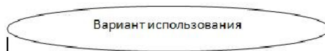
Рисунок 3.2 - Вариант использования
